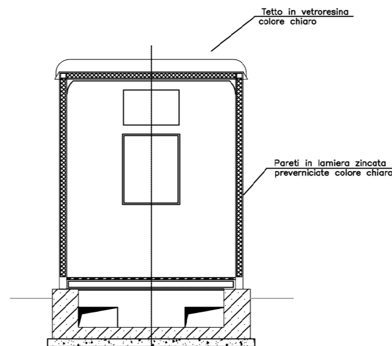
SEZIONE C-C
