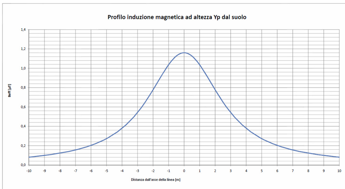
Figura 1: Profilo dell'induzione magnetica calcolata a Y_p=1,5 m di altezza dal suolo. Sezione cavo 400\text{ mm}^2 , corrente nominale 346,5. Si nota come le ipotesi assunte per il calcolo siano ancora conservative.
