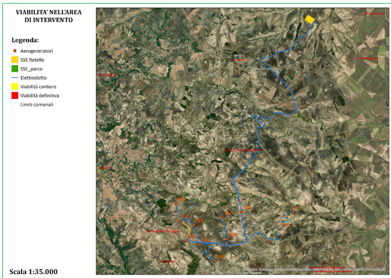
Figura 12 – Carta della viabilità: elettrodotto, v. di cantiere e v. definitiva
