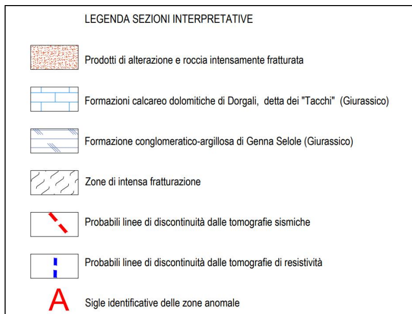
Figura 26 - Legenda interpretativa per le indagini relative alle fondazioni degli argini
