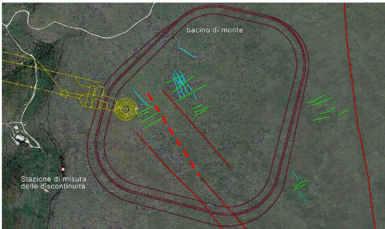
Figura 3 Sviluppo dei sistemi di discontinuità evidenti in foto aerea. L'area è quella del bacino di monte sulle dolomie giurassiche. Faglie: linee rosse. Principali famiglie di fratture presenti nell'area: linee verdi e ciano. La linea rossa tratteggiata indica il probabile andamento della faglia individuata dalle indagini ERT sotto i sedimenti colluviali.
