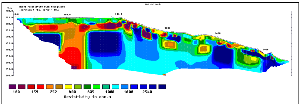
Figura 19 - Profilo geoelettrico profondo PDP-2E (Elaborazione con algoritmo robust )
