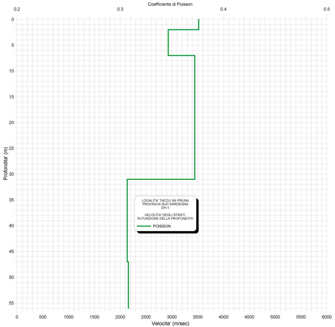
Figura 25 - Down-Hole DH-S1_Diagramma del Coefficiente di Poisson
