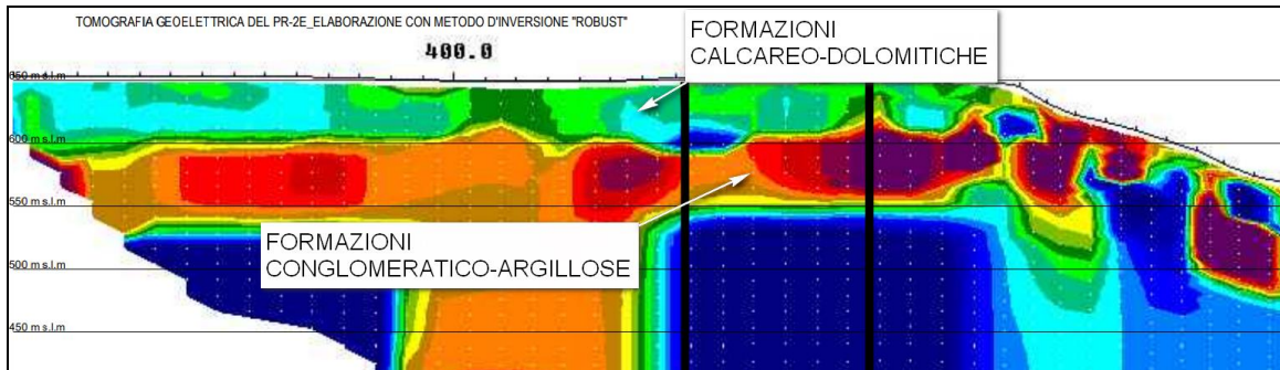
Figura 31 - Discontinuità sub-orizzontale tra la Formazione di Dorgali ed i terreni sottostanti
