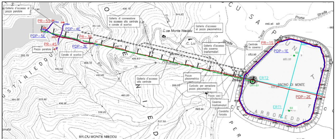
Figura 3 - Piano di posizione generale sul layout del Progetto di Massima
