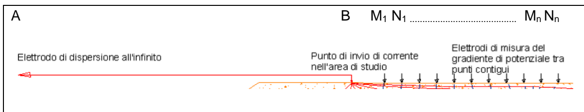
Figura 9 - Dispositivo Polo-Dipolo
