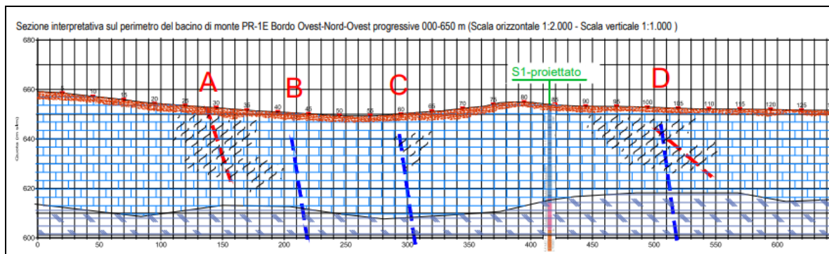
Figura 27 - Sezione interpretativa per le fondazioni sul lato Ovest-Nord-Ovest del Bacino
