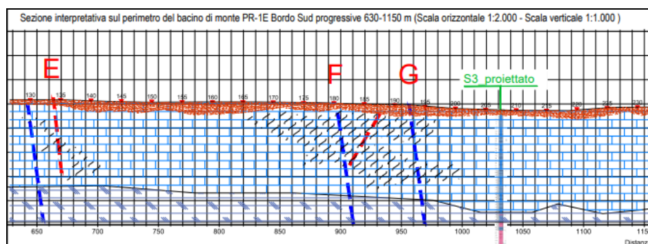
Figura 28 - Sezione interpretativa per le fondazioni sul lato Sud-Sud-Ovest del Bacino
