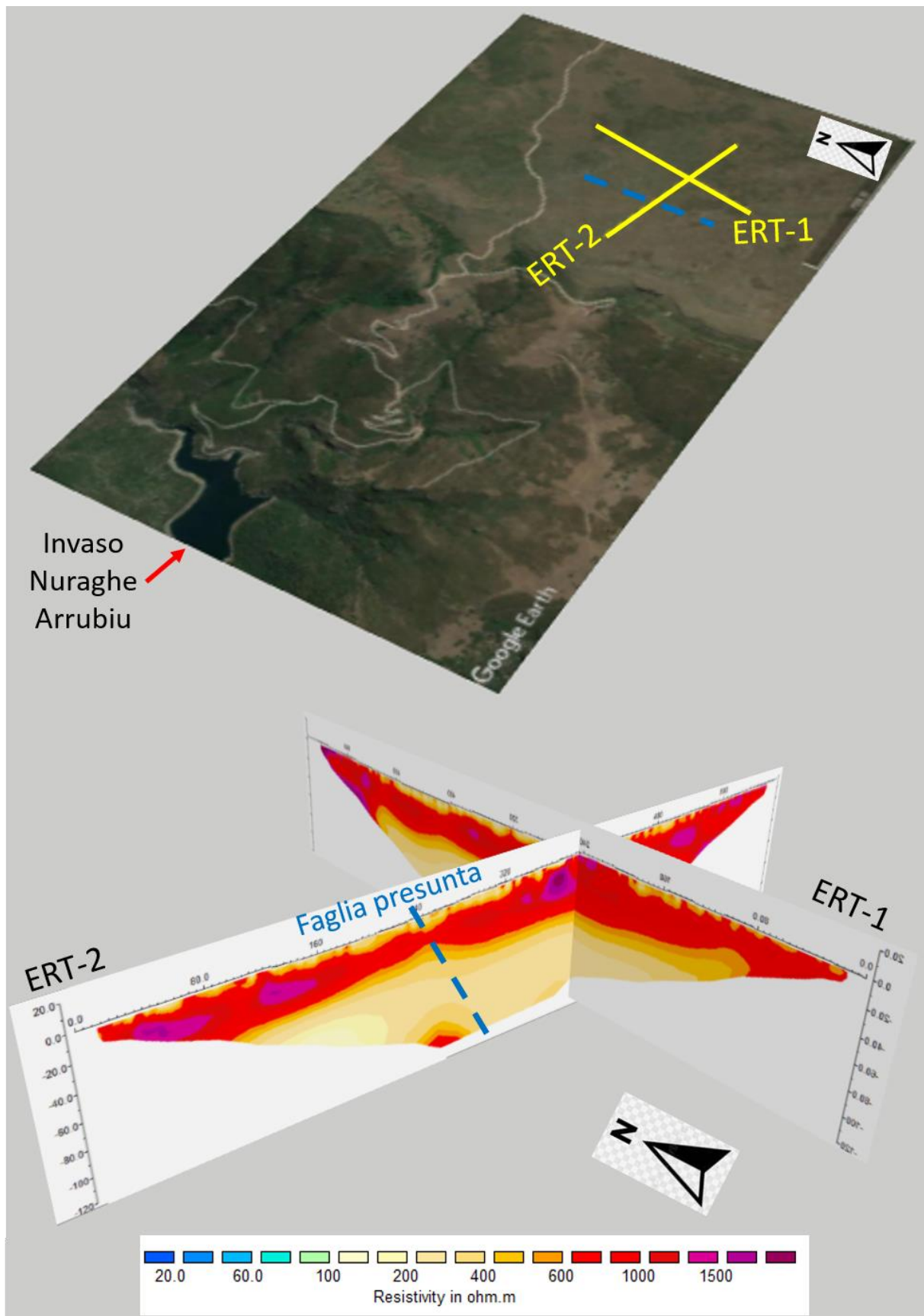
Figura 12 – Visione 3D dell'intersezione tra le tomografie ERT-1 e ERT-2 da SUD-OVEST. Con la linea blu tratteggiata è riportata la faglia presunta.
