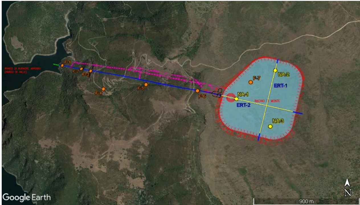
Figura 9 Immagine satellitare del terreno individuato per la realizzazione del bacino di monte: - linee gialle (profili ERT); - linea blu ( waterway ); - linee fucsia (gallerie di accesso necessarie per lo scavo delle opere in sotterraneo); - cerchi gialli (sondaggi previsti); - cerchi arancione (rilievi strutturali programmati).
