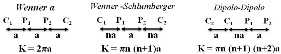
Figura 6 Configurazioni elettrode e relativi fattori geometrici di alcuni stendimenti impiegati in ambito geologico.
