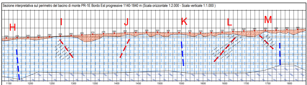
Figura 29 - Sezione interpretativa per le fondazioni sul lato Est-Sud-Est del Bacino
