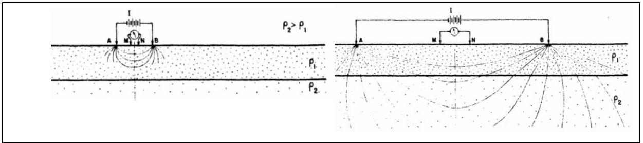
Figura 8 - Differenti profondità di penetrazione del segnale al variare delle dimensioni
