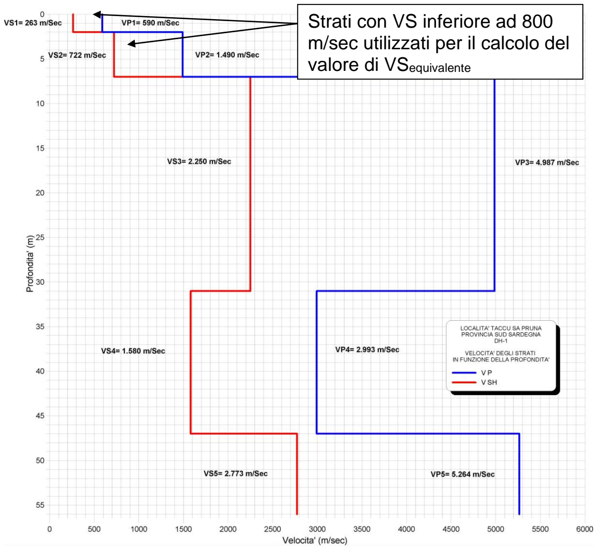
Figura 24 - Down-Hole DH-S1_Diagramma delle velocità delle onde P d SH
