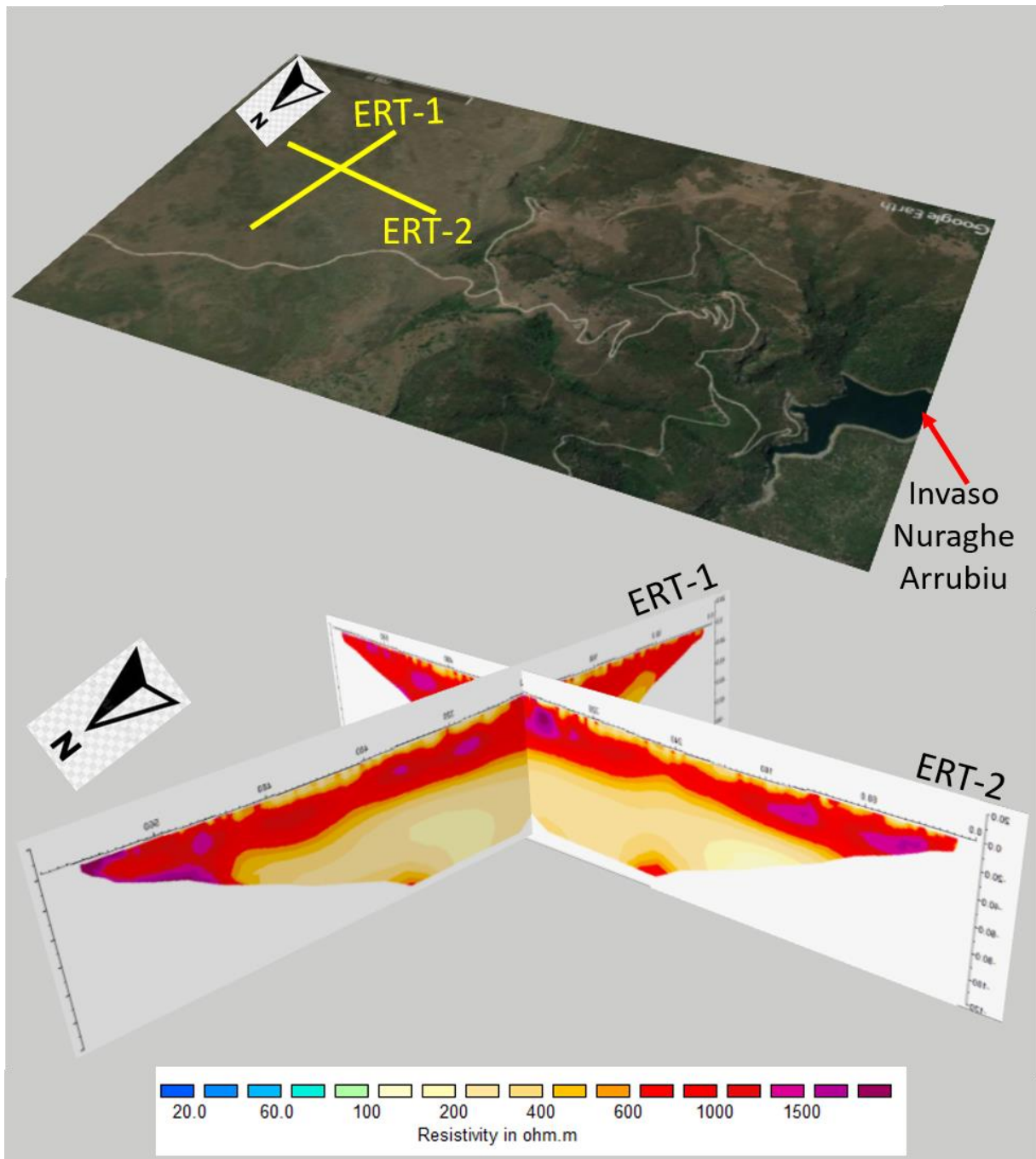
Figura 13 – Visione 3D dell'intersezione tra le tomografie ERT-1 e ERT-2 da NORD-OVEST.
