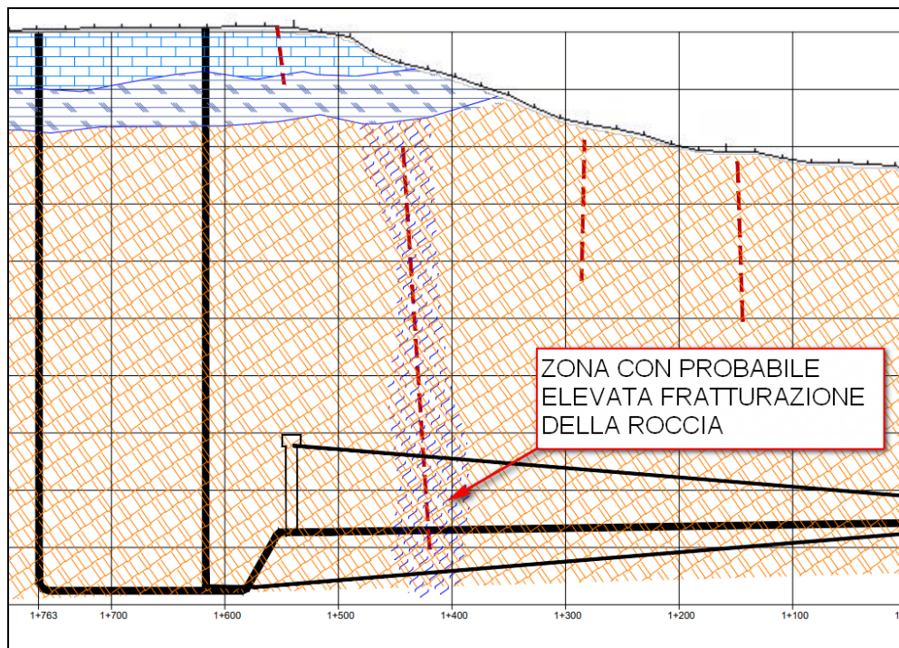
Figura 33 - Zona di intensa fratturazione tra la P.k. 1+390 ed 1+450 della galleria di scarico
