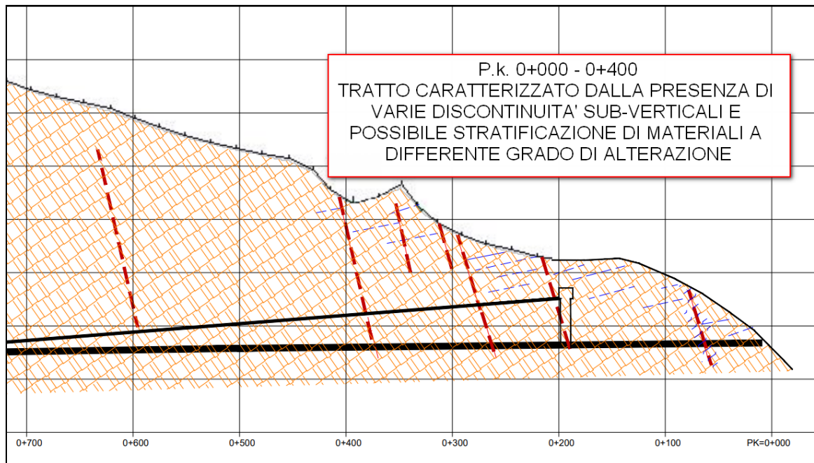
Figura 34 - Zona potenzialmente intensamente fratturate alla P.k. 0+000 - 0+400
