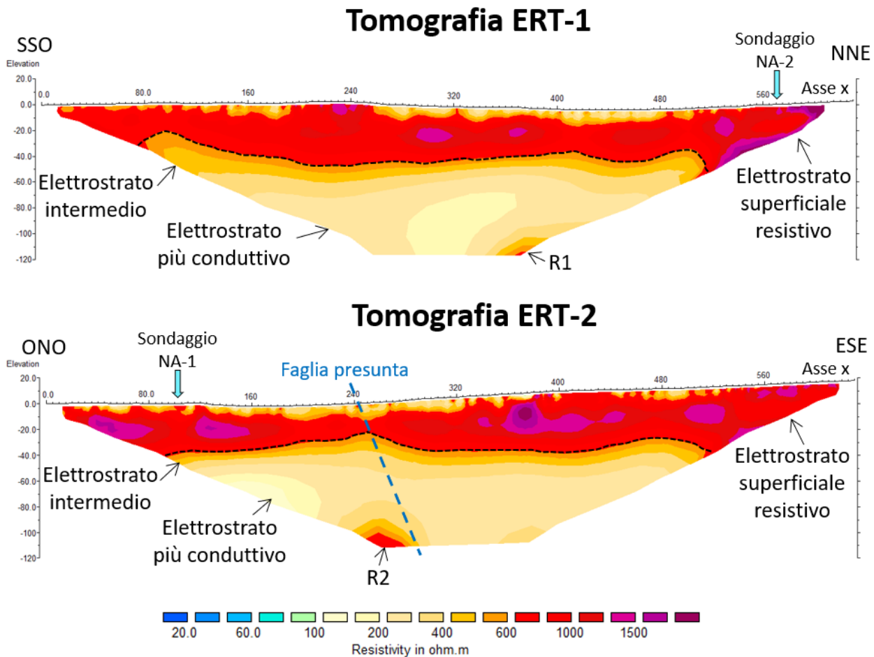
Figura 10 Tomografie elettriche ERT-1 e ERT-2. La linea nera tratteggiata indica il contatto stratigrafico tra le dolomie resistenti e le siltiti più conduttive; la linea blu tratteggiata segnala una probabile faglia. R1 e R2 sono anomalie resistenti rilevate al margine delle tomografie.
