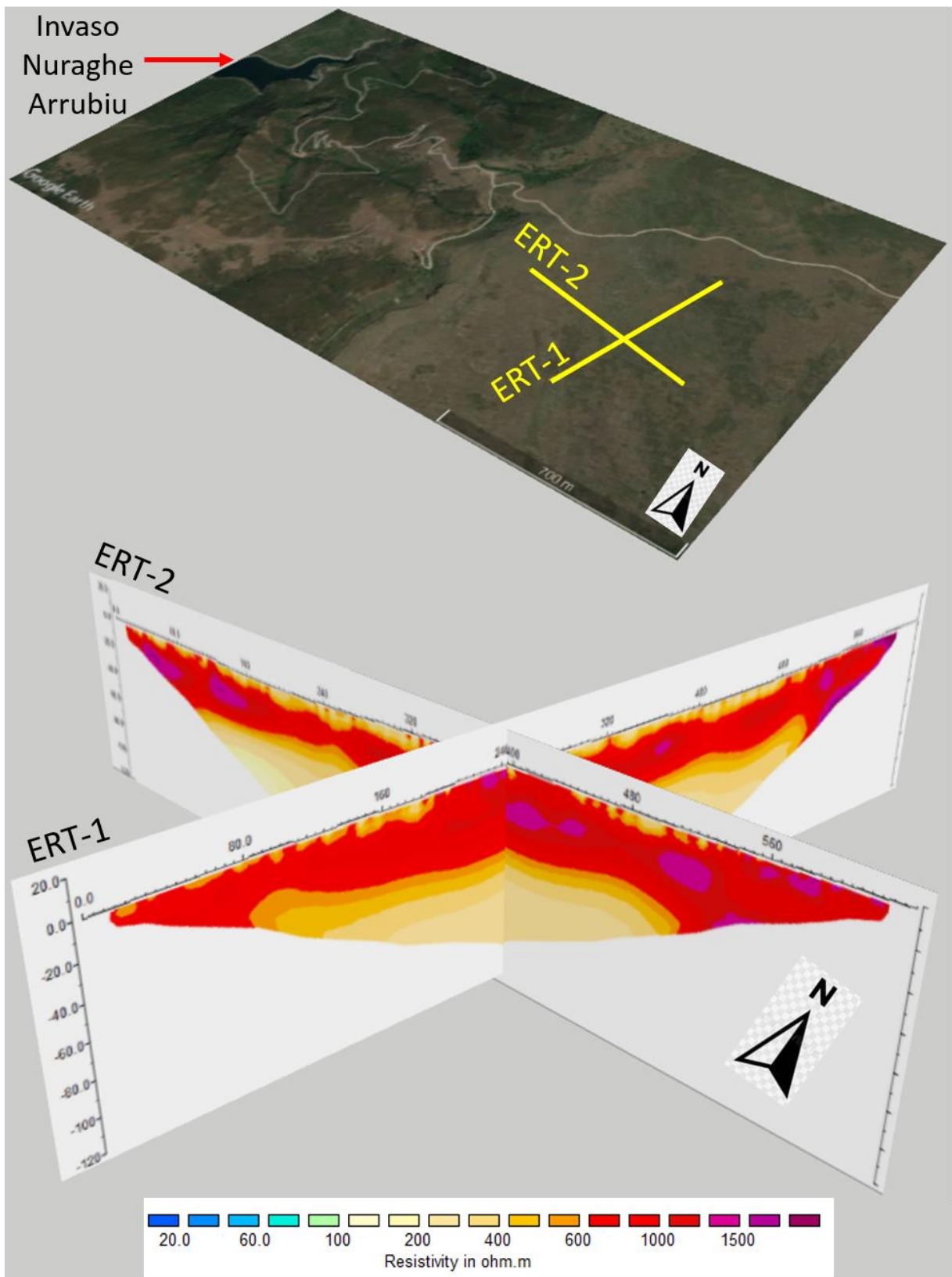
Figura 11 – Visione 3D dell’intersezione tra le tomografie ERT-1 e ERT-2 da SUD-EST.
