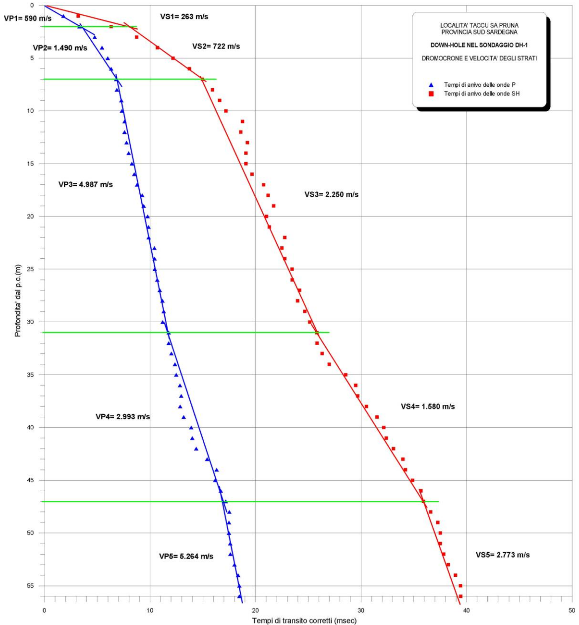
Figura 23 - Down-Hole DH-S1_Dromocrone e calcolo della velocità di strato
