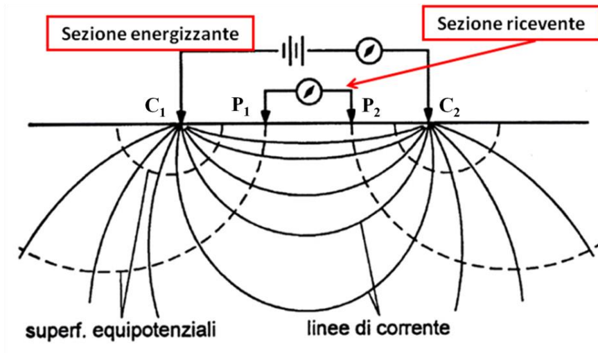
Figura 4 Schematizzazione di un’indagine di resistività. C 1 e C 2 elettrodi di corrente connessi al sistema energizzante; P 1 e P 2 elettrodi di potenziale connessi al sistema ricevente.
