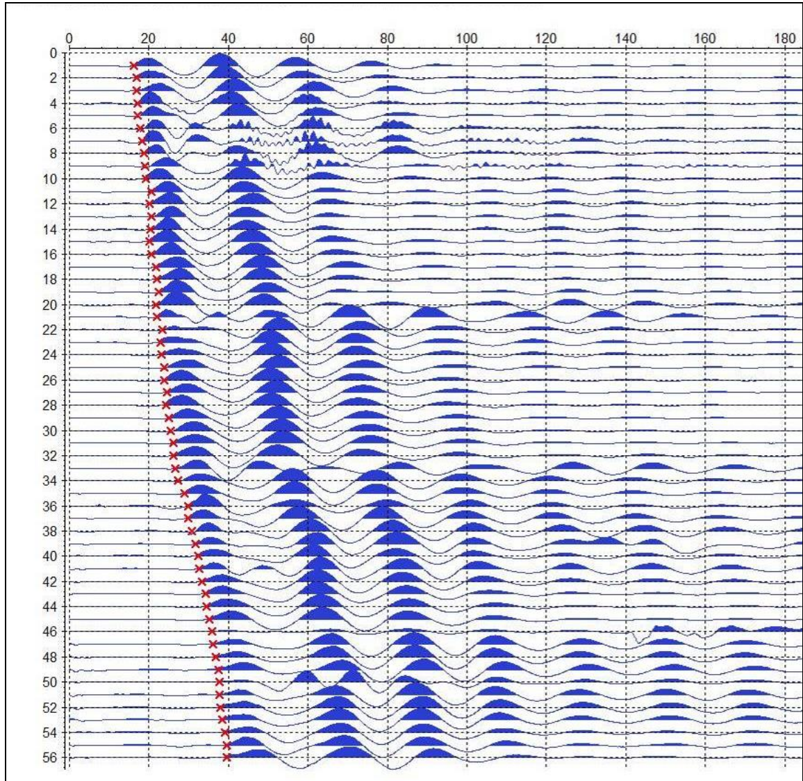
Figura 22 - Down-Hole DH-S1_Onde SH assemblaggio delle tracce del canale 12
