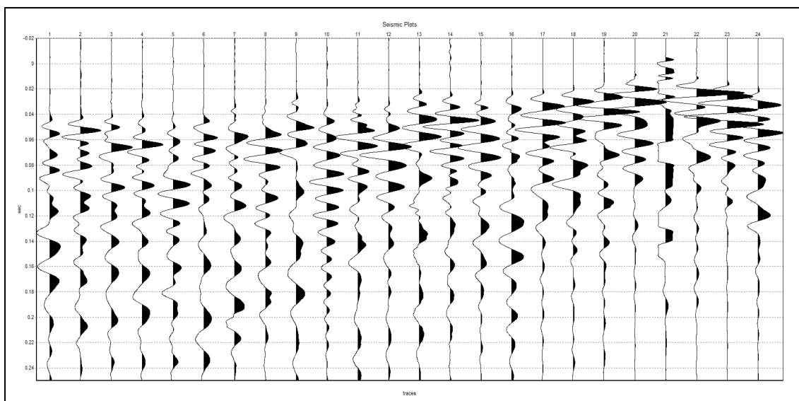
Figura 6 - Sismogramma di campagna
