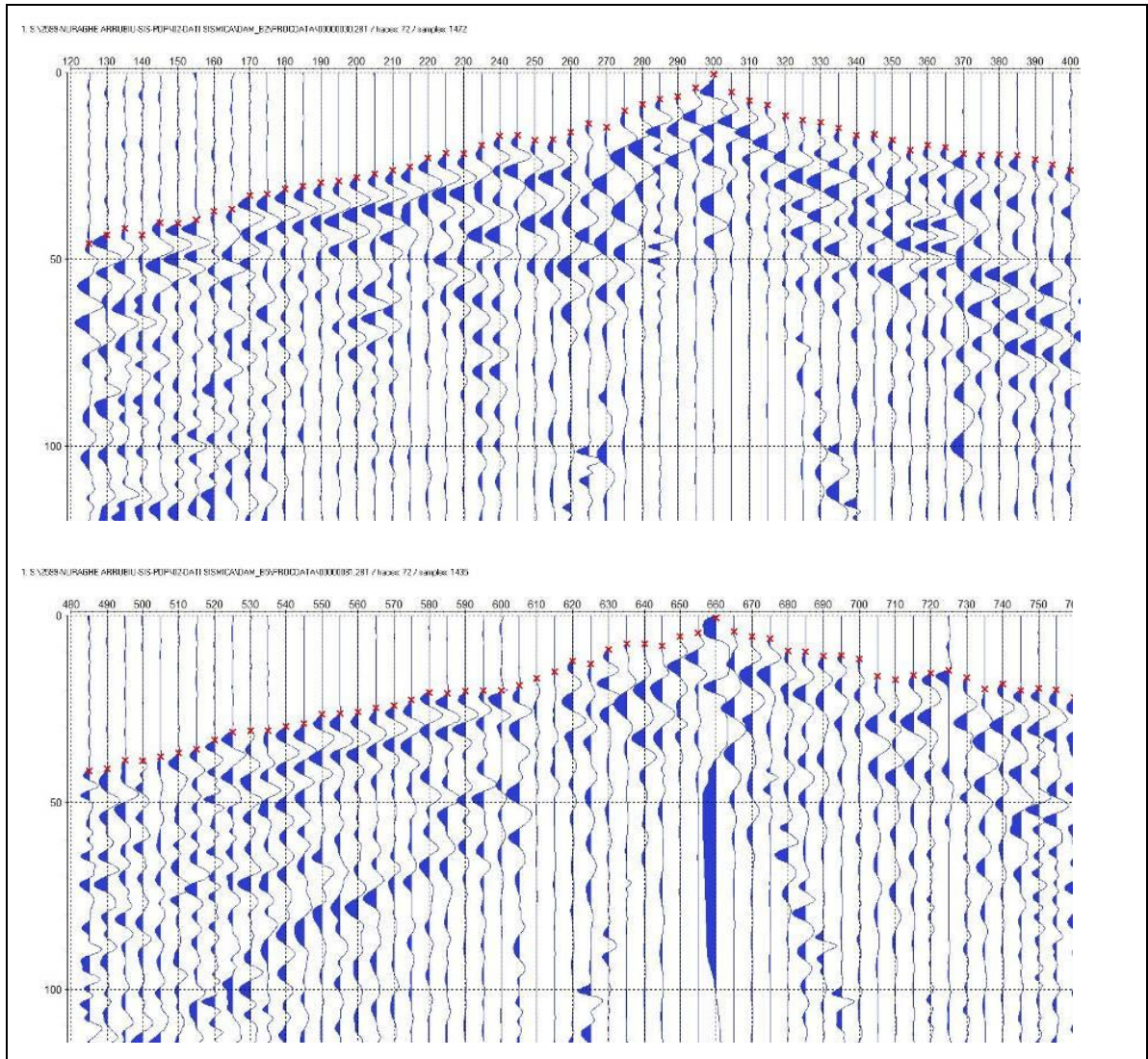
Figura 15 - Individuazione dei primi arrivi
