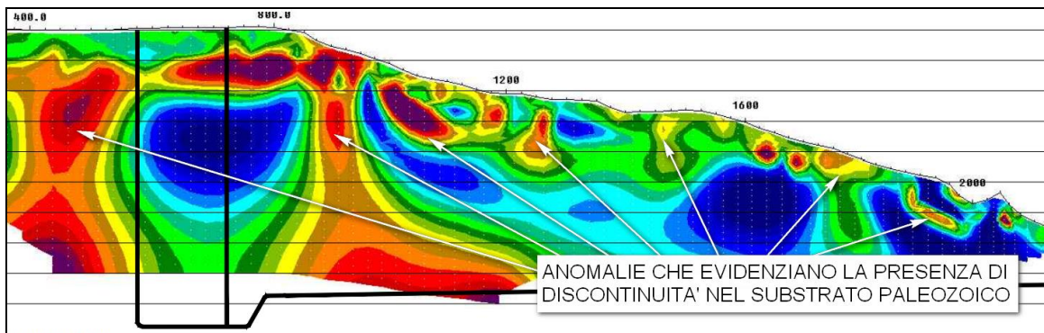
Figura 32 - Discontinuità ad inclinazione variabile nel substrato paleozoico
