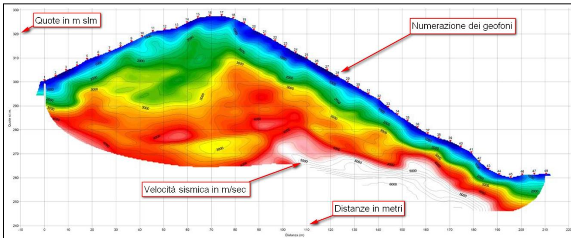
Figura 17 - Tomografia sismica per il profilo PR-4S in onde P
