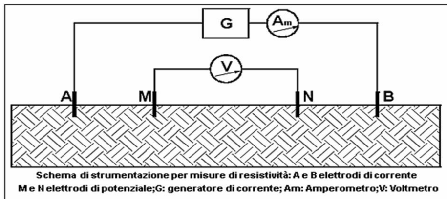
Figura 7 - Schema generico per misure di resistività elettrica
