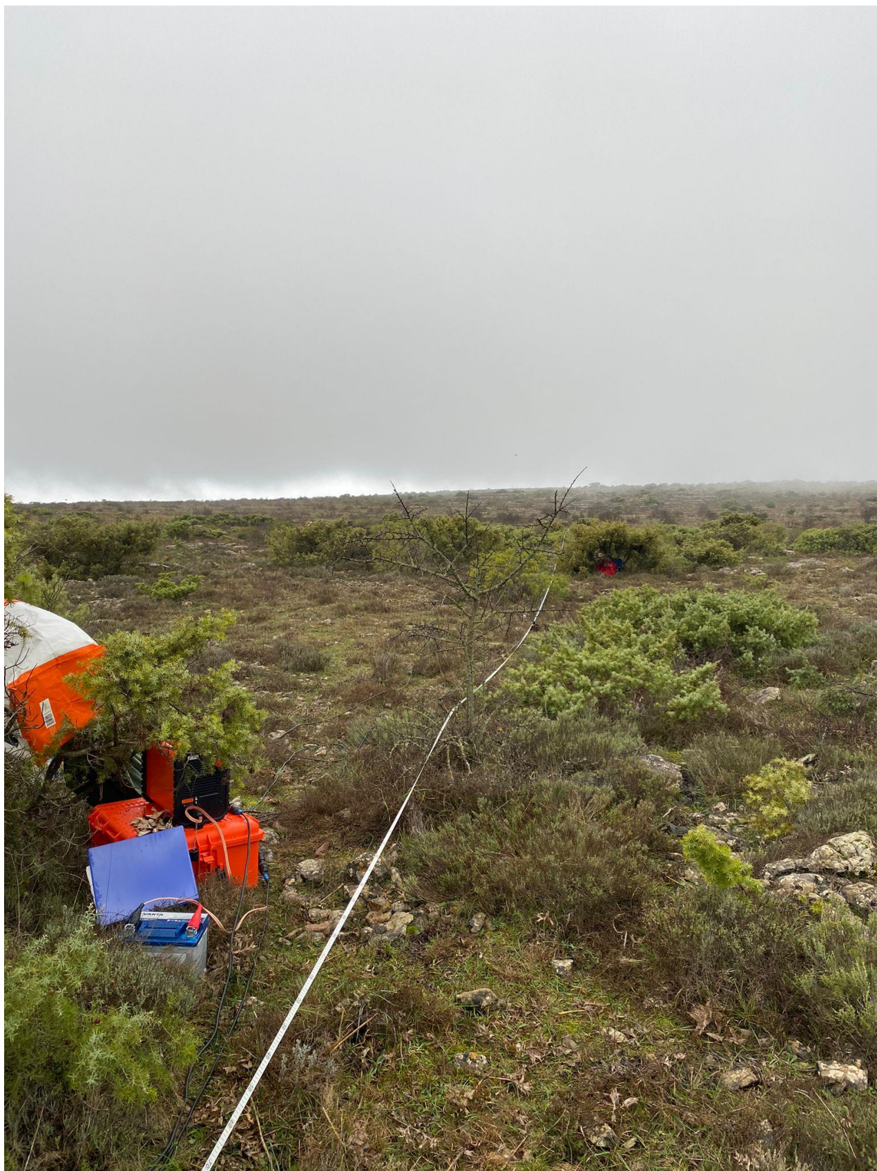
Foto 6 - Posizionamento del georesistivimetro nel punto centrale di ERT-2 durante le fasi di acquisizione.
