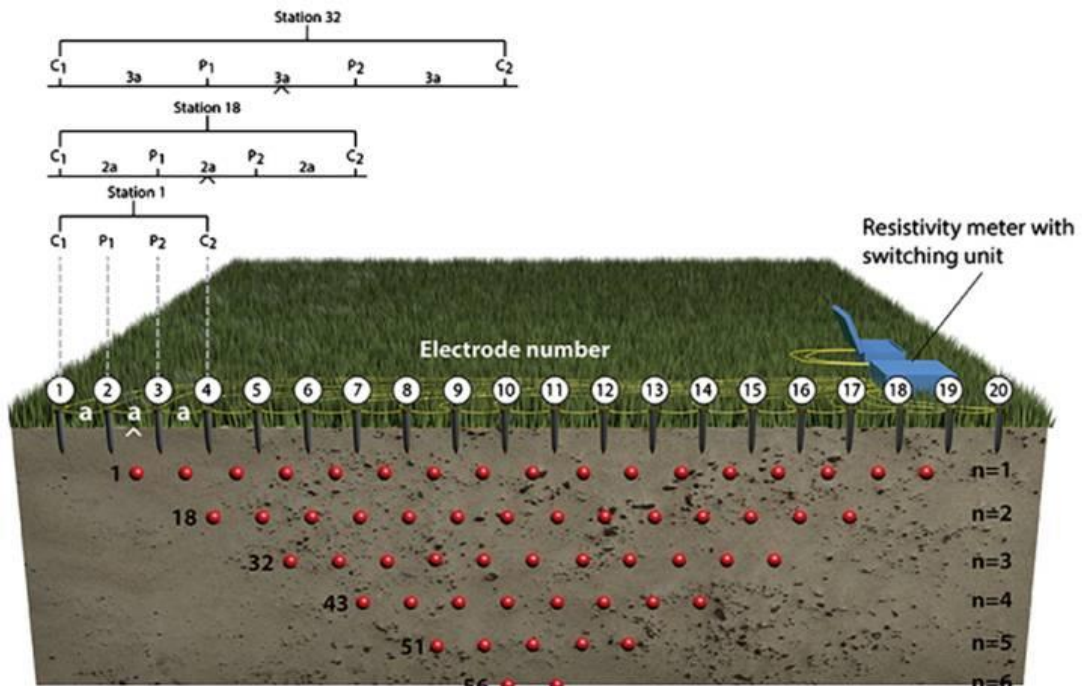
Figura 5 Stendimento multi-elettrodo.
