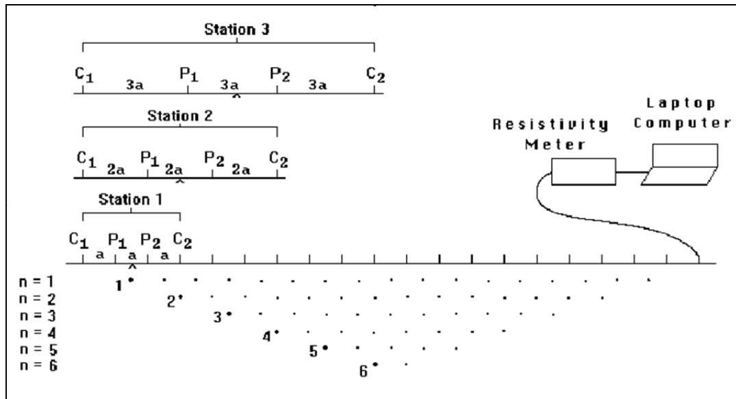
Figura 10 - Approccio multi-elettrodo
