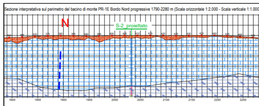
Figura 30 - Sezione interpretativa per le fondazioni sul lato Nord-Nord-Est del Bacino
