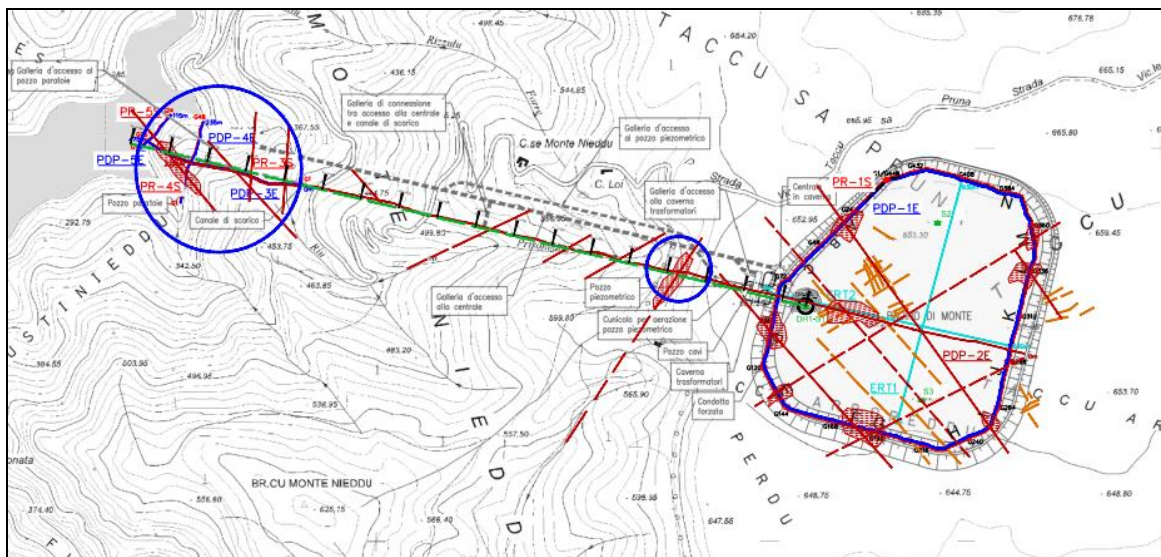
Figura 35 - Mappa di sintesi delle strutture individuate dalla campagna di indagini geofisiche
