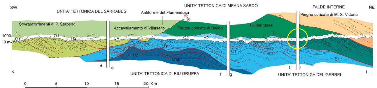
Figura 1 Sezioni geologiche schematiche attraverso la "Zona a falde" del basamento sardo. Il cerchio giallo indica l'area di studio.
