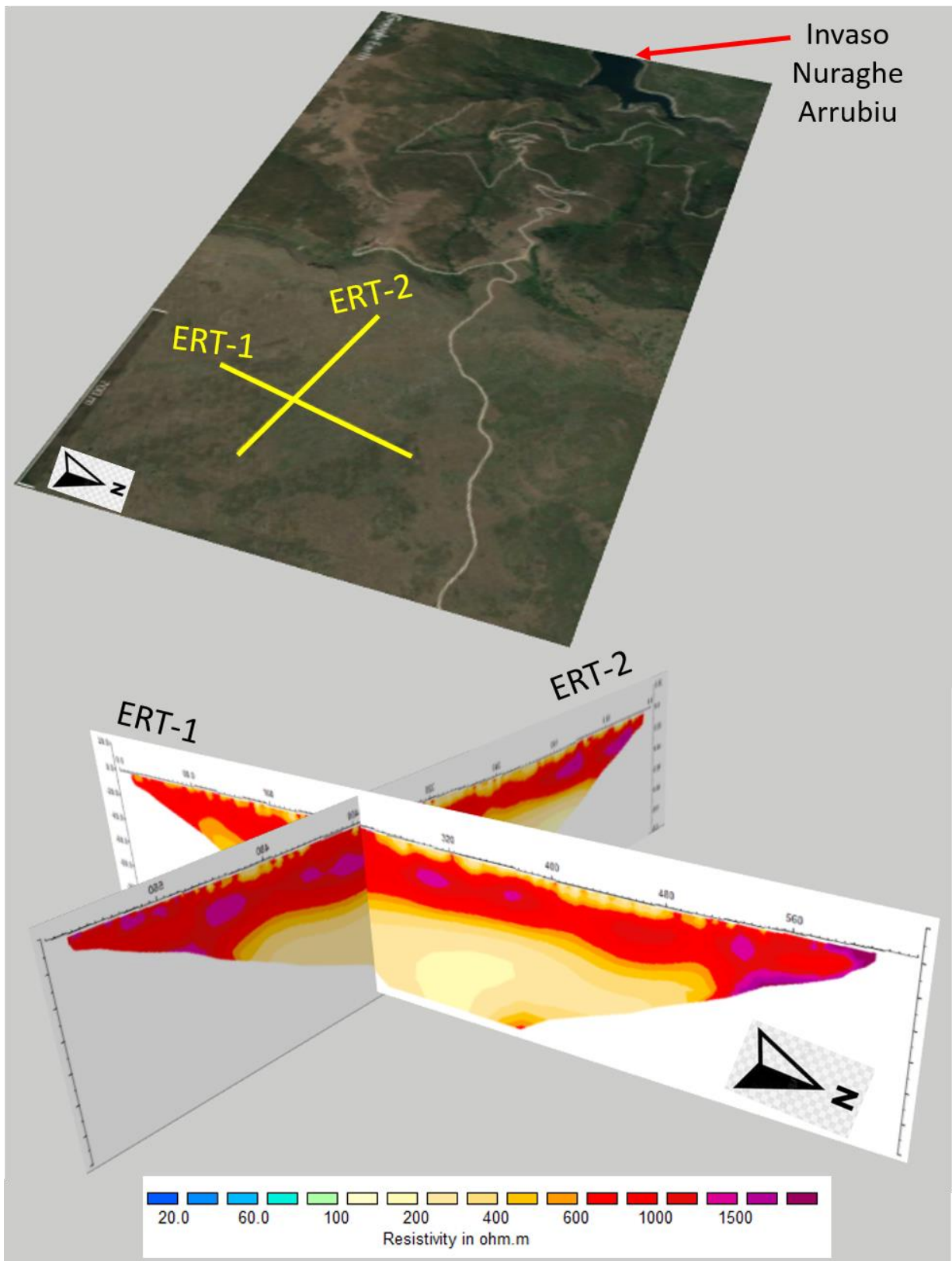
Figura 14 – Visione 3D dell’intersezione tra le tomografie ERT-1 e ERT-2 da NORD-EST.
