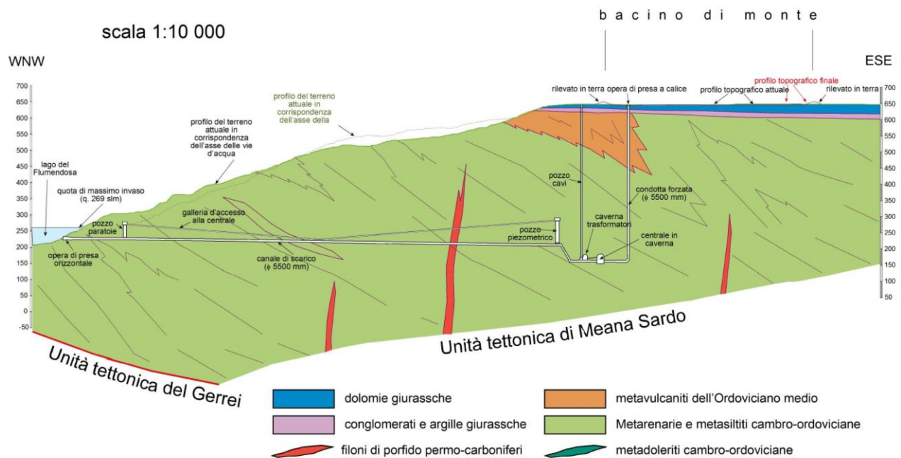
Figura 2 Sezione geologica lungo le opere in progetto (in asse galleria, pozzo piezometrico e centrale in caverna). Si tratta di una sezione interpretativa, pertanto non rappresenta i reali spessori, geometrie ed estensioni delle diverse unità.
