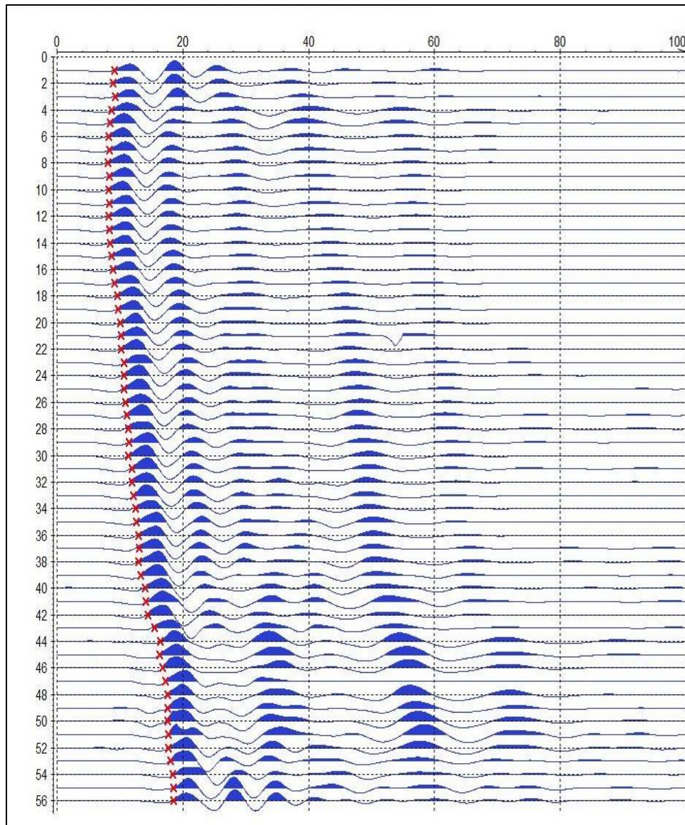
Figura 21 - Down-Hole DH-S1_Onde P assemblaggio delle tracce del canale 1
