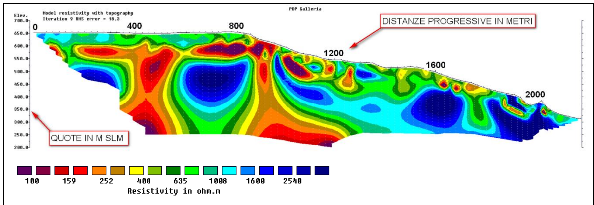
Figura 18 - Profilo geoelettrico profondo PDP-2E (Elaborazione con algoritmo standard )
