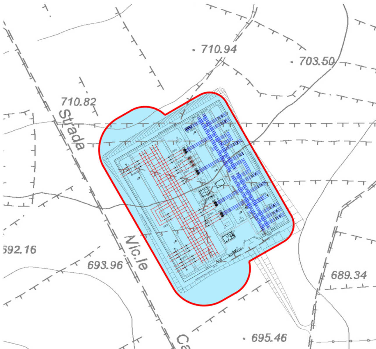
Figura 10. Planimetria con indicazione dell'isolinea a 3 \mu\text{T} (linea color magenta)
