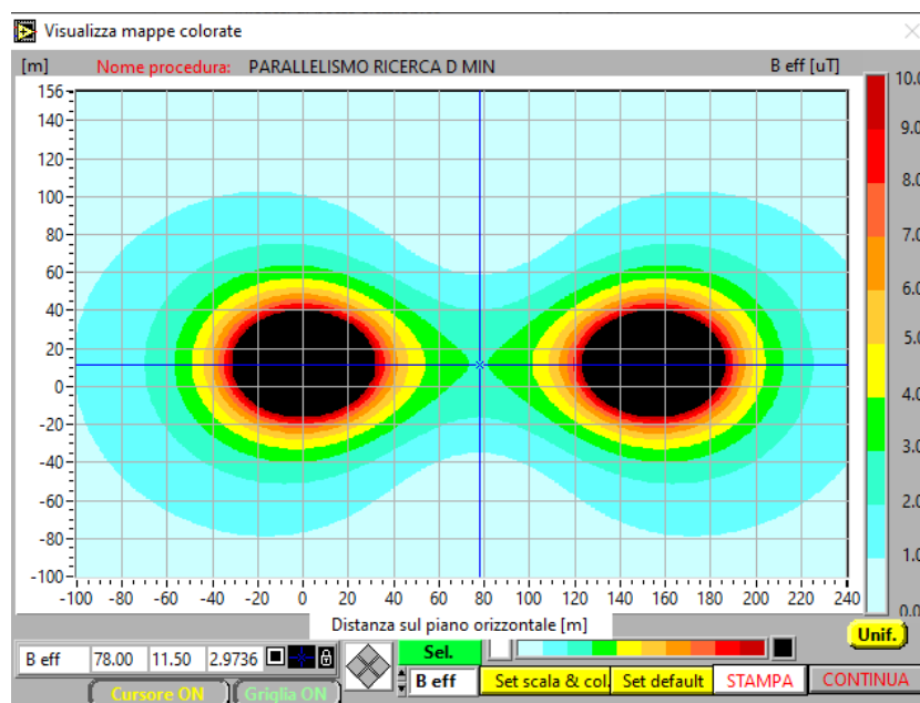
Figura 1-1 Curve isolivello del campo magnetico per linee parallele con interasse di 155 m. Il livello di tensione considerato è pari a 2995 A e la configurazione geometrica delle fasi è pari a quella del sostegno di tipo CA ST 380 kV.
