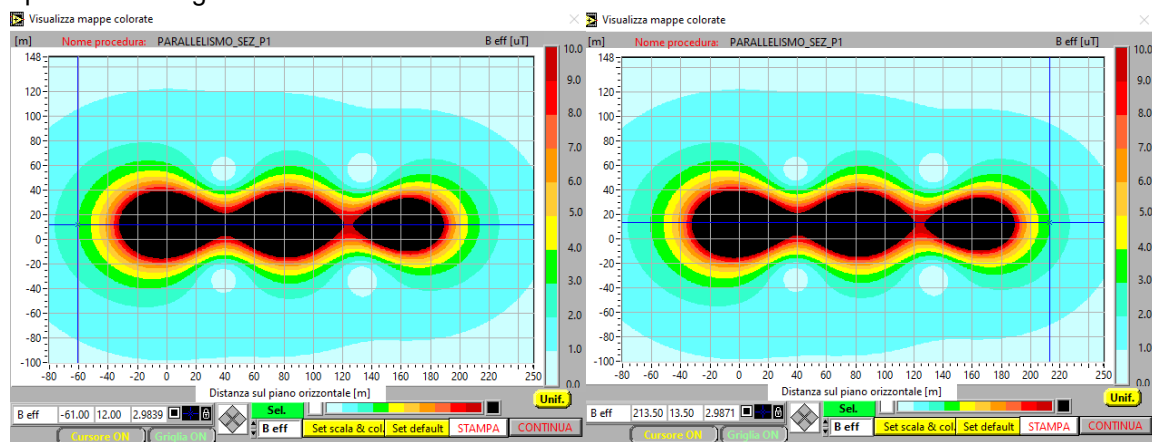
Figura 1-4. Mappa delle curve equivello del campo elettromagnetico in caso di parallelismo di 3 linee aeree a 380 kV poste ad interasse di 81 m.
