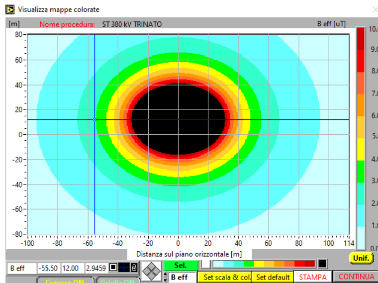
Risultati di calcolo bidimensionale della fascia di rispetto dei 3 \mu T (DPA=56 m+56m).
