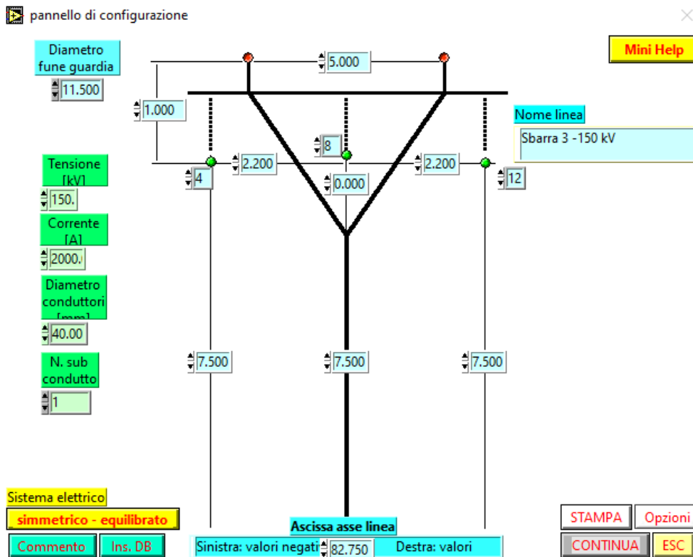
Figura 6. Configurazione geometrica sbarra 3.
