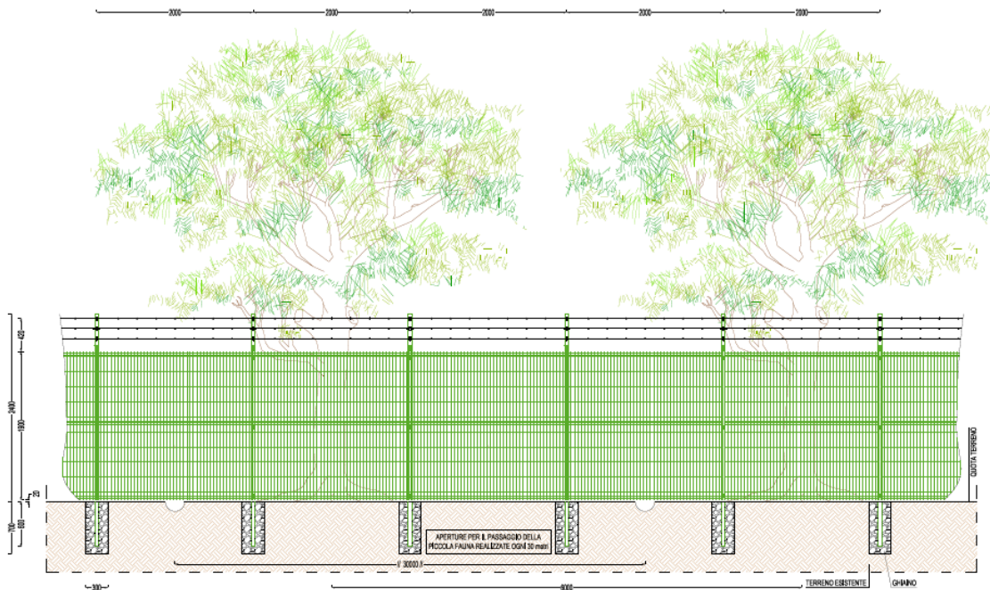
Figura 31: Prospetto recinzione con fascia di mitigazione
