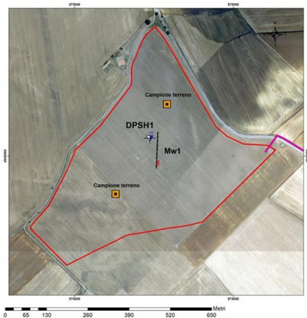
Figura 72: Ubicazione indagini
