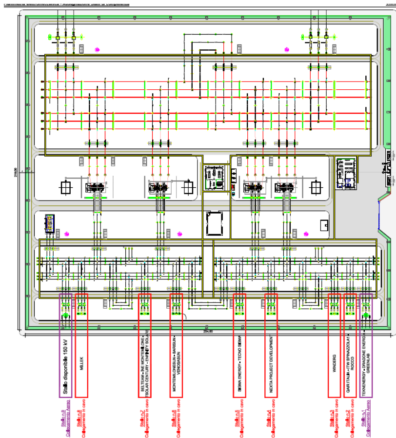
Figura 34: Planimetria SE con ubicazione dell'assegnazione degli stalli
