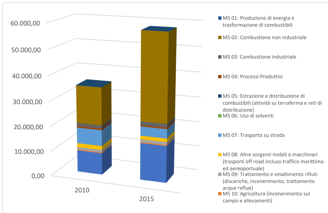
Figura 51: Emissioni totali di CO (Mg) negli anni 2010 – 2015 nella Regione Basilicata (ISPRA, SINANET)
