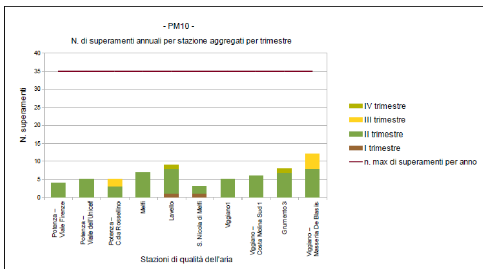
Figura 47: Numero di superamenti annuali aggregate per trimestre
