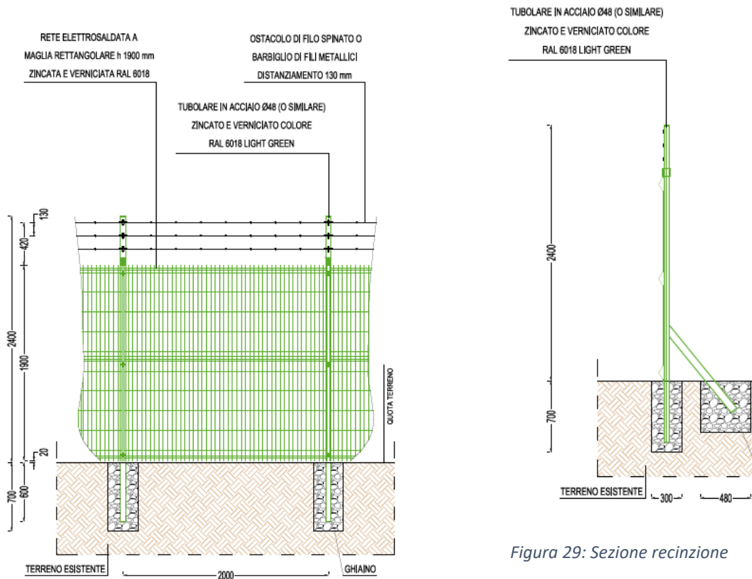
Figura 28: Prospetto recinzione
