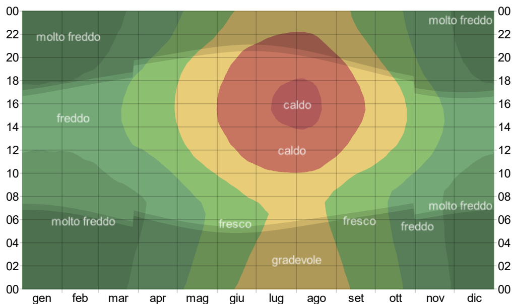
Figura 37: Temperatura oraria media
