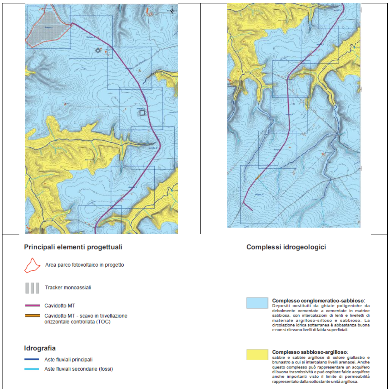
Figura 64: idrogeologia dell'area di intervento
