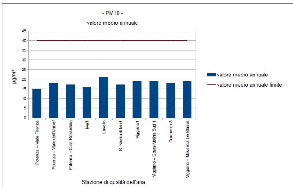
Figura 48: PM_{10} - Valore medio annuo
