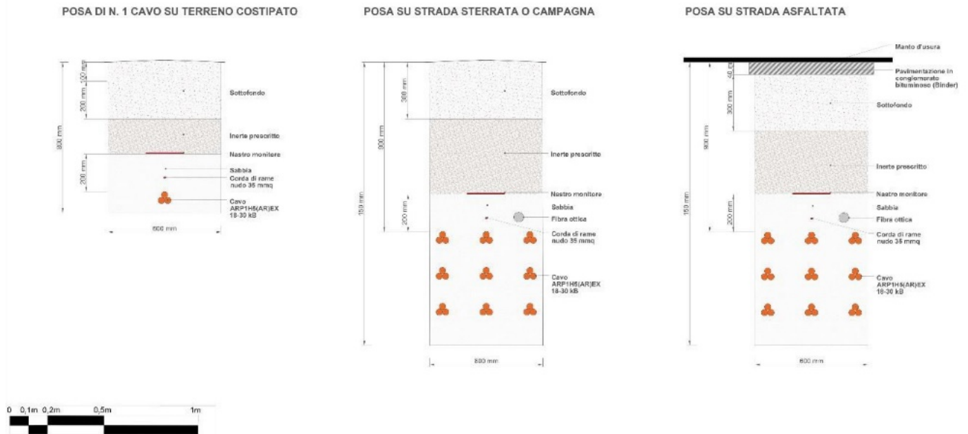
Figura 5: Sezione tipica di posa della linea in cavo
