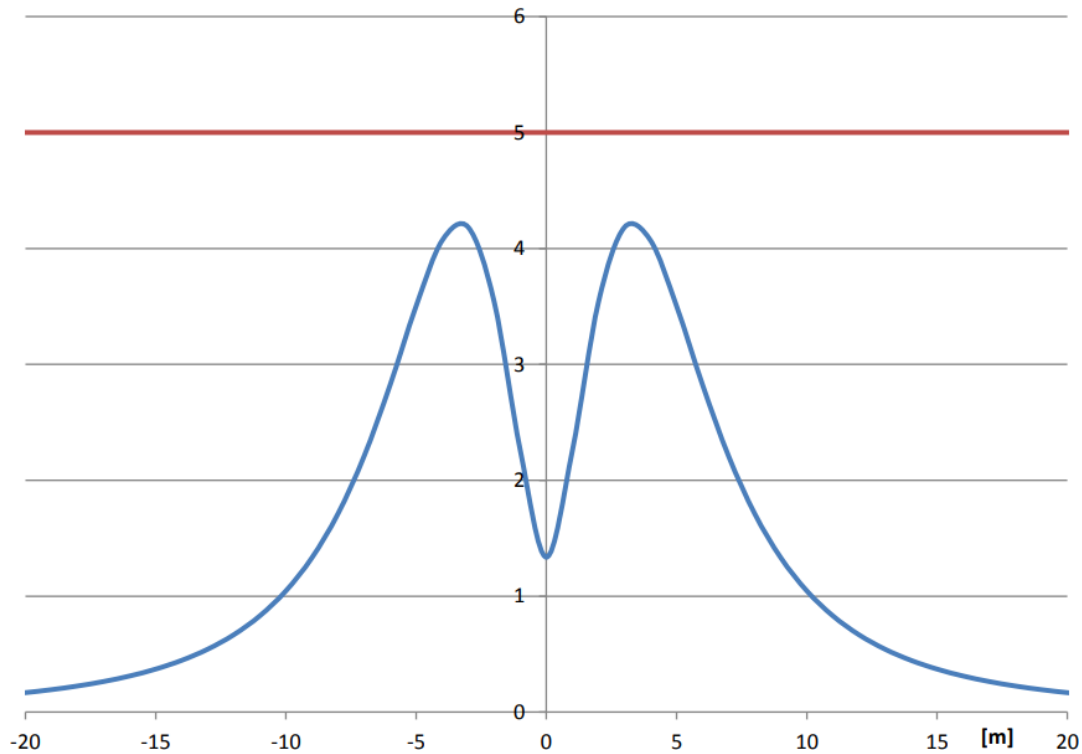
Figura 9: Campo elettrico al suolo generato dal sistema di sbarre a 220 kV
