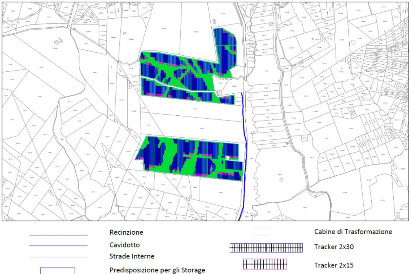
Figura 2 – Layout dell'area d'impianto ricadente nel territorio di Piana degli Albanesi (PA) località Jencheria, su base catastale.
