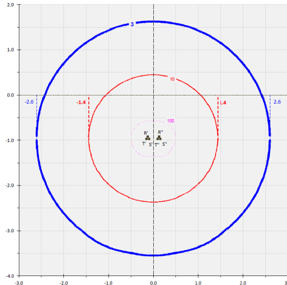
Figura 8: Curve di equivello per il campo di induzione magnetica generato da una linea MT posata a trifoglio ( I_{max}=710\text{A} ; formazione (3x1x630))
