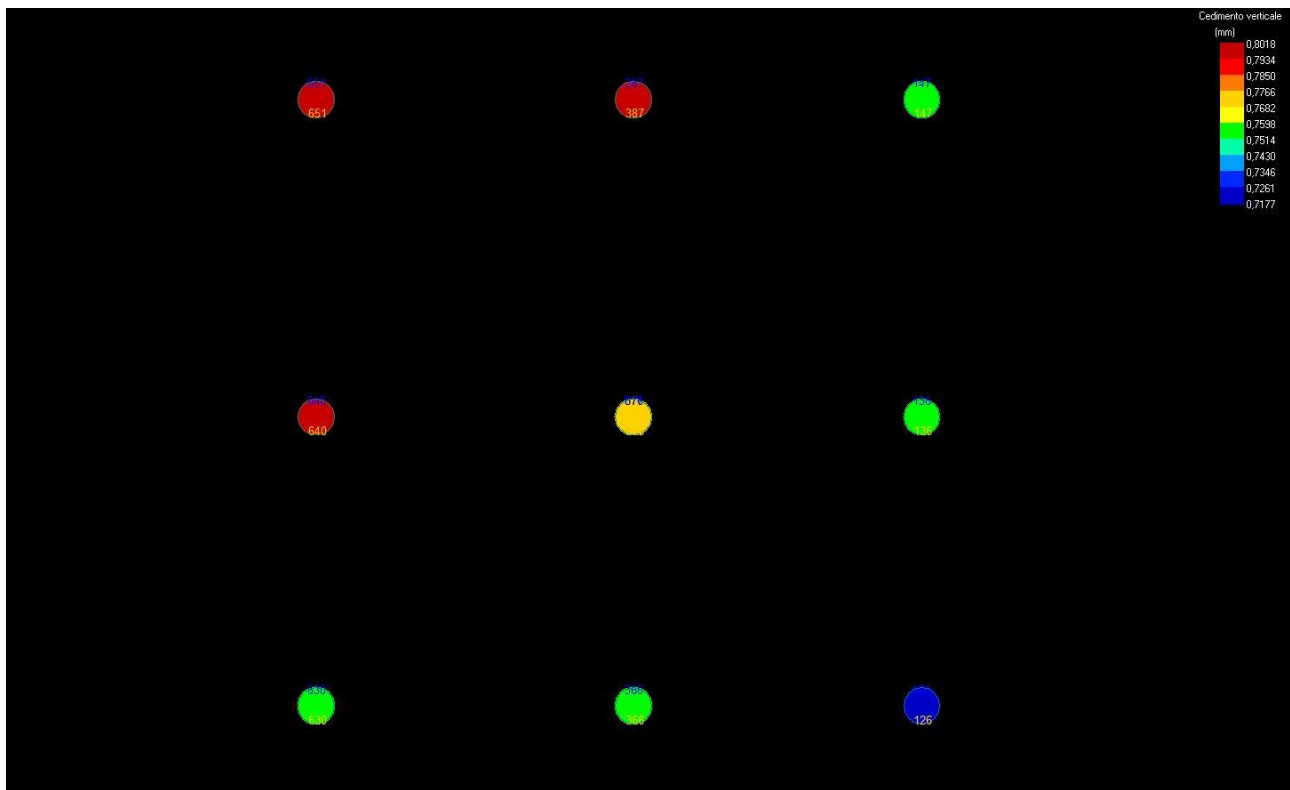
Figura 4 – Cedimenti massimi
