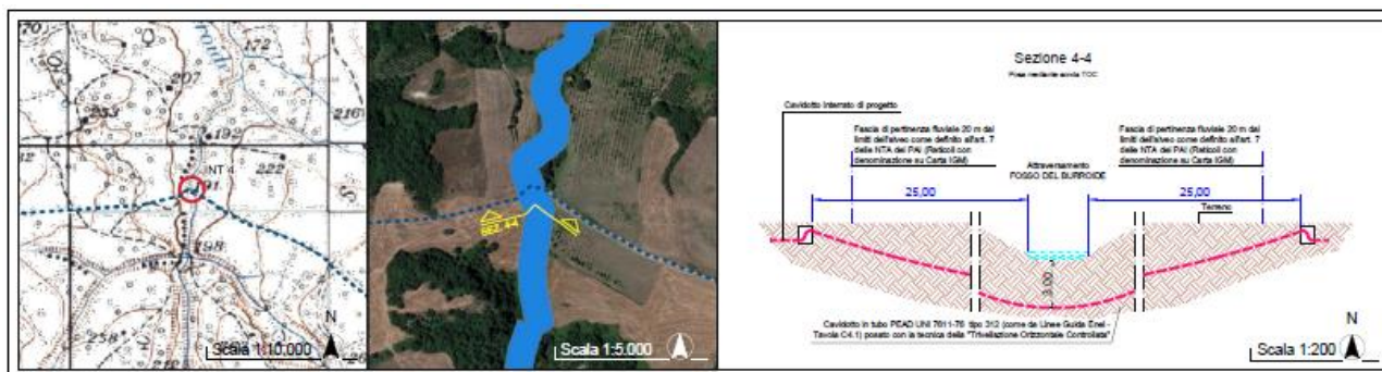
Figura 3--Stralcio studio degli attraversamenti – “F.sso del Burroide” - GLN-CIV-TAV-017 – Studio degli attraversamenti
