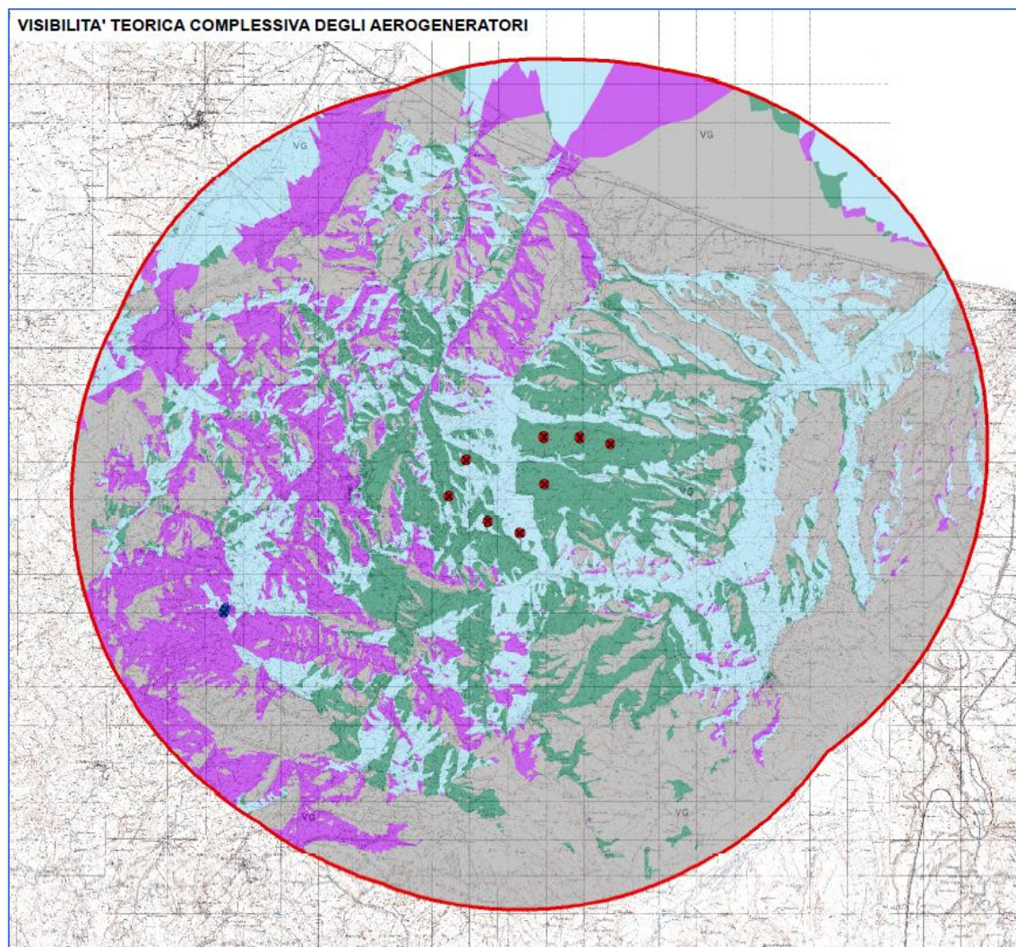
Figura 8 - Visibilità complessiva degli aerogeneratori in progetto e realizzati
