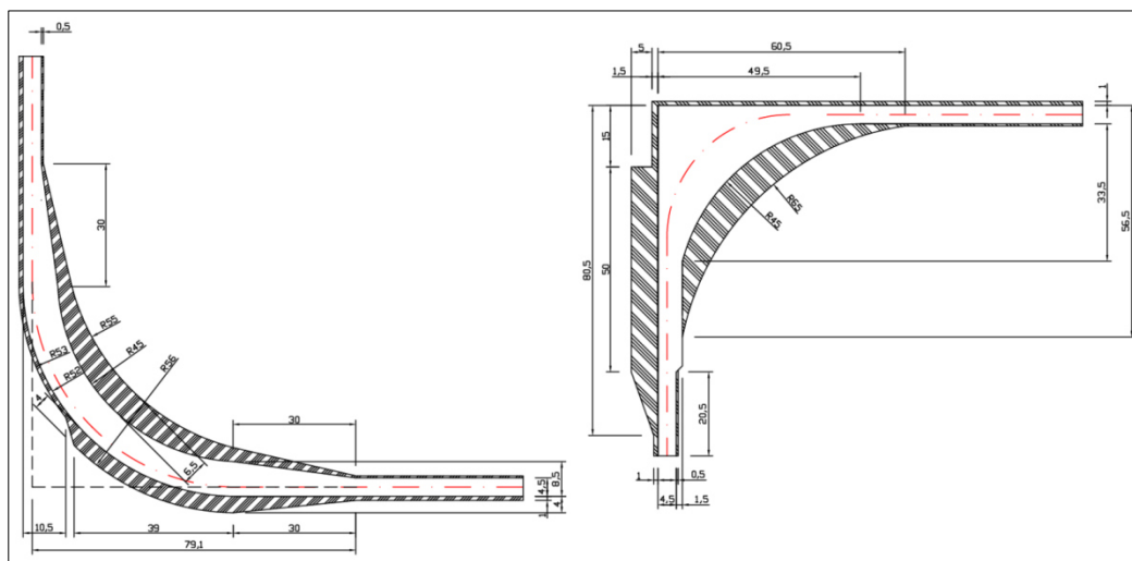
Figura 9 - Particolare realizzazione raccordo strade
