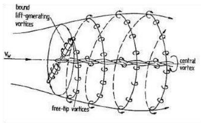
Figura 7 - Vortici e scia
