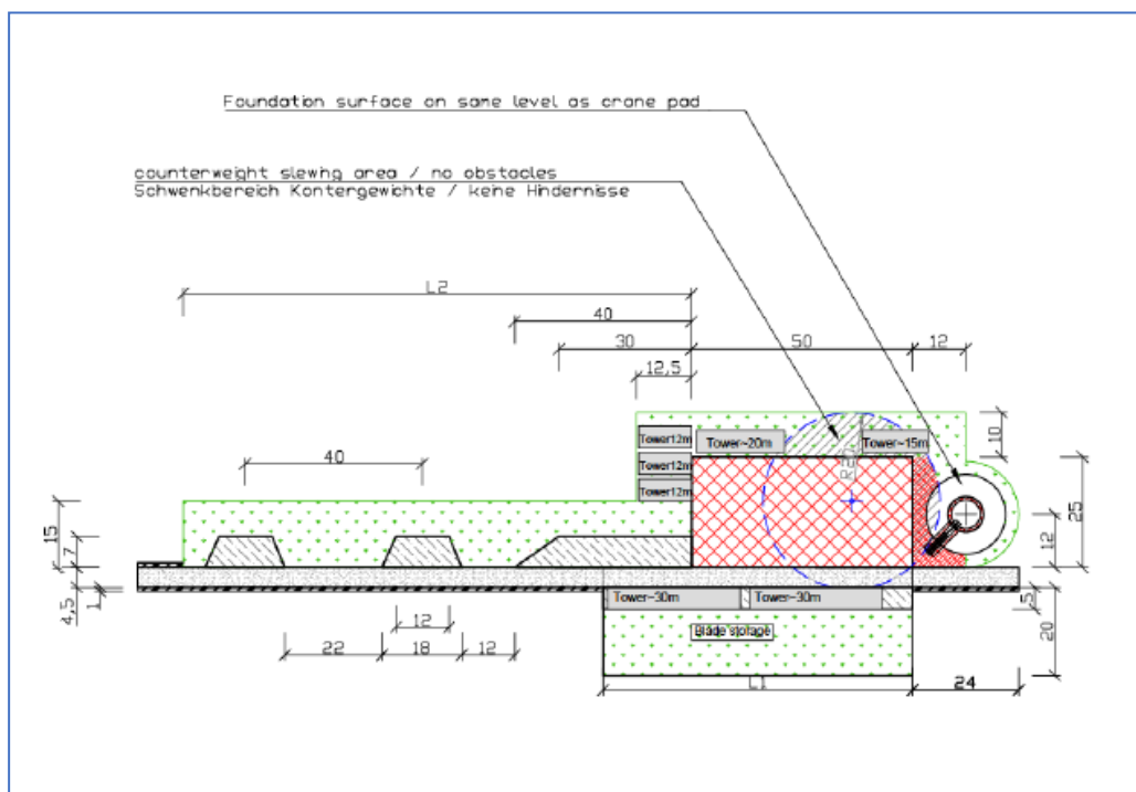
Figura 10 - Piazzola di montaggio
