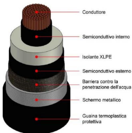
Figura 11 - Esempio di cavo
