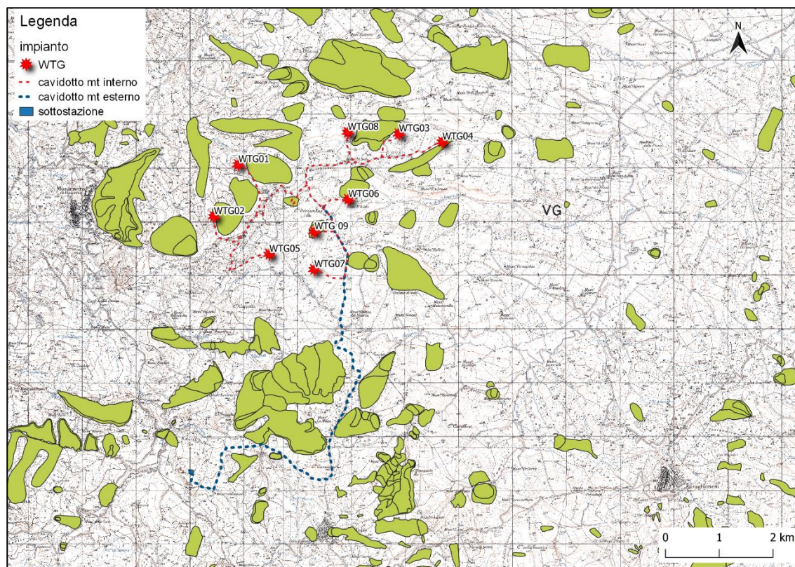
Figura 3 - Ipotesi di layout a 9 aerogeneratori
