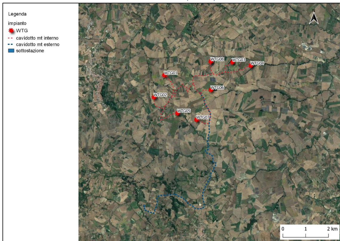
Figura 4 – schema definitivo a 8 WTG
