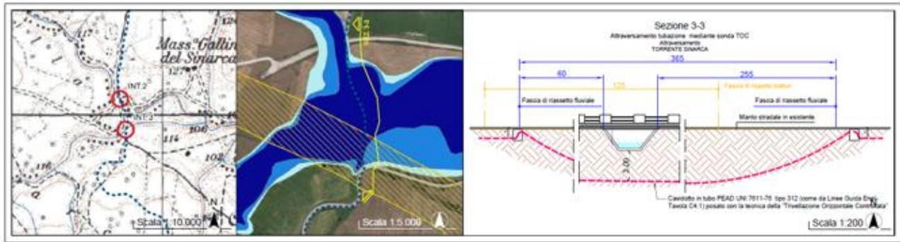
Figura 8--Stralcio studio degli attraversamenti – “Torrente Sinarca” - MNT-CIV-TAV-017 – Studio degli attraversamenti
