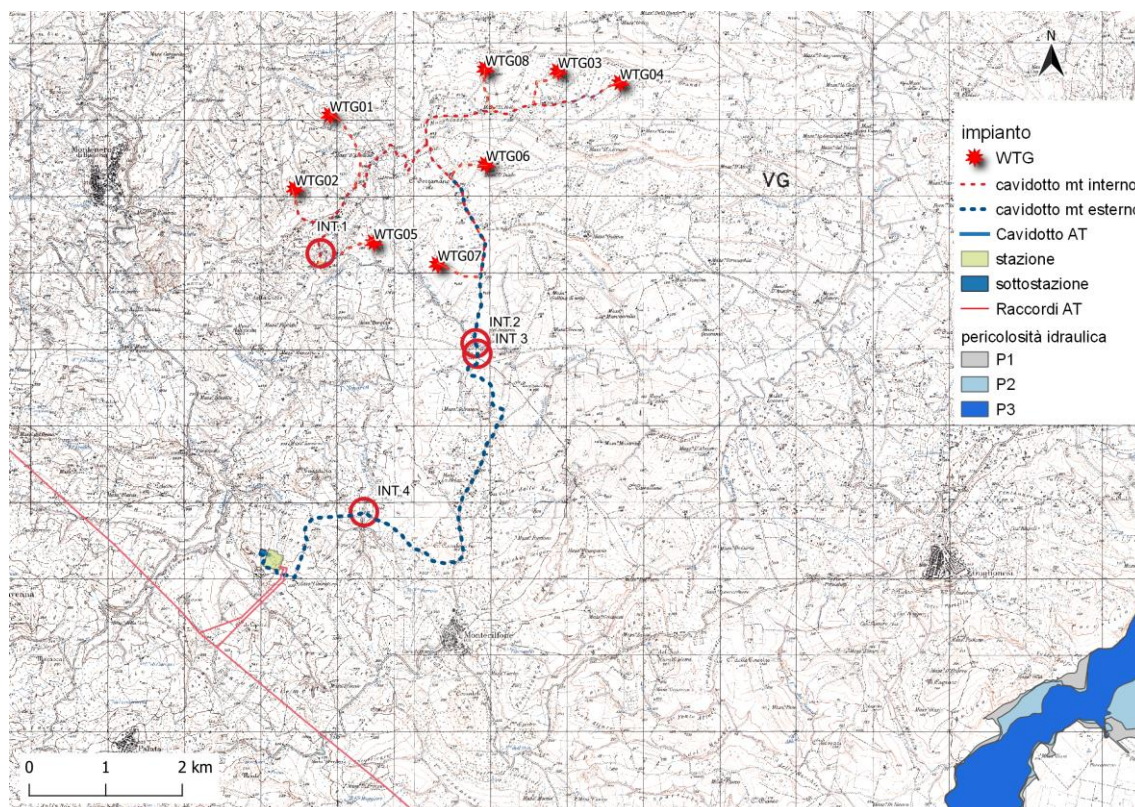
Figura 3 - Inquadramento sul PAI ALLUVIONI - AdB Fiume Biferno
