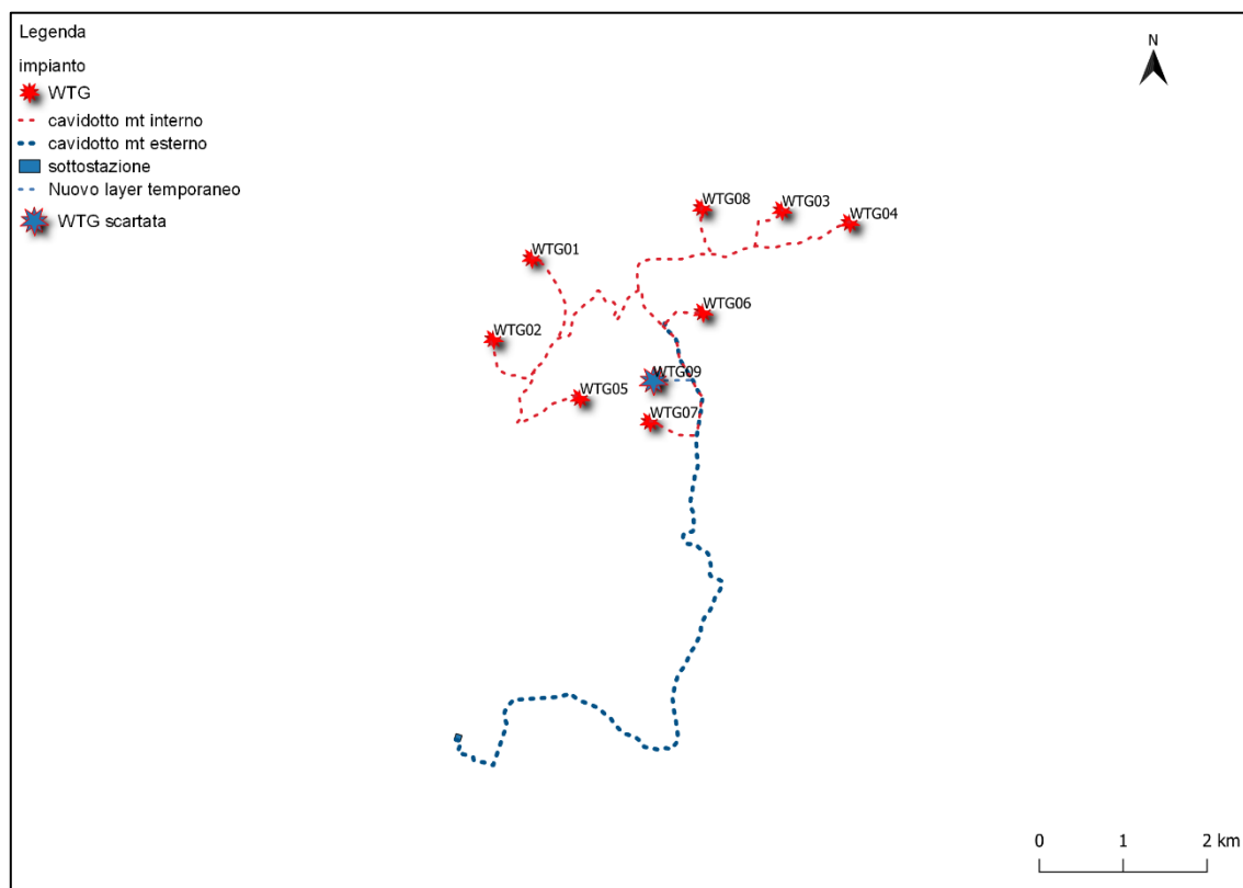
Figura 24 - Sovrapposizione schema layout di partenza a 9 WTG (in blu) e schema definitivo a 8 WTG (in rosso).
