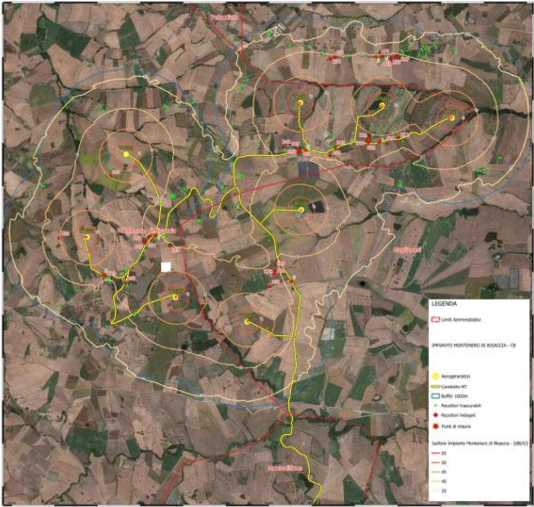
Figura 7 - Stralcio della planimetria delle isofone e recettori
