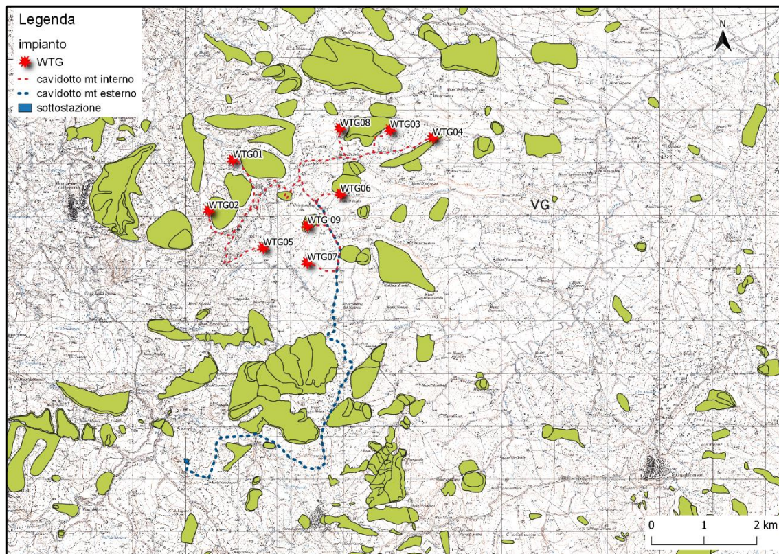
Figura 5 - Ipotesi di layout a 9 aerogeneratori
