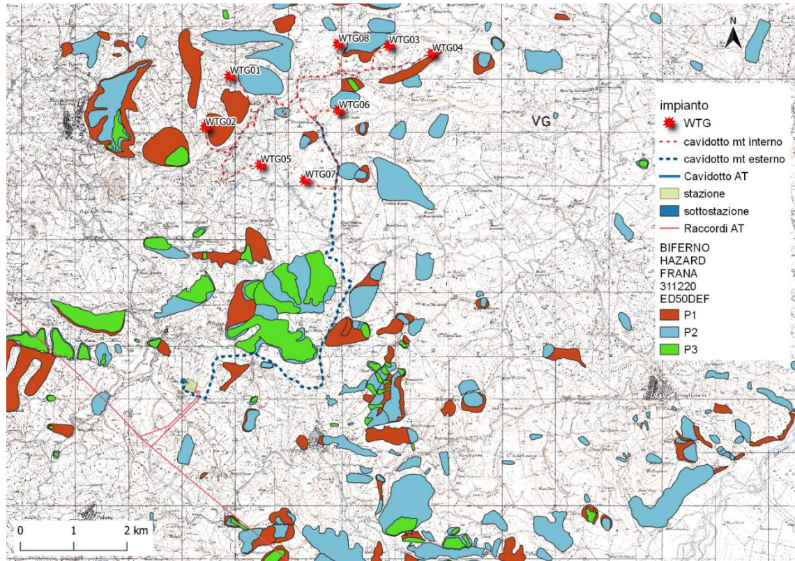
Figura 4 - Inquadramento sul PAI FRANE – AdB Fiume Biferno
