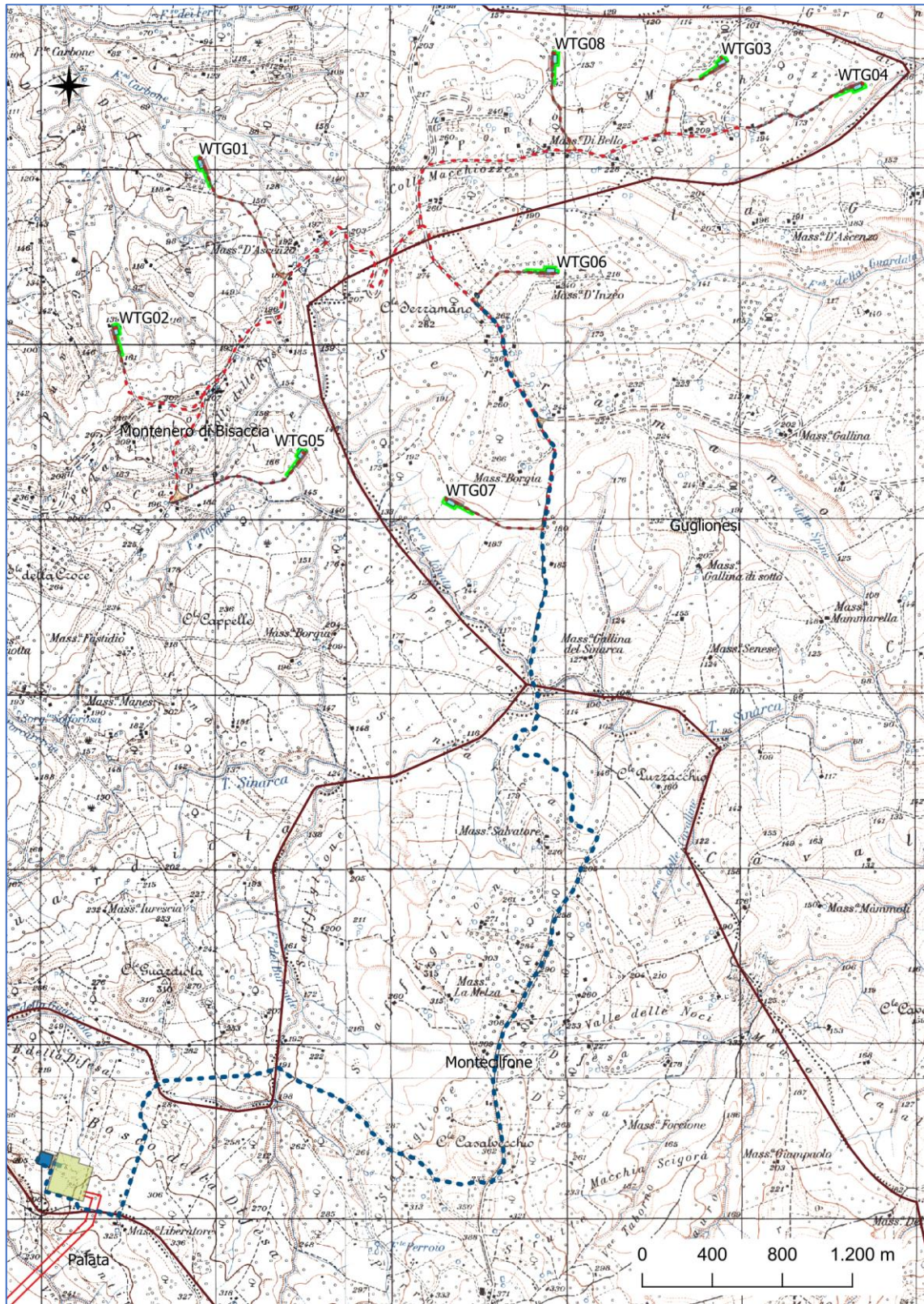
Figura 1 - Inquadramento su IGM
