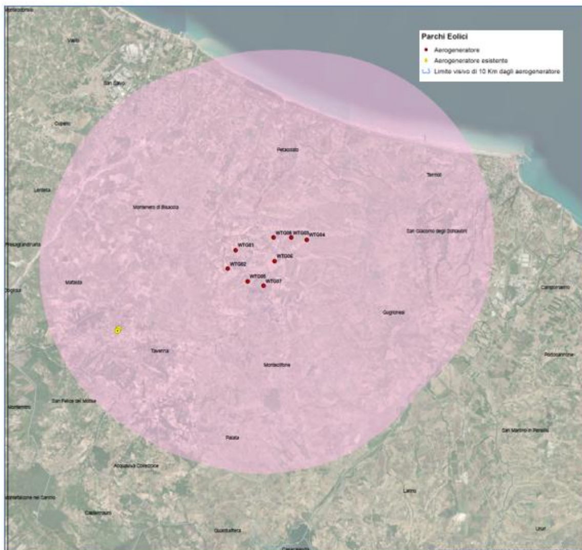
Figura 10 - Inquadramento del Parco eolico rispetto agli altri aerogeneratori realizzati
