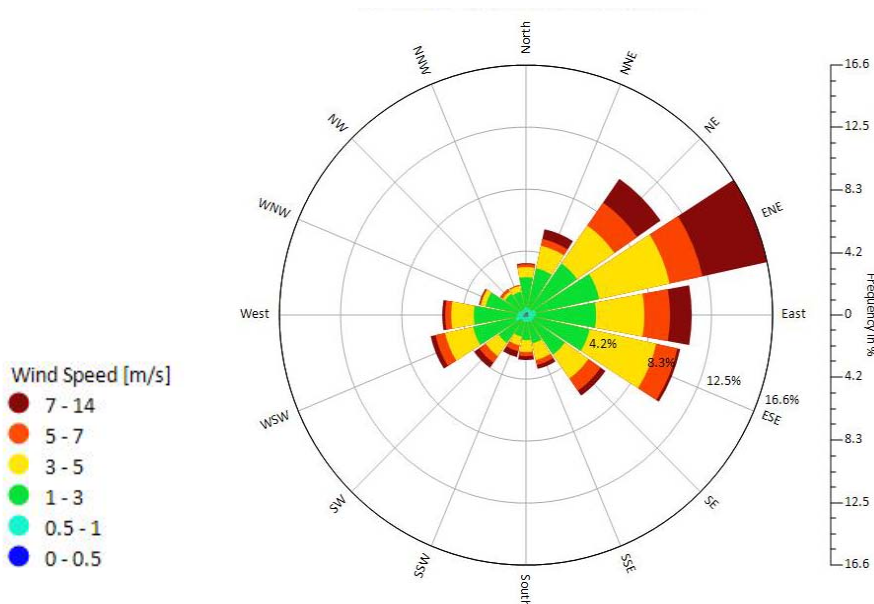
Figura 12 - Rosa dei venti stimata in corrispondenza dello stabilimento Versalis per l'anno 2021 - quota 500 m
