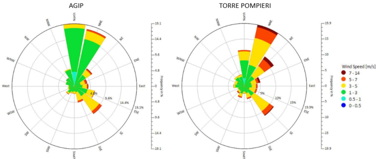
Figura 4 - Rose dei venti per l'anno 2021
