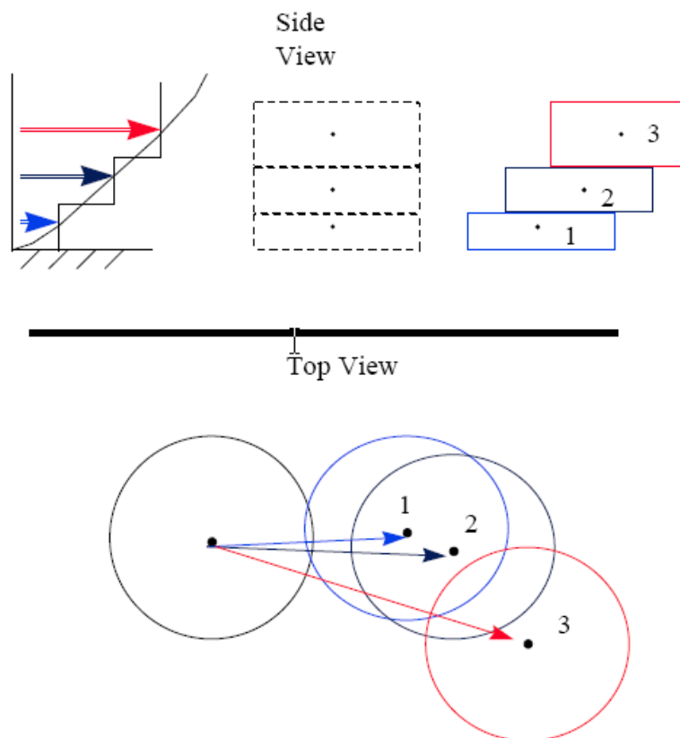
Figura 13 - Schema di funzionamento del modello CALPUFF
