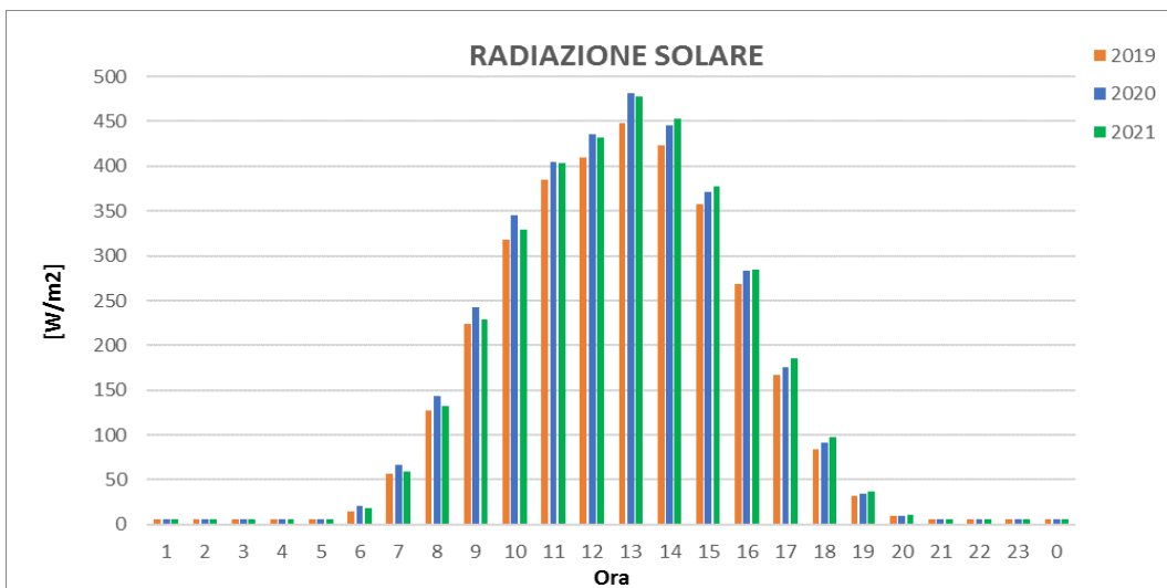
Figura 9 - Radiazione solare oraria nel triennio 2019 - 2021
