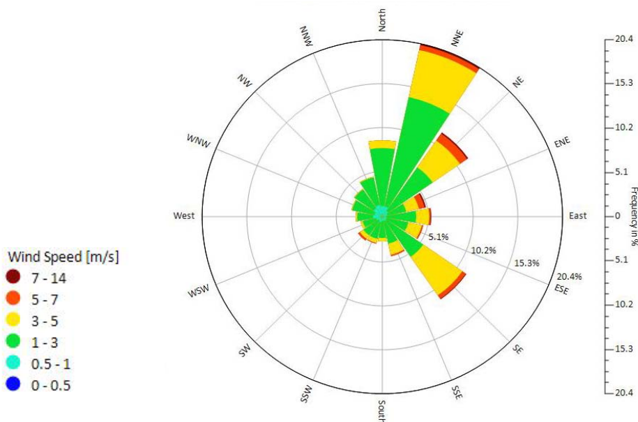
Figura 10 - Rosa dei venti stimata in corrispondenza dello stabilimento Versalis per l'anno 2021 - quota 10 m
