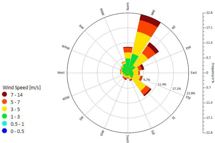
Figura 11 - Rosa dei venti stimata in corrispondenza dello stabilimento Versalis per l'anno 2021 - quota 100 m
