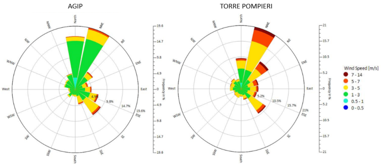
Figura 2 - Rose dei venti per l'anno 2019
