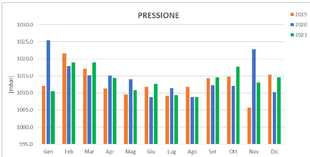
Figura 8 - Andamento della pressione atmosferica media mensile nel triennio 2019 – 2021
