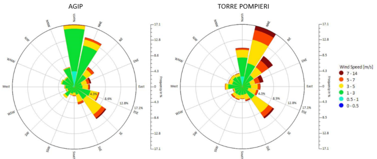
Figura 3 - Rose dei venti per l'anno 2020
