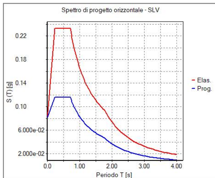
31_RIS_SPETTRI_PROGETTO_SLV_O.
