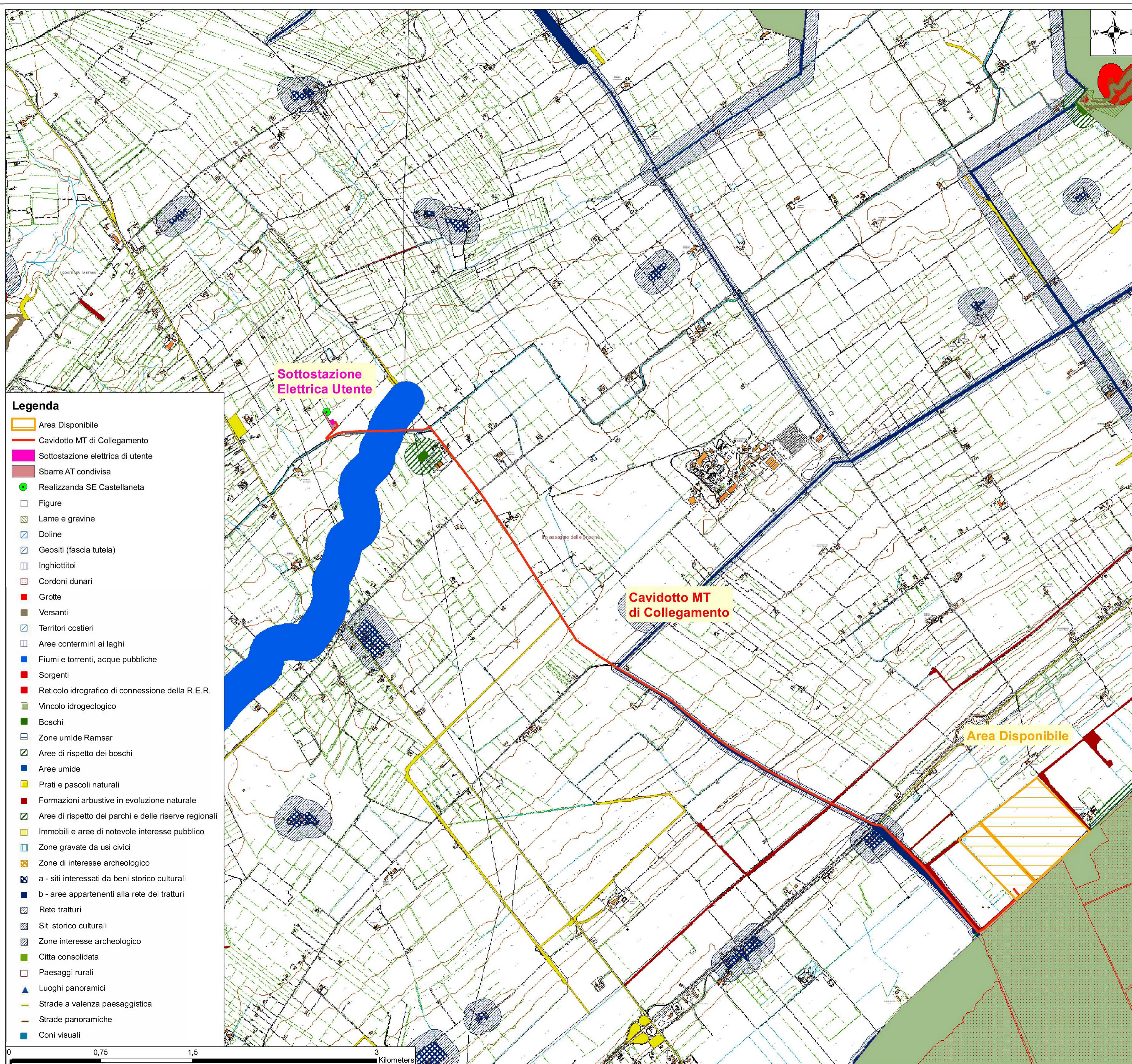
INQUADRAMENTO TERRITORIALE - COROGRAFIA SU CTR - SCALA 1:15.000
