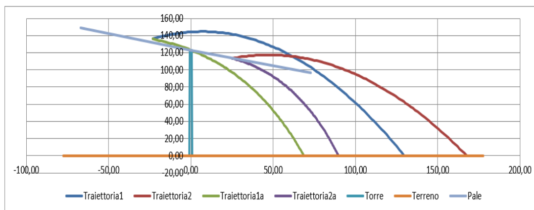
Figura 5 Calcolo della gittata mediante interpolazione dei valori assunti dall'angolo di lancio \alpha in WORST CASE
