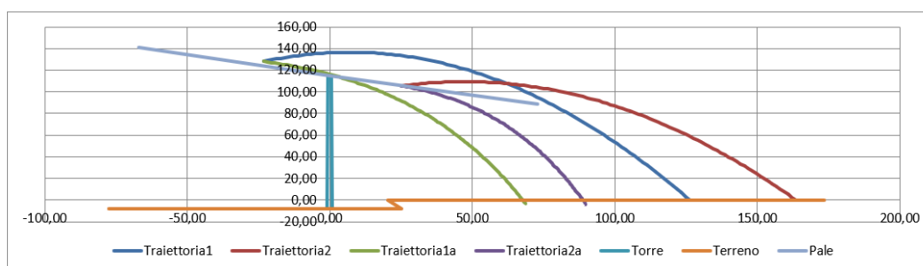
Figura 8 Calcolo della gittata mediante interpolazione dei diversi valori assunti dall'angolo di lancio \alpha in REAL CASE considerando un dislivello in posizione sopraelevata del ricevitore rispetto all'aerogeneratore e la presenza di attrito viscoso dovuto all'aria
