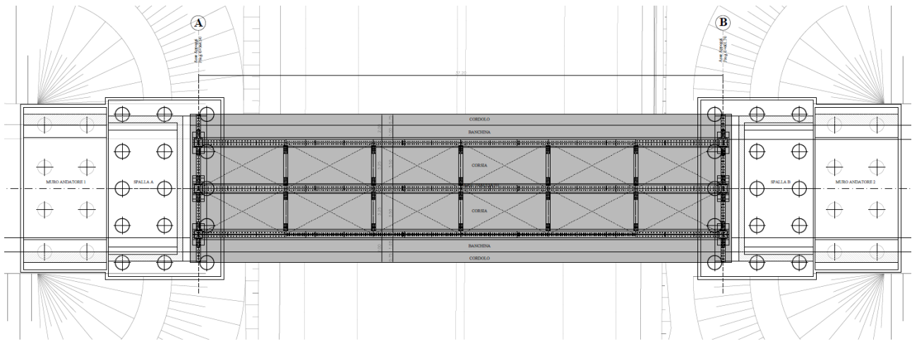
Pianta impalcato cavalcavia
