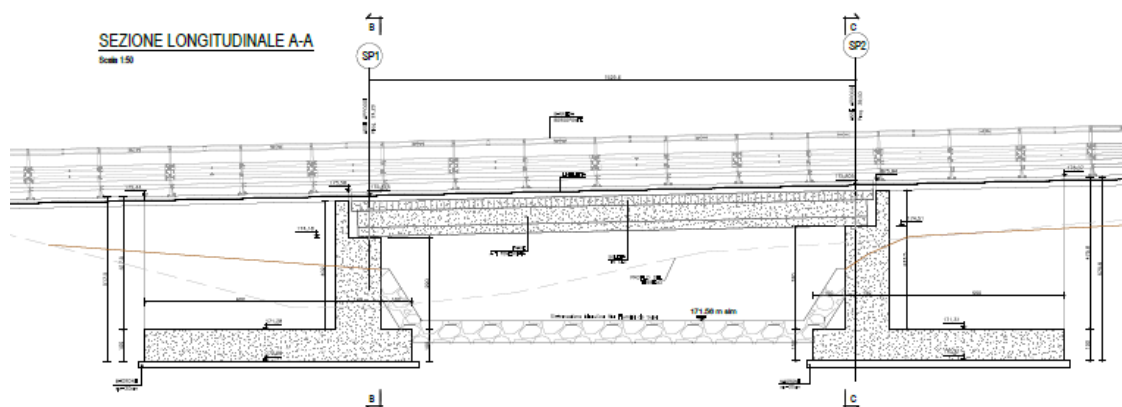
Profilo longitudinale
