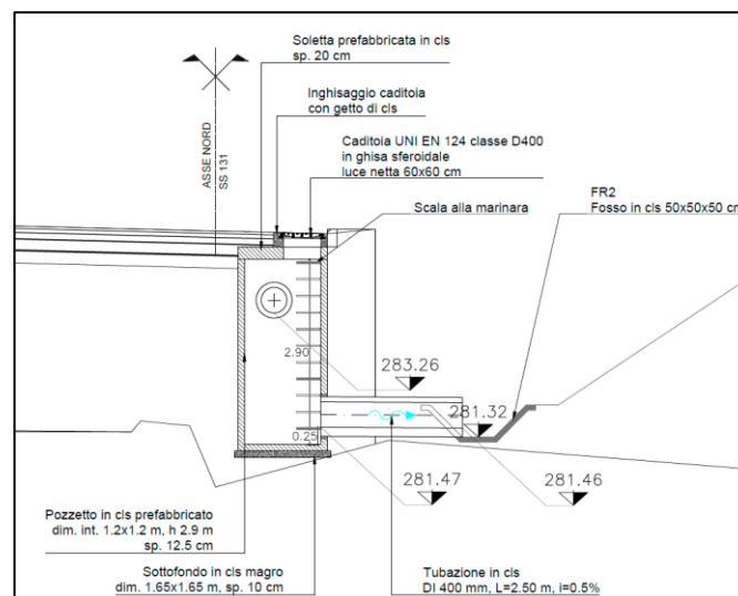
Particolare della sezione in rilevato con muro di sottoscarpa con drenaggio per mezzo di un sistema costituito da griglie e collettori sottostanti
