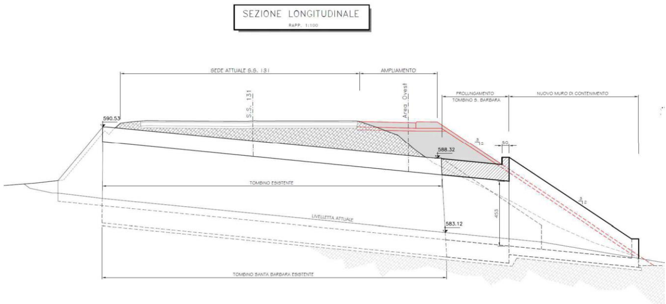
Profilo longitudinale
