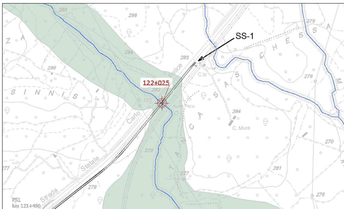
Figura 2 - PSFF intervento a progr km 122+025
