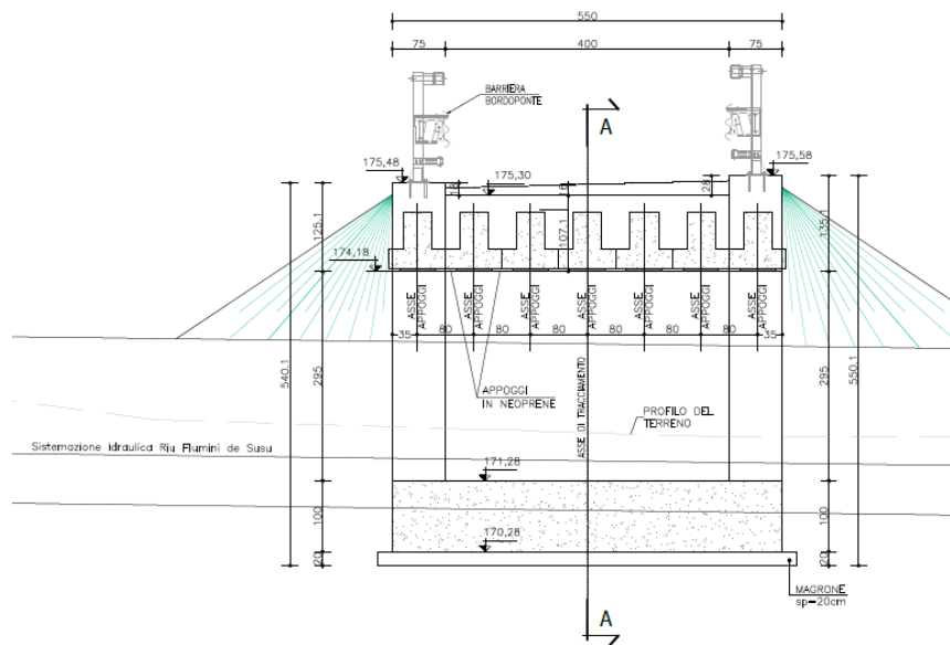
Sezione trasversale corrente
