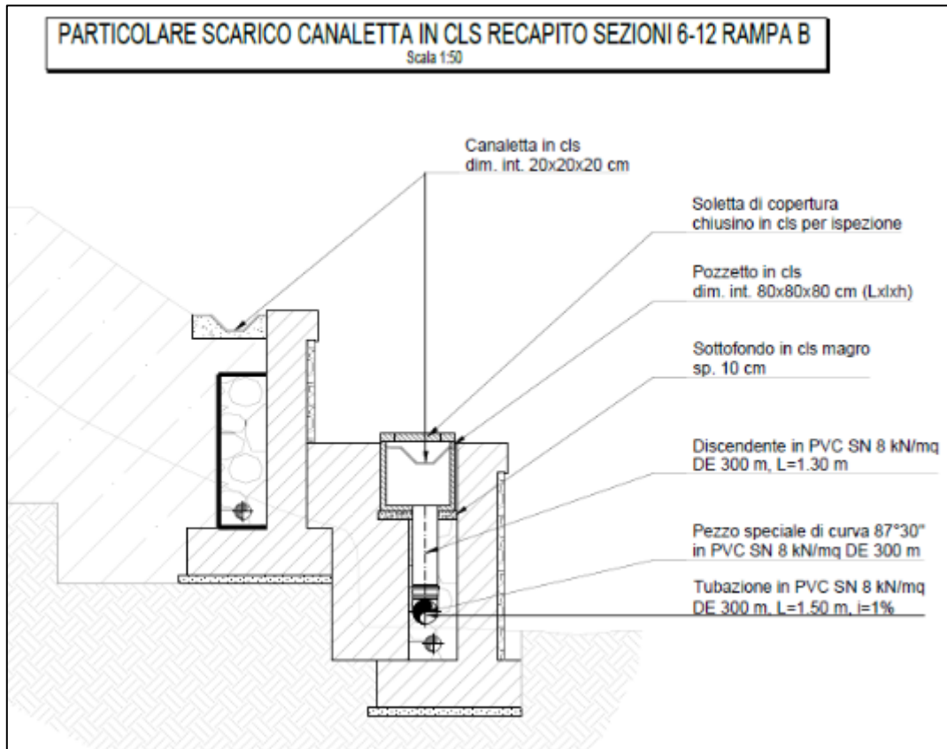
Figura 158 – Particolare dello scarico della canaletta trapezia in cls di dimensioni 20x20x20 cm in fosso esistente a tergo del muro di sottoscarpa
