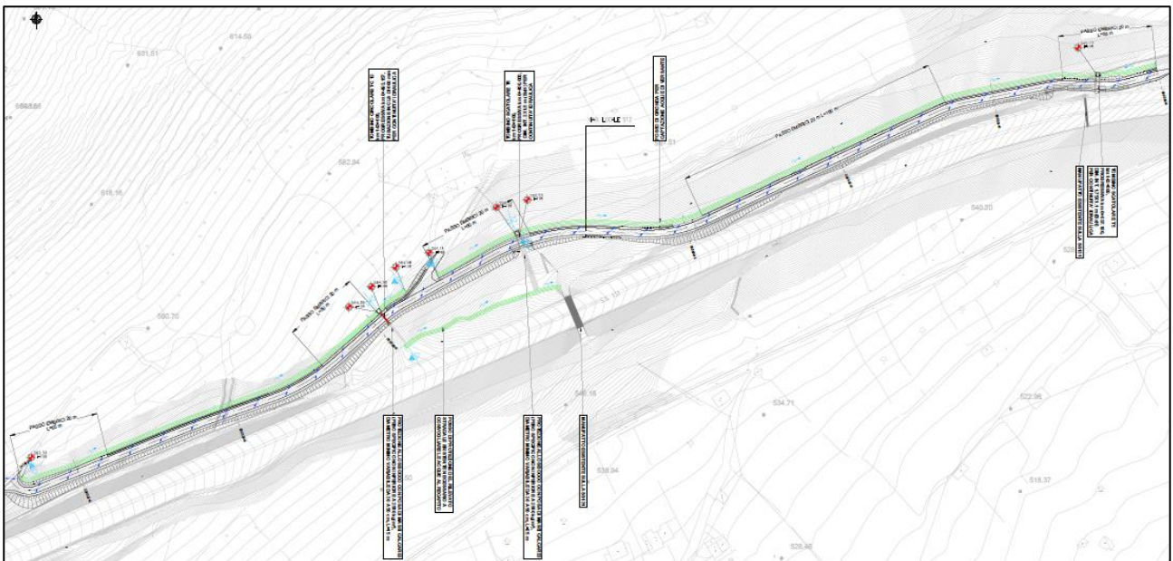
Figura 183 - Stralcio planimetrico intervento S12-Risoluzione accesso C.N. dal km 143+215 al km 143+900
