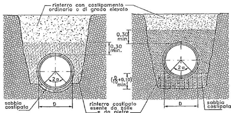
Figura 298 - Tipologia di posa "tipo B"
