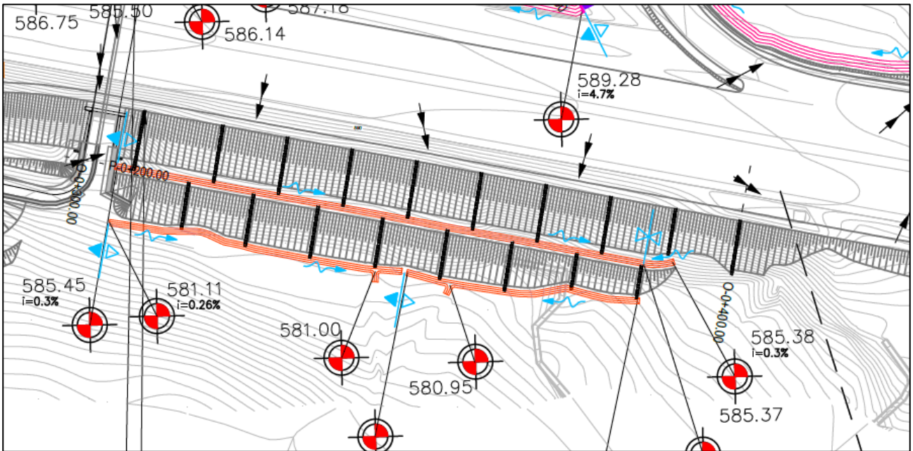
Figura 276 – Disposizione degli embrici lungo la banchettatura, svincolo dell'Area Archeologica di S. Barbara
