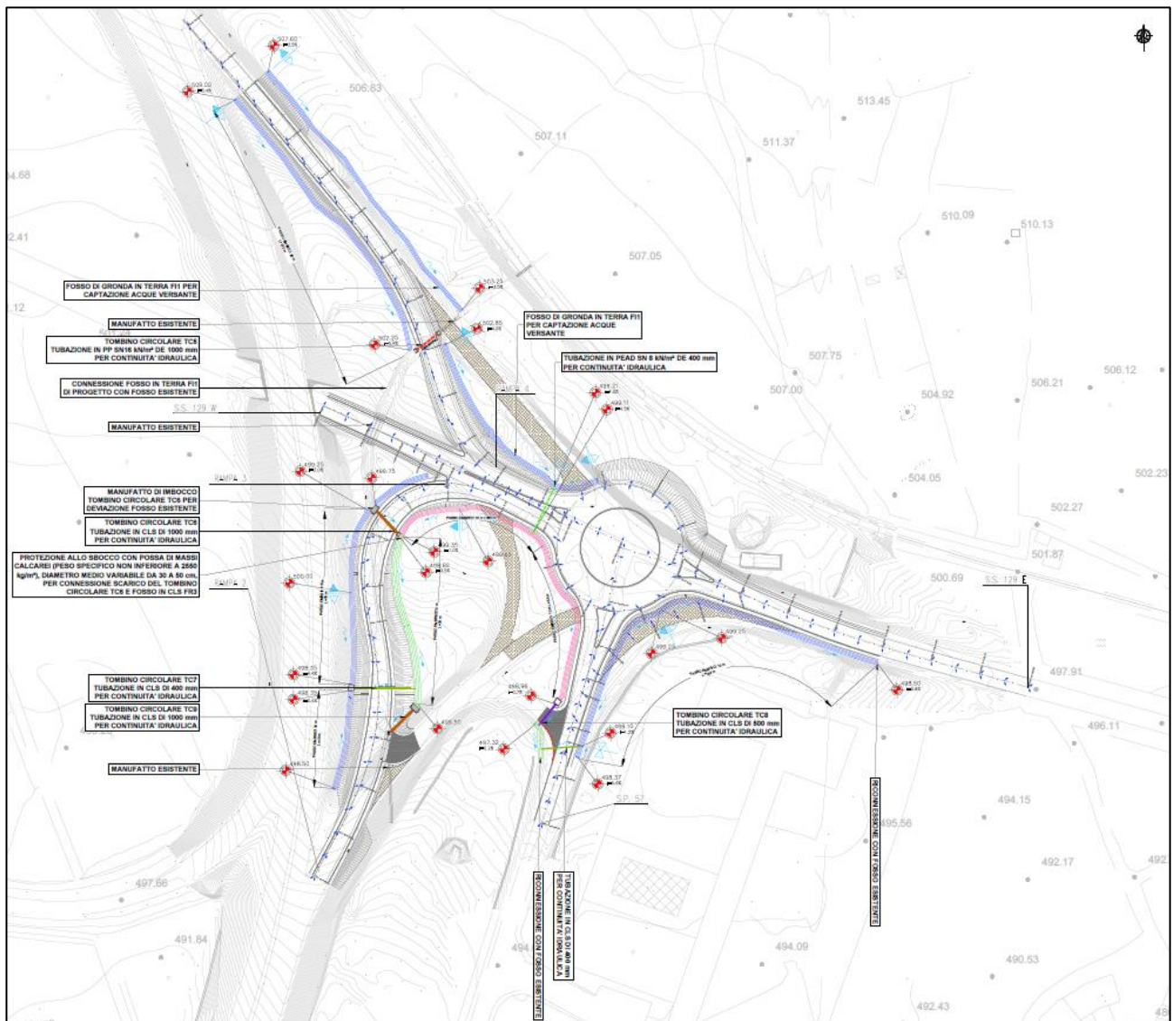
Figura 264- Stralcio planimetrico intervento V09-Svincolo di Macomer al km 142+500
