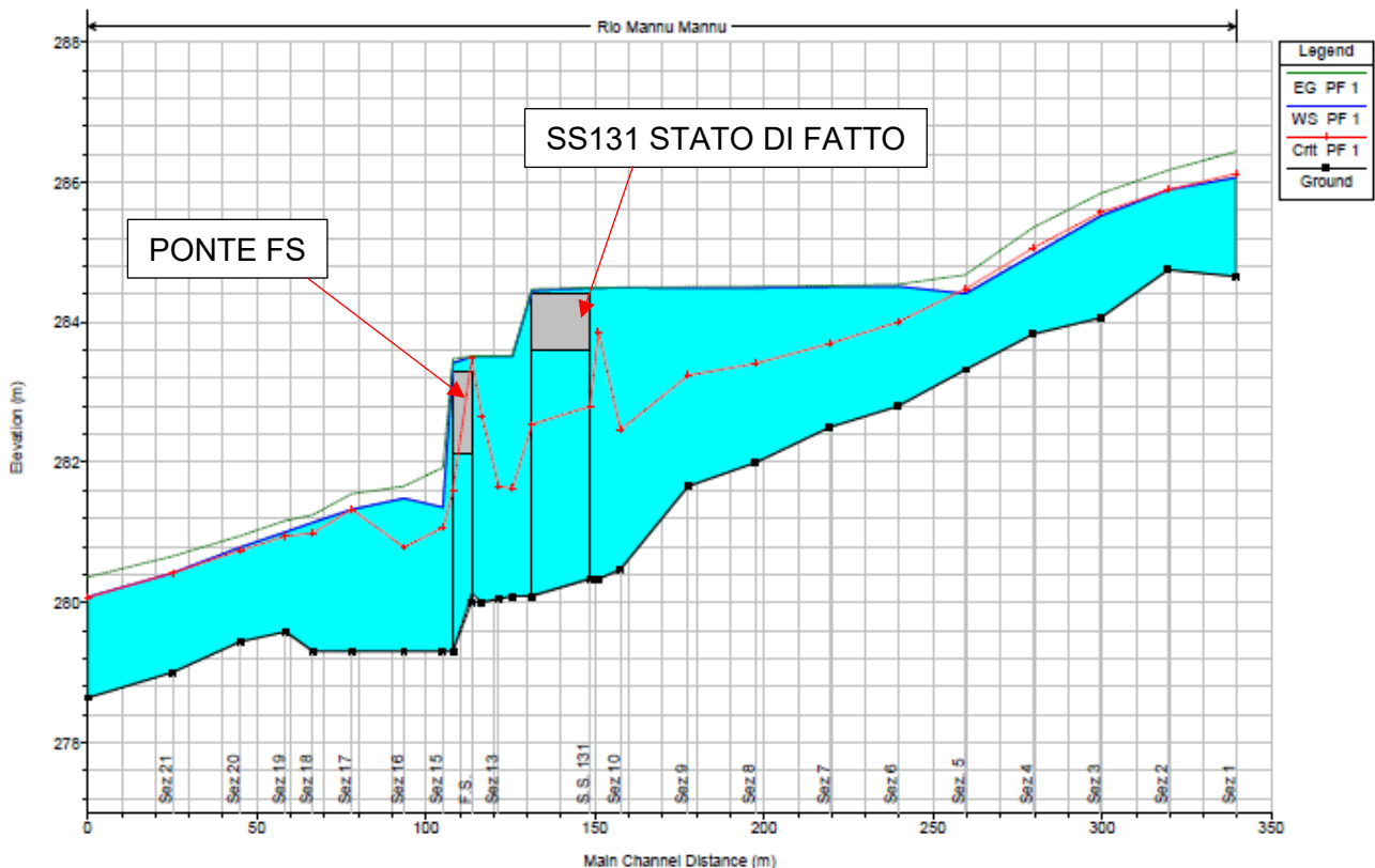
Figura 23 – Profilo longitudinale stato di fatto (Q TR 200 anni)
