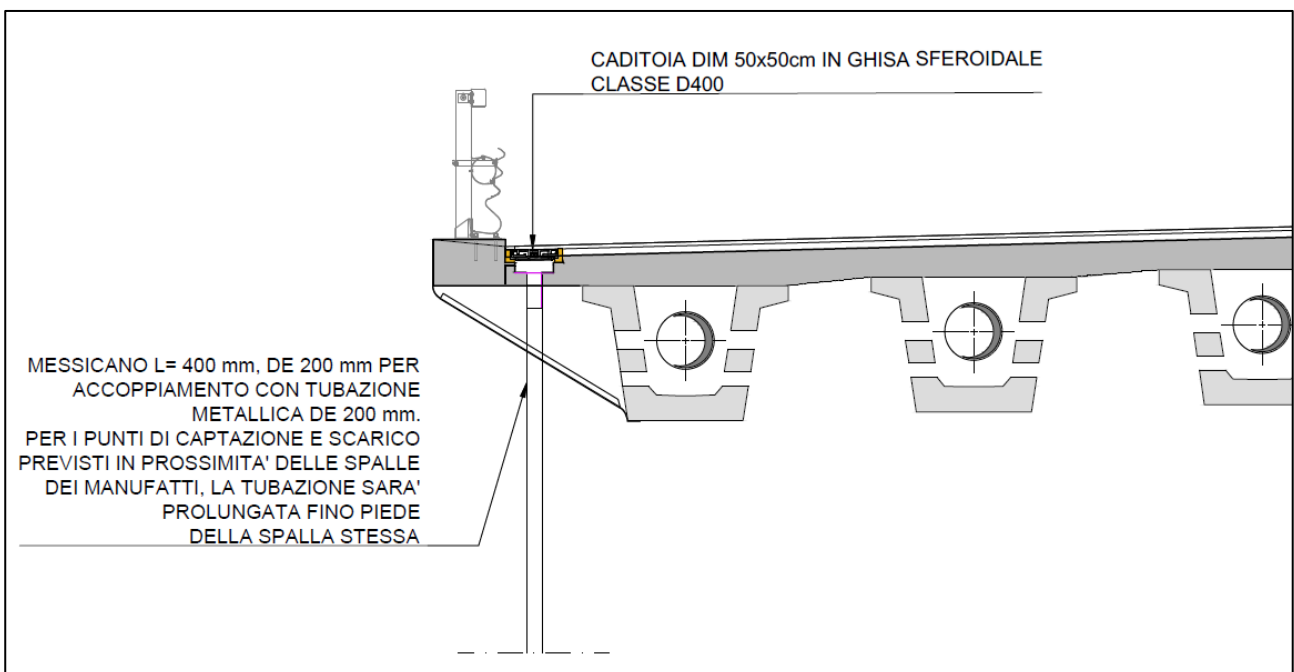
Figura 165 – Particolare tipologico di captazione delle acque meteoriche e sezione tipo di scarico nel collettore principale in viadotto
