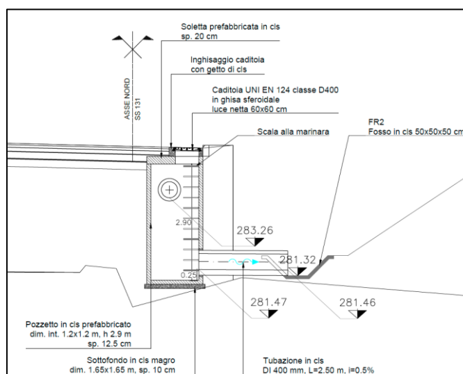
Figura 156 – Particolare della sezione in rilevato con muro di sottoscarpa con drenaggio per mezzo di un sistema costituito da griglie e collettori sottostanti
