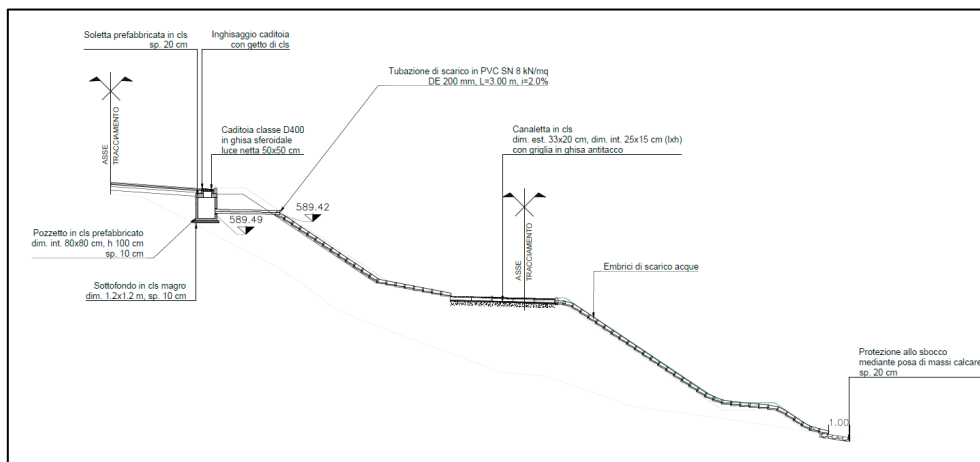
Figura 275 – Particolare della captazione lungo il percorso pedonale dello svincolo di S. Barbara
