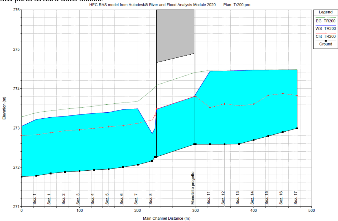
Figura 106 - Profilo longitudinale stato di progetto (Q TR 200 anni)
