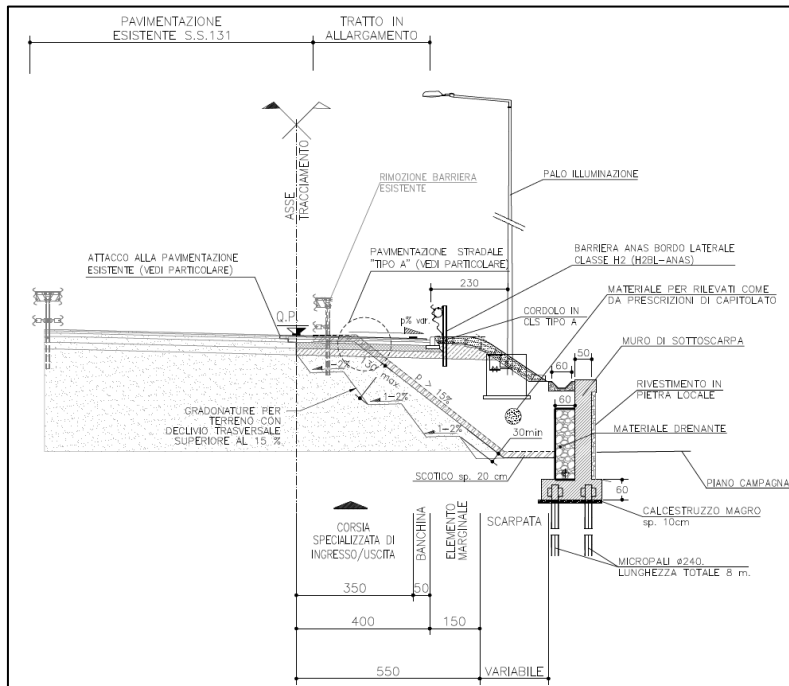
Figura 157 – Sezione tipo in rilevato in presenza di muro di sottoscarpa. Il sistema di drenaggio prevede l'adozione di embrici e di una canaletta trapezia in cls di dimensioni 20x20x20 cm
