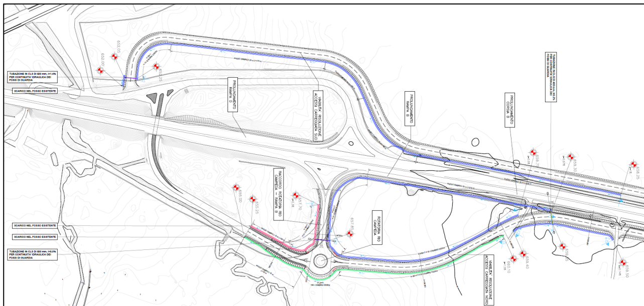
Figura 288 - Stralcio planimetrico intervento V11-Svincolo Campeda al km 152
