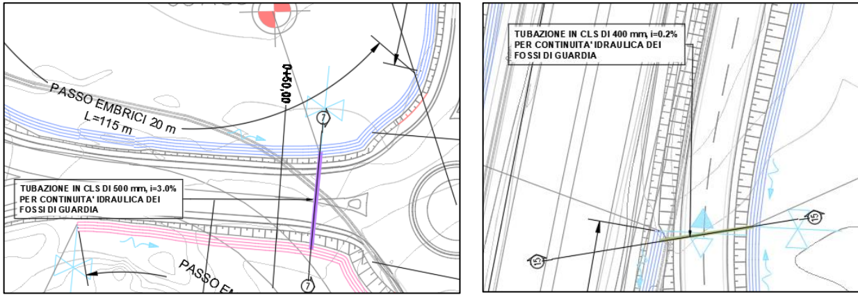
Figura 292 – Stralcio planimetrico con ubicazione degli attraversamenti previsti in progetto
