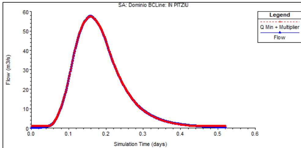
Figura 116 – Idrogramma Riu Pitziu
