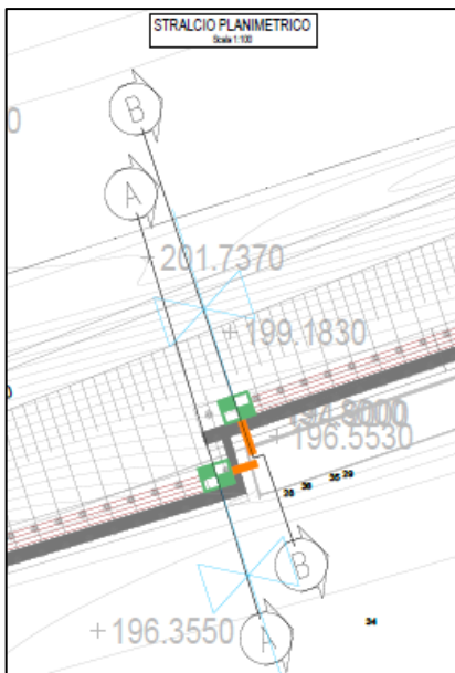
Figura 247 – Particolare dello scarico della canaletta trapezia in cls di dimensioni 20x20x20 cm in fosso esistente a tergo del muro di sottoscarpa
