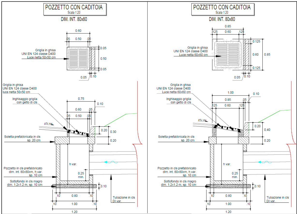
Figura 162 – Particolare dello scarico con griglia e pozzetto sottostante in cls in corrispondenza della cunetta alla francese. Le acque vengono coltettate da tubazioni in cls o PEad DE variabile al di sotto della cunetta
