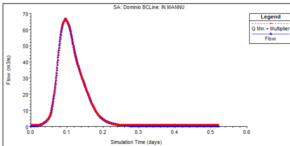
Figura 117 – Idrogramma Riu Mannu
