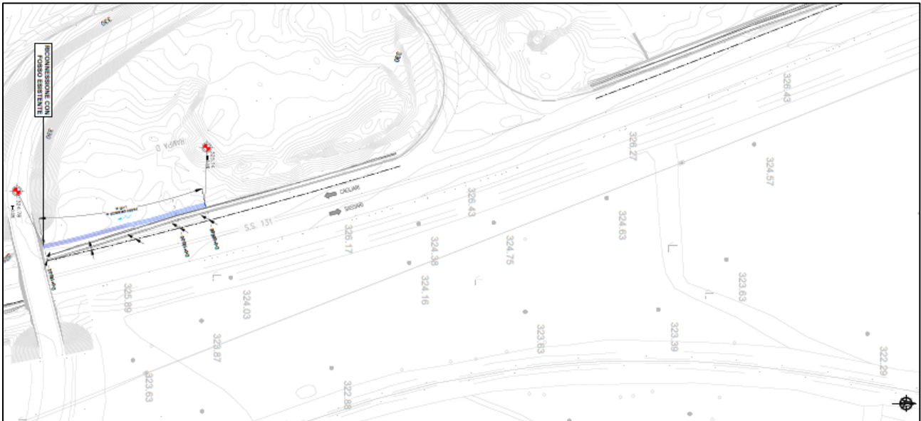
Figura 262-Stralcio planimetrico intervento V07-Svincolo di Norbello al km 128+000
