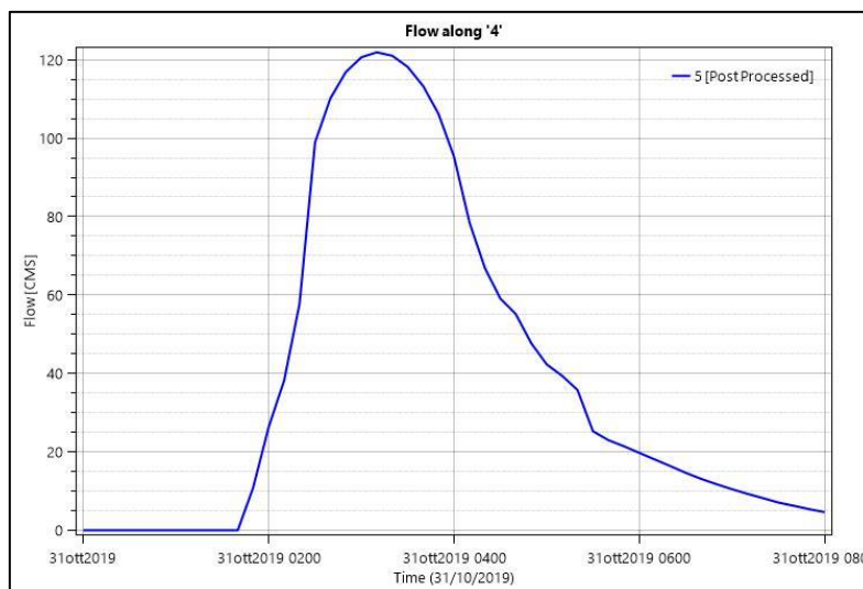
Figura 123 – Idrogramma in corrispondenza dell'attraversamento sul Riu Temo
