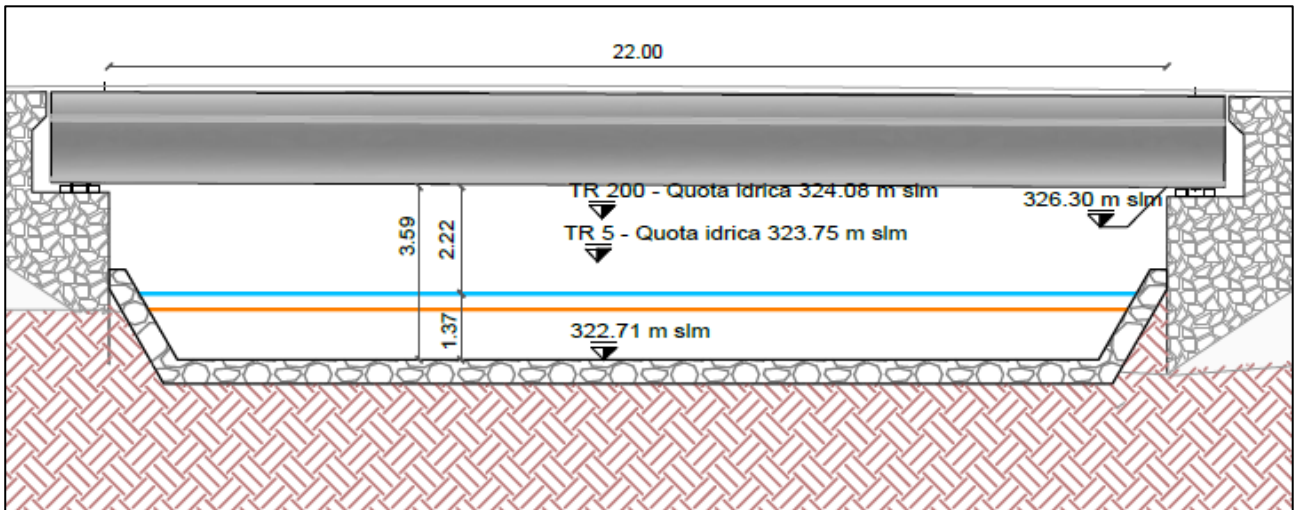
Figura 70 – Verifica compatibilità NTC2008 manufatto di progetto (TR 200 anni) complanare B
