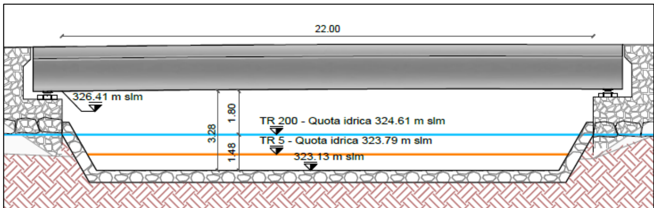
Figura 69 – Verifica compatibilità NTC2008 manufatto di progetto (TR 200 anni)
