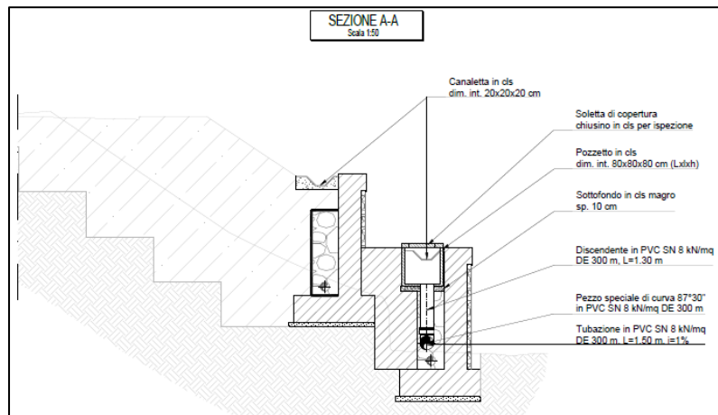
Figura 246 – Sezione tipo in rilevato in presenza di muro di sottoscarpa. Il sistema di drenaggio prevede l'adozione di embrici e di una canaletta trapezia in cls di dimensioni 20x20x20 cm
