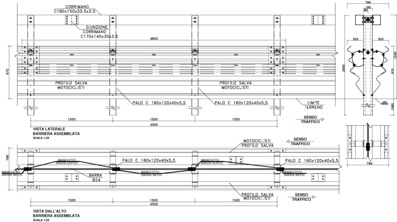
Vista laterale e dall'alto barriera ANAS H4 ST DSM
