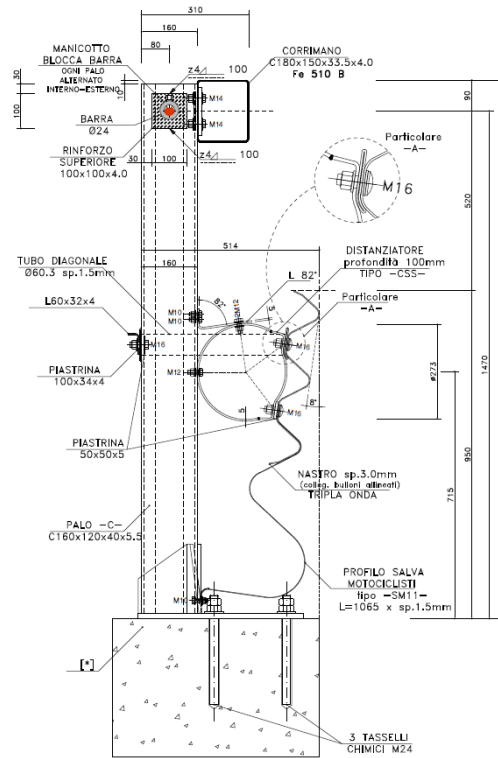
Sezione barriera ANAS H4 BPSM
