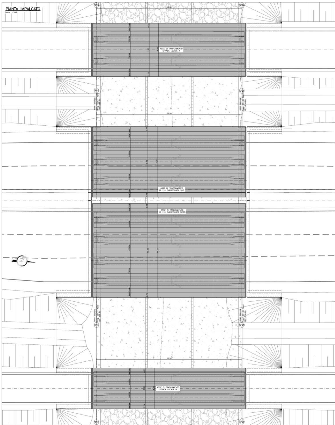
Pianta impalcato
