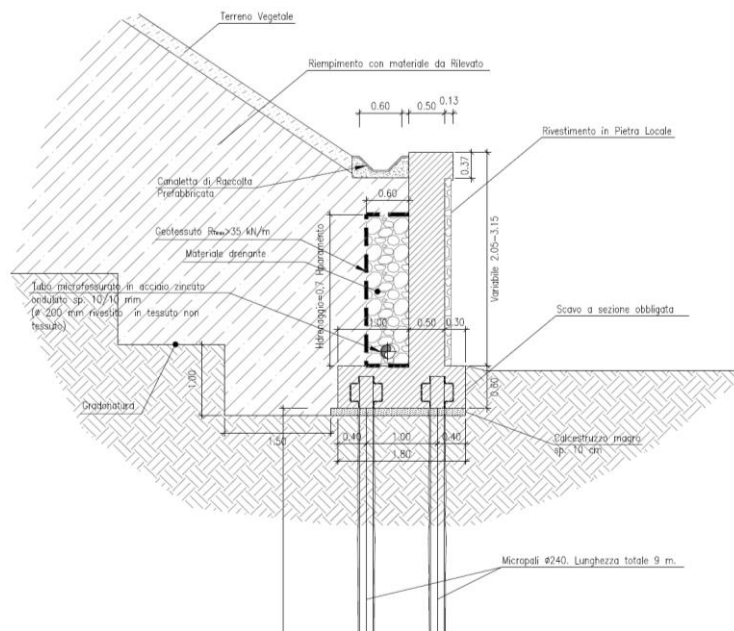
Sezione tipo Muro V03-OS01
