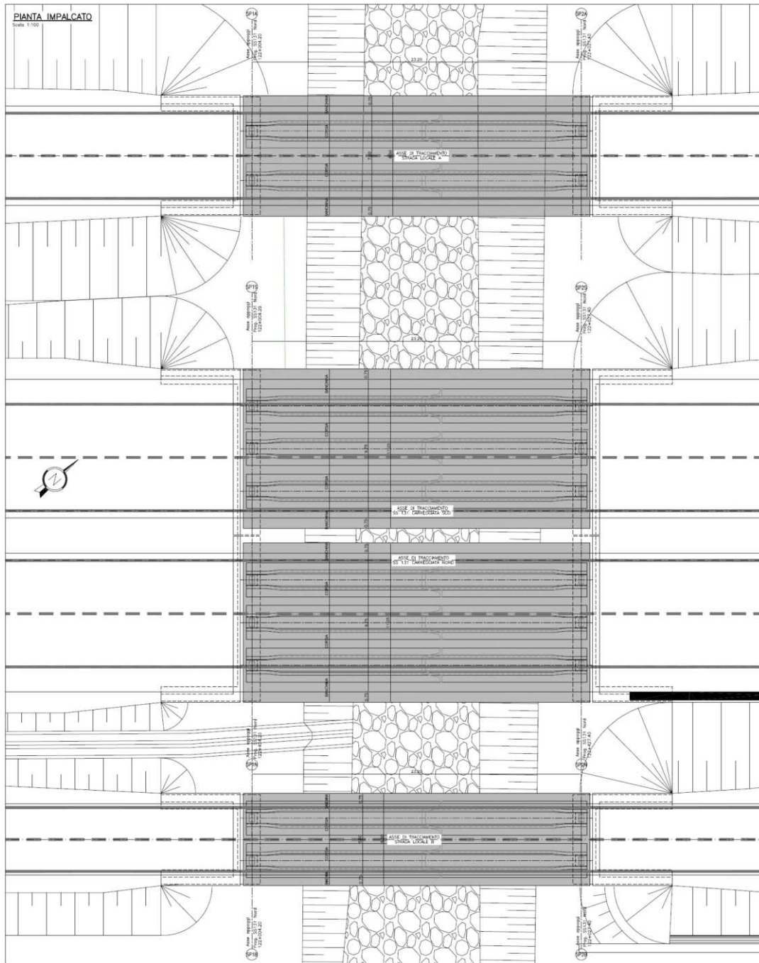
Pianta impalcato
