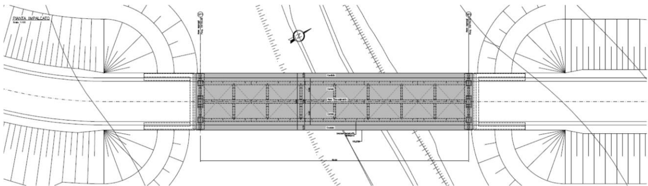
Pianta impalcato
