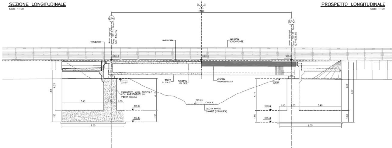
Profilo longitudinale
