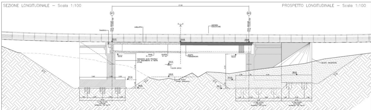
Profilo longitudinale
