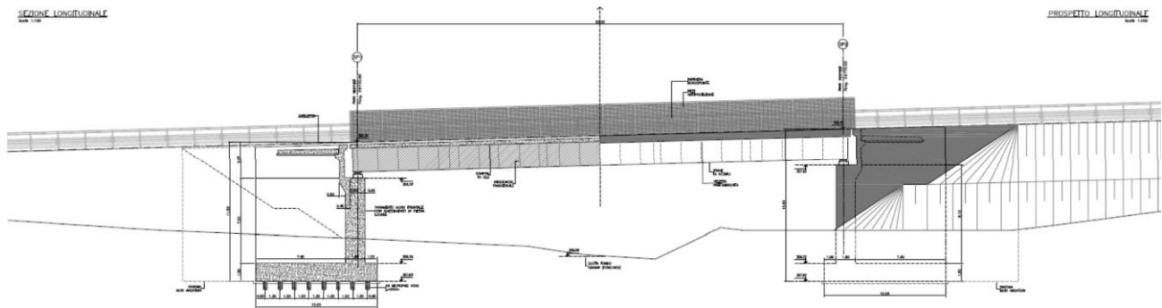
Profilo longitudinale
