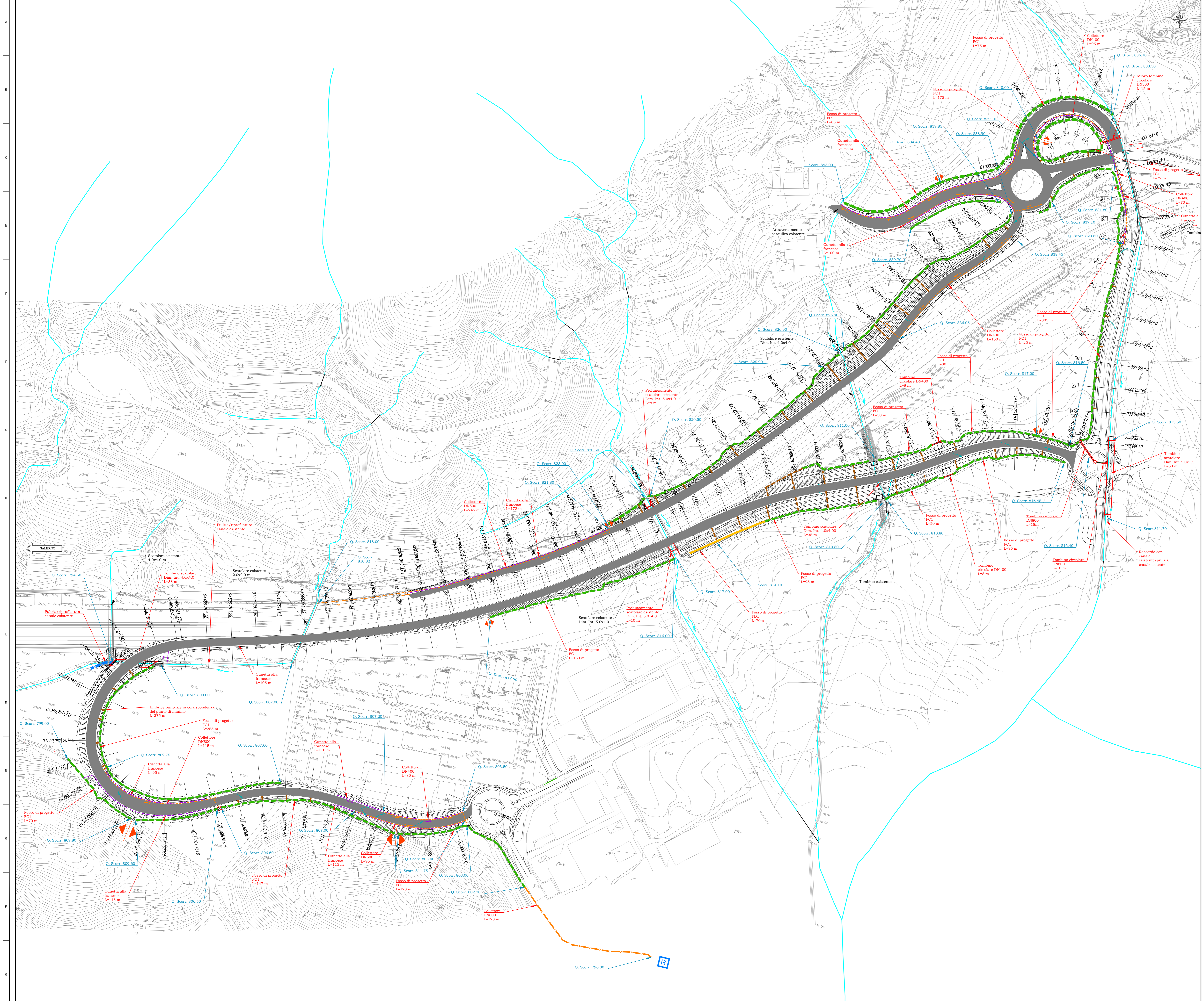
Tavola 1/2 - Svincolo sud
