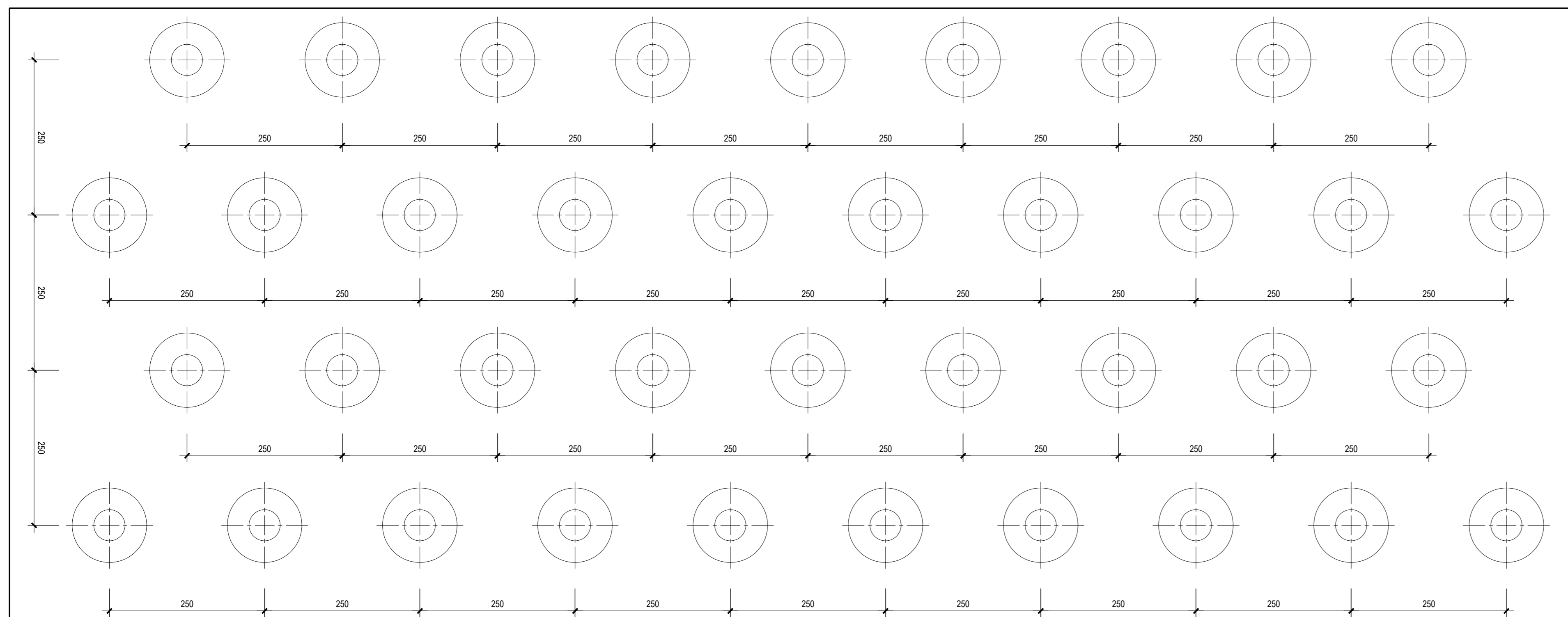
PIANTA -Scala 1:50
