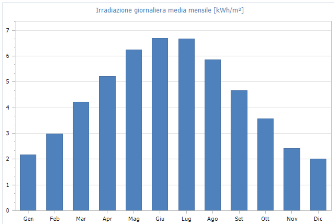
Fig. 1: Irradiazione giornaliera media mensile sul piano orizzontale [kWh/m²]- Fonte dati: Enea - Località di riferimento: Santa Teresa di Riva (ME)
