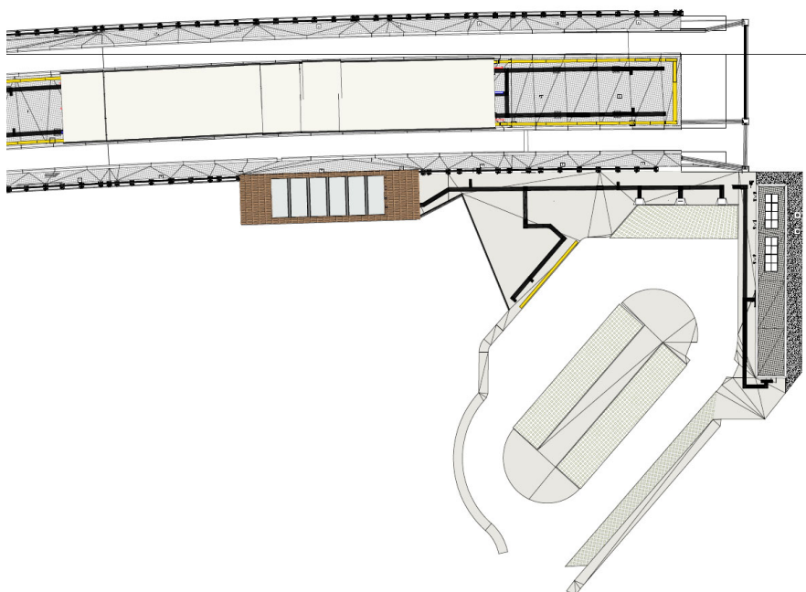
Planimetria inserimento campo fotovoltaico
