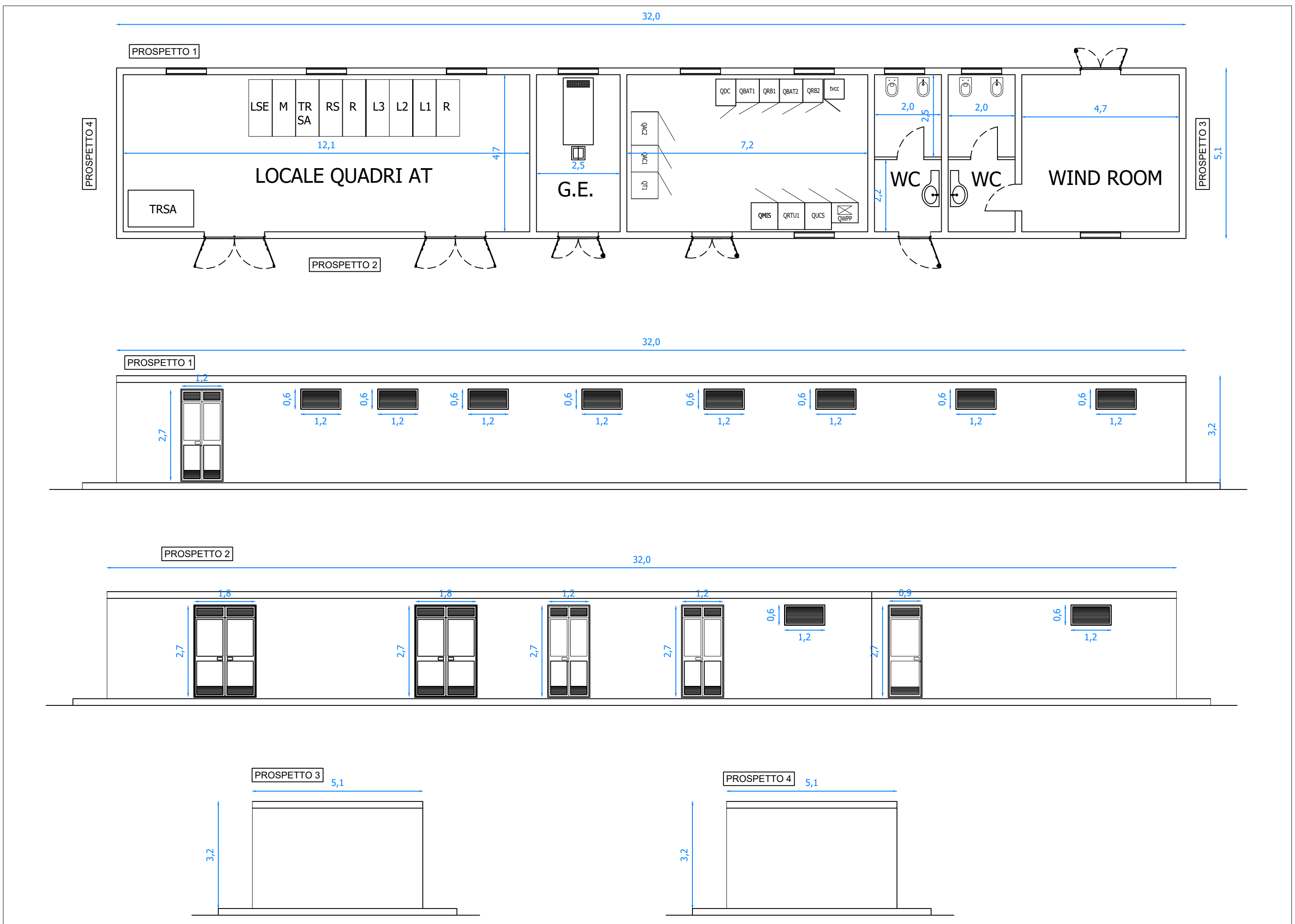
Prospetti fabbricato
