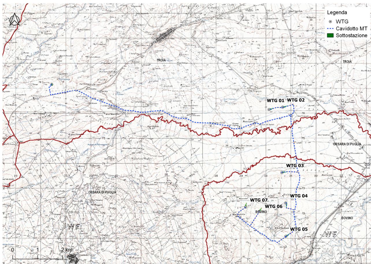
Figura 2 - Inquadramento impianto su Stralcio IGM 1:25.000
