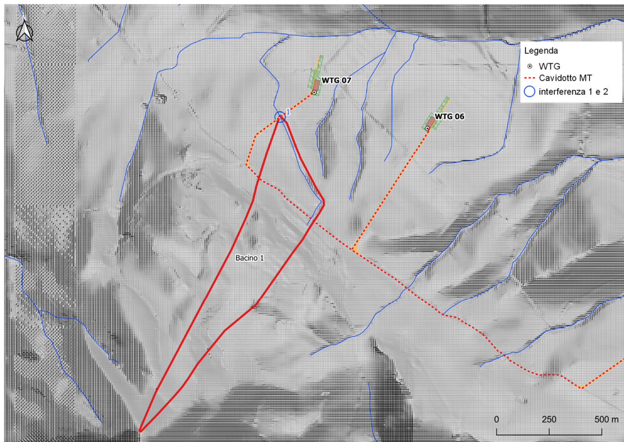
Figura 4 - Individuazione bacini idrologici su DTM (Digital Terrain Model)
