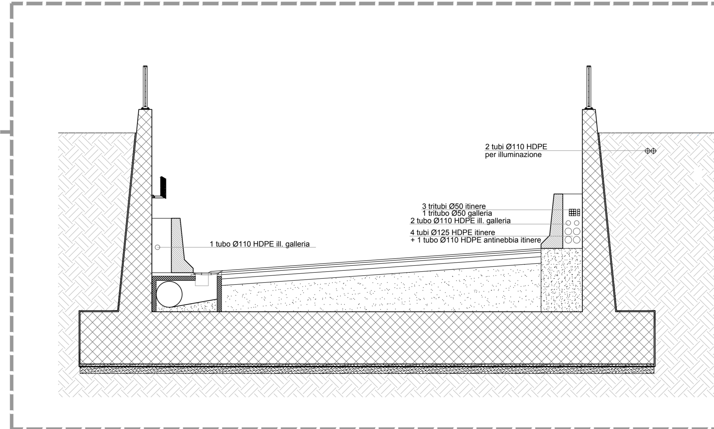
SEZIONE TIPO CAVIDOTTO PER TRATTI IN TRINCEA
