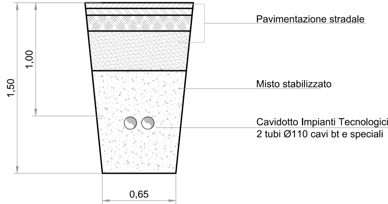
CAVIDOTTI IN SPARTITRAFFICO CENTRALE
