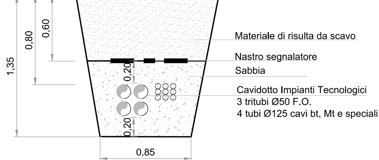
CAVIDOTTI ALLA BASE DEL RILEVATO - CARREGGIATA SUD
