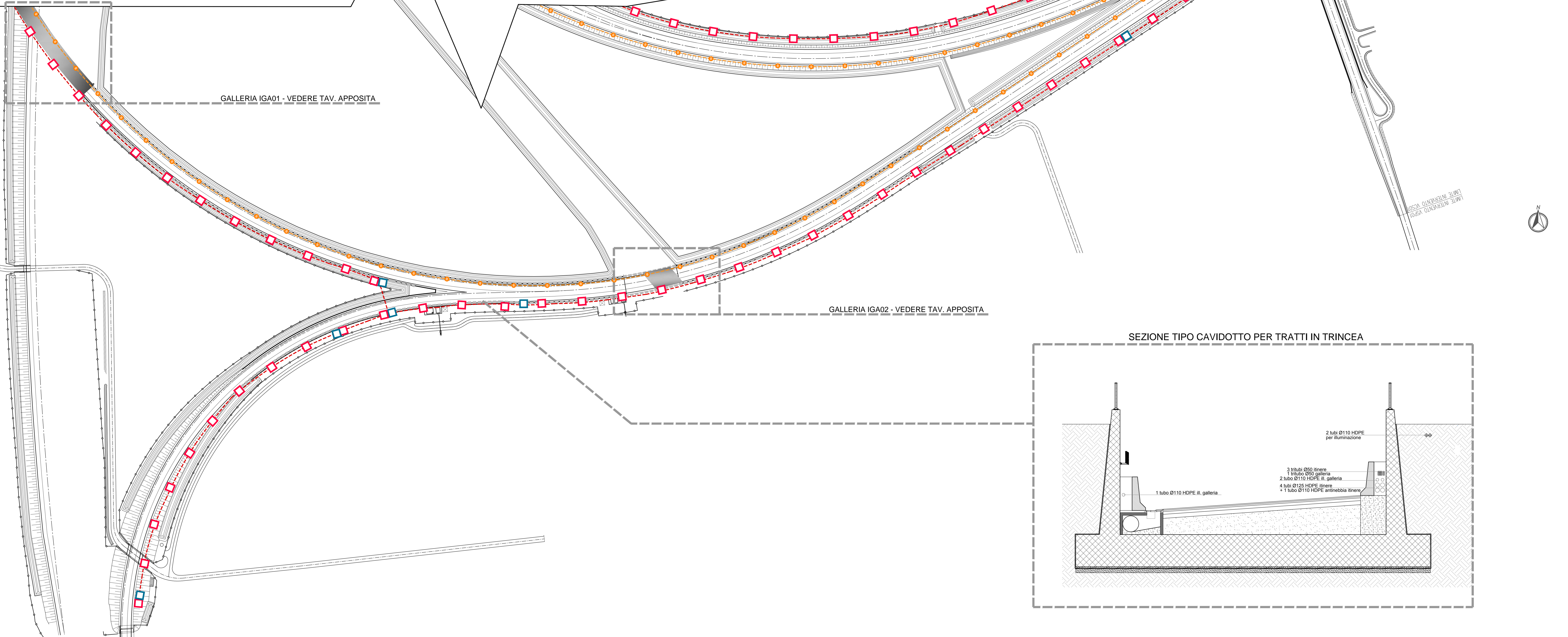
PLANIMETRIA CAVIDOTTI IN ITINERE SVINCOLO A22 - scala 1:1000
