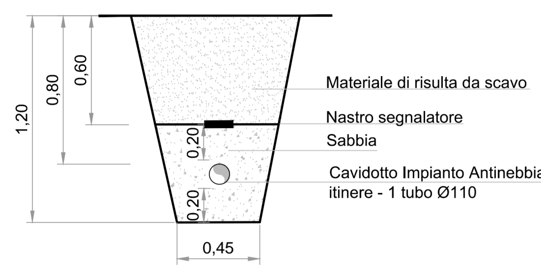
CAVIDOTTO ANTINEBBIA IN ITINERE IN RILEVATO - LATO DESTRO
