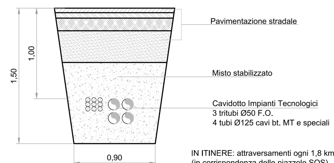
ATTRAVERSAMENTI CORPO AUTOSTRADALE
