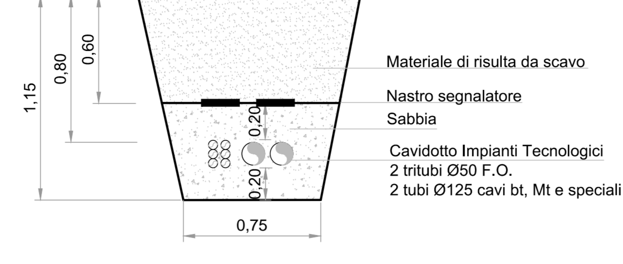
CAVIDOTTI ALLA BASE DEL RILEVATO - CAREGGIATA NORD
