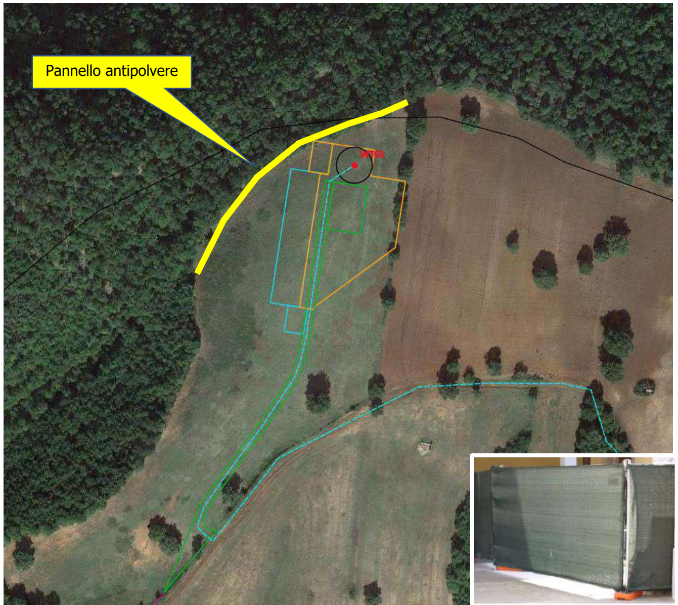
Figura 5-1: Esempio di posizionamento barriera antipolvere
