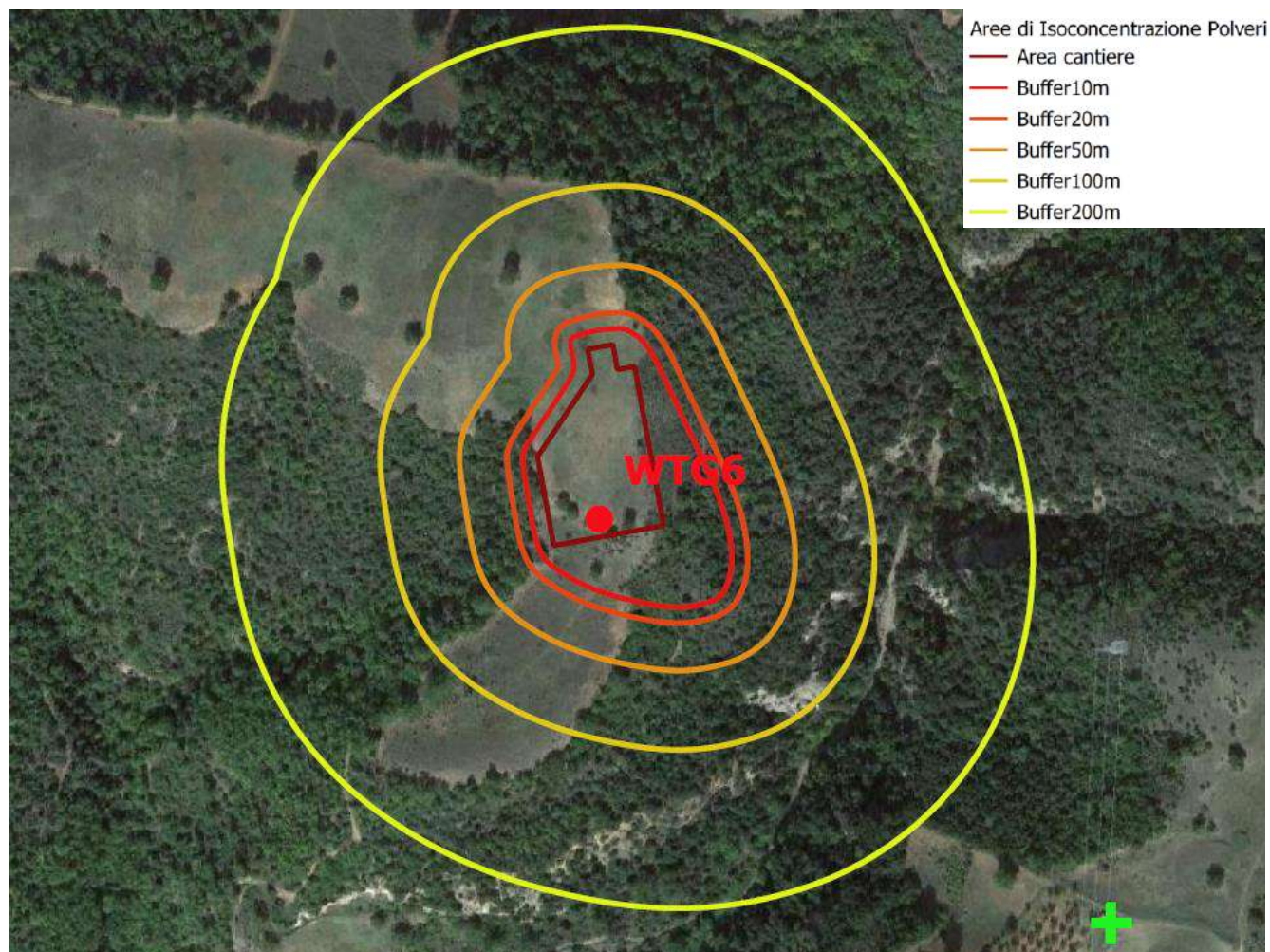
Figura 4-65: Aree Isoconcentriche nell'area di cantiere della turbina WTG06
