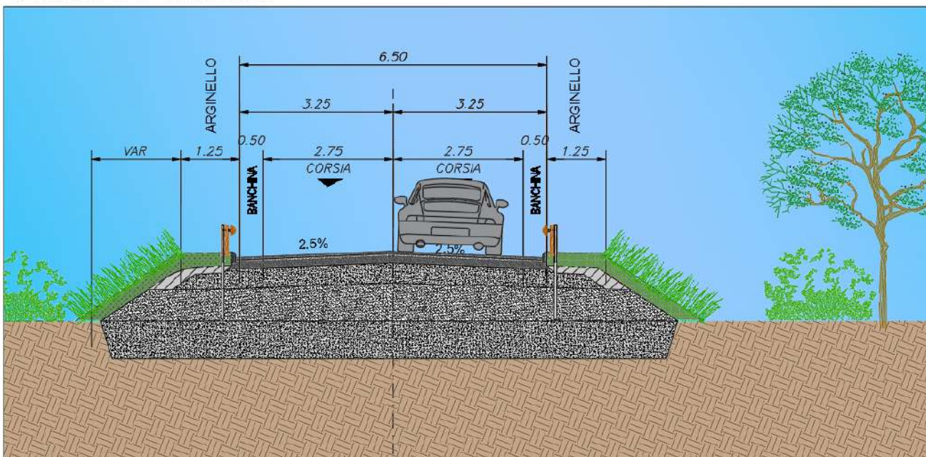
Figura 4-30: Sezione Tipo F in rilevato
