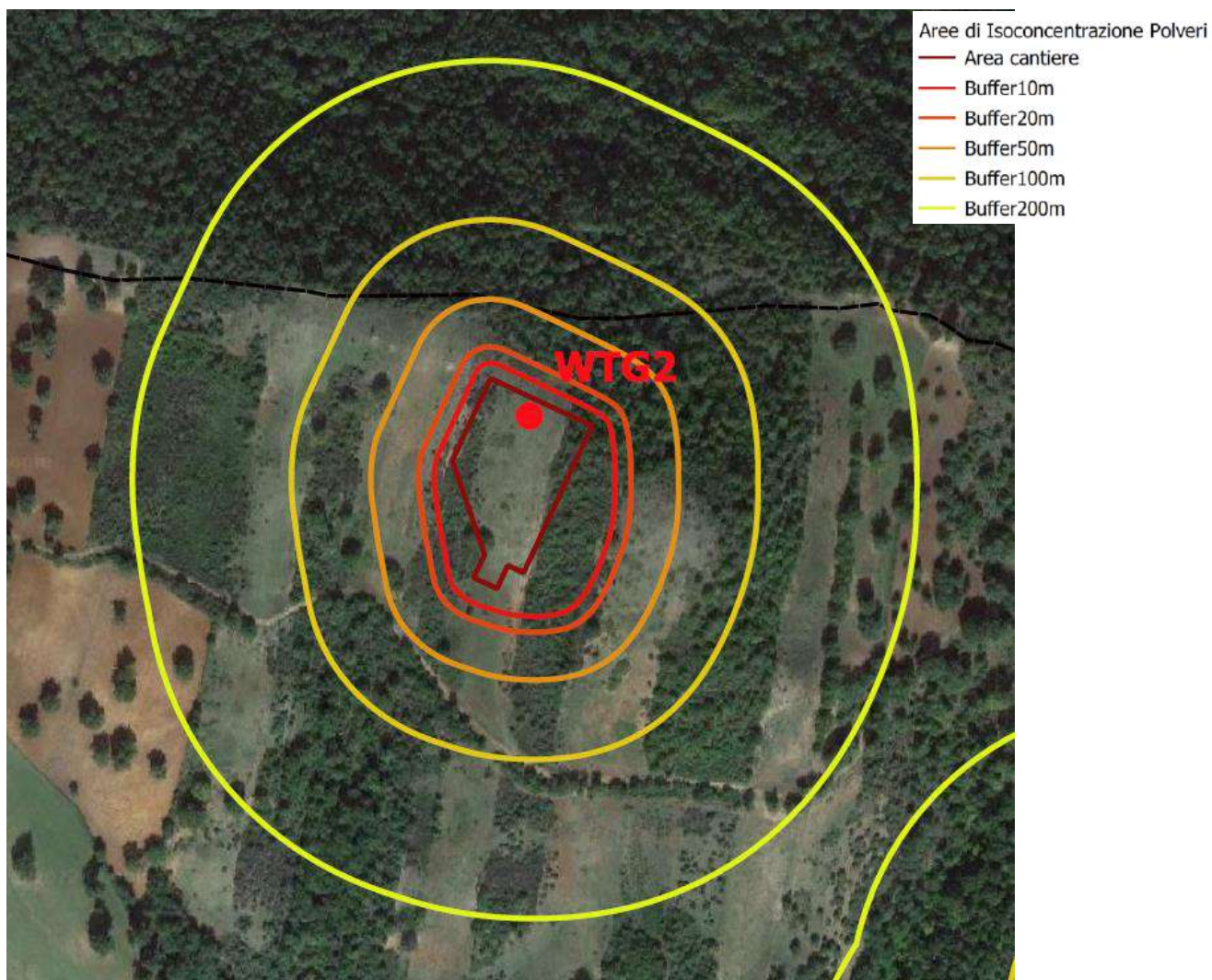
Figura 4-61: Aree Isoconcentriche nell'area di cantiere della turbina WTG02
