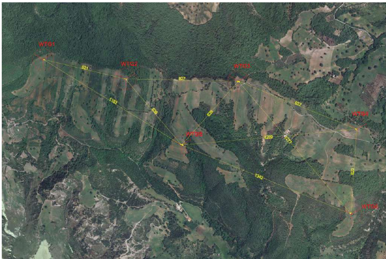
Figura 4-72: Estratto tavola A.16.b.1.2 Planimetria con distanze aerogeneratori
