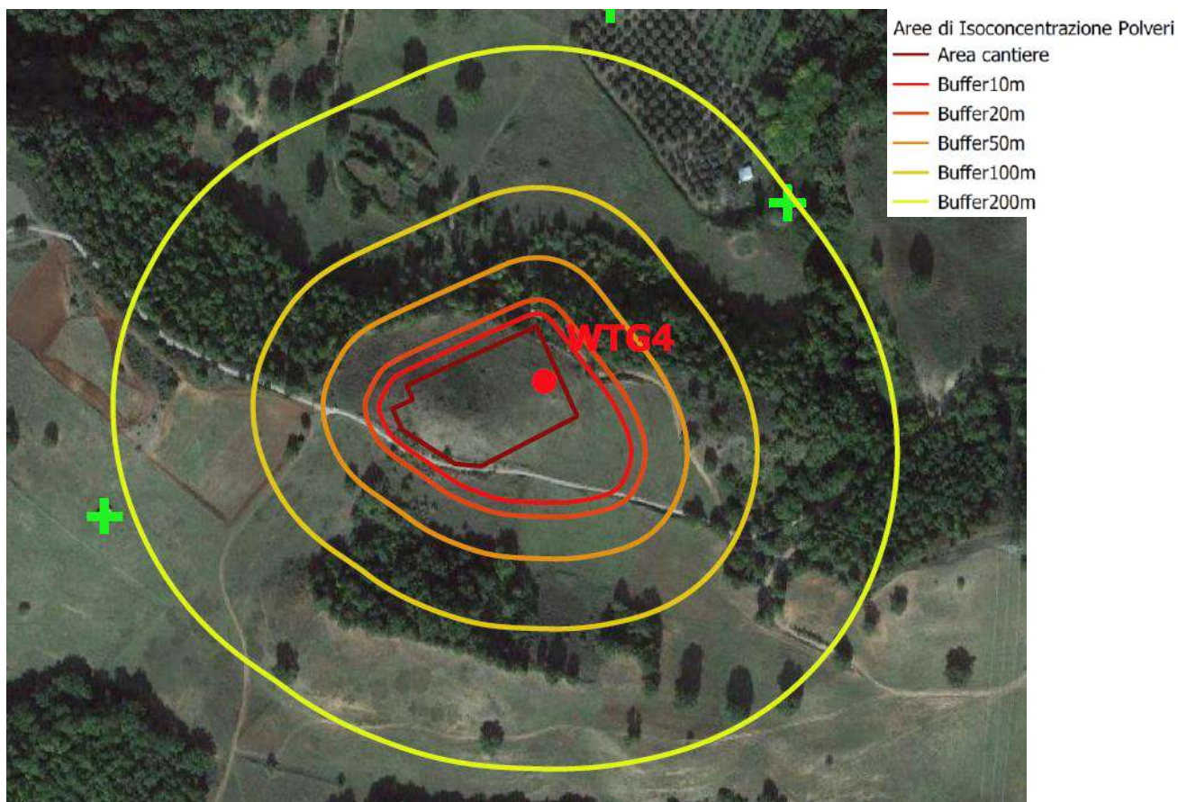
Figura 4-63: Aree Isoconcentriche nell'area di cantiere della turbina WTG04
