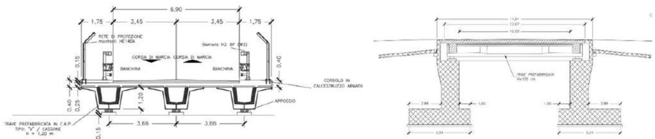
Figura 4-35: Sezioni Tipo Ponte 1
