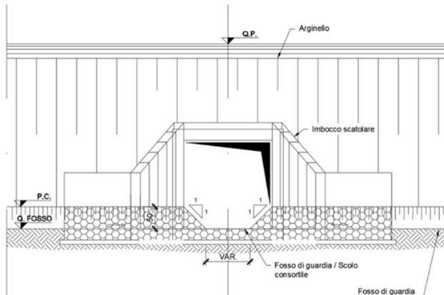
Figura 4-37: Sezioni Tipo Tombino Scatolare
