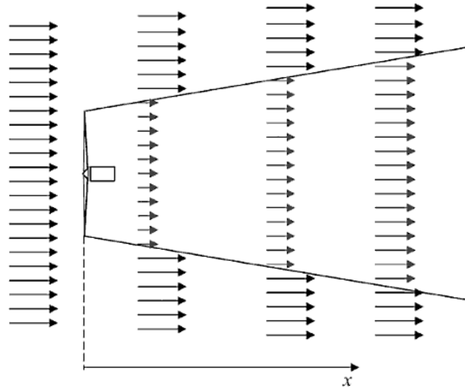
Figura 4-71: Andamento della scia provocata dalla presenza di un aerogeneratore. [Caffarelli-De Simone Principi di progettazione di impianti eolici Maggioli Editore]
