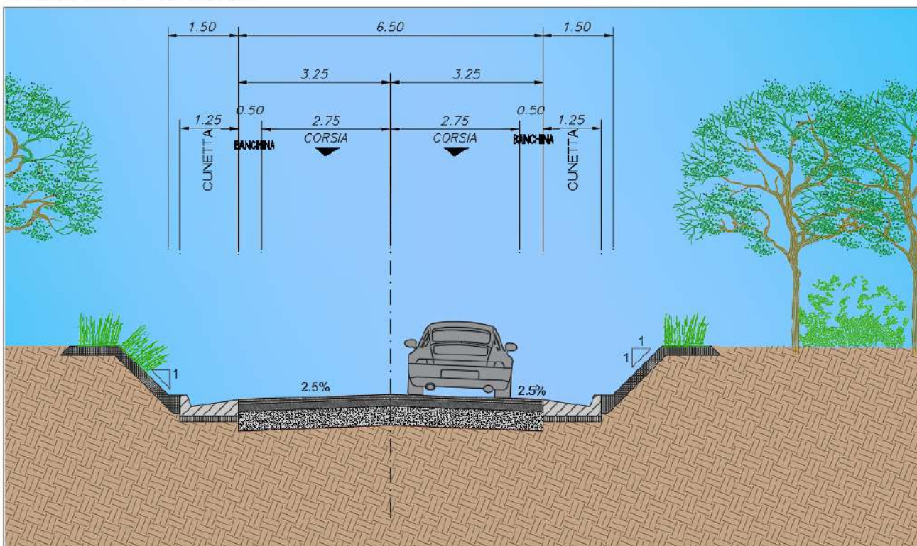
Figura 4-31: Sezione Tipo F in trincea
