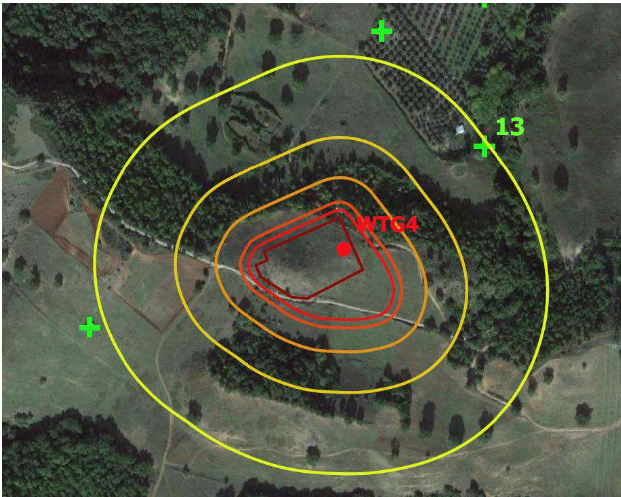
Figura 4-82: Aree di Isoconcentrazione e Ricettori – WTG 04
