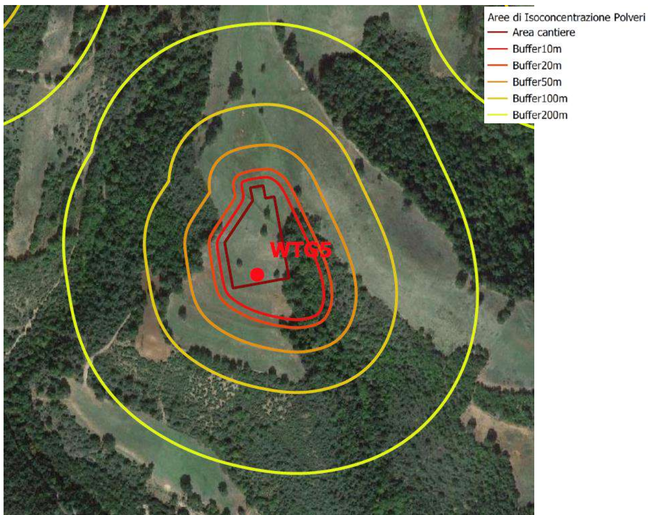
Figura 4-64: Aree Isoconcentriche nell'area di cantiere della turbina WTG05
