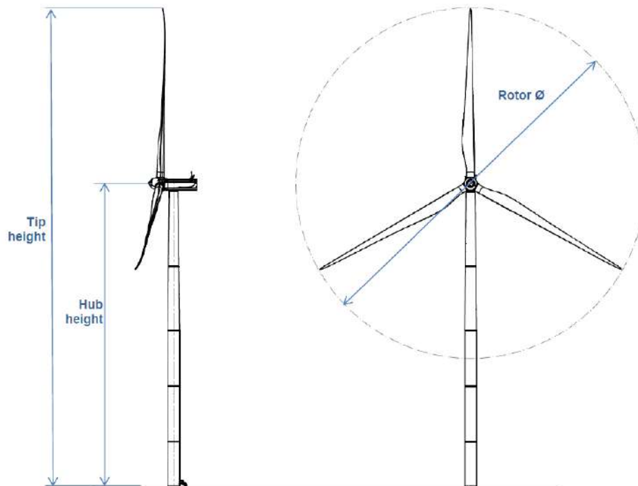
Figura 4-24: Struttura aerogeneratore
