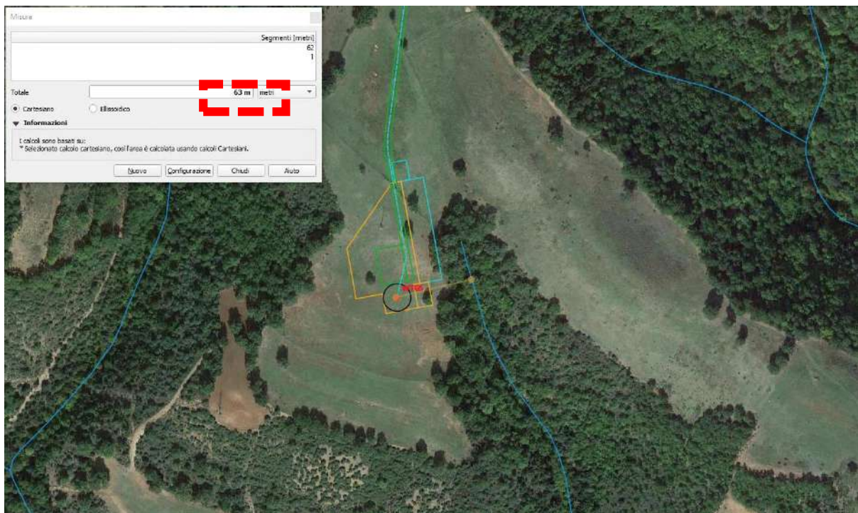
Figura 4-74: Distanza tra l'asse della turbina WTG 05 e l'alveo del corso d'acqua superficiale
