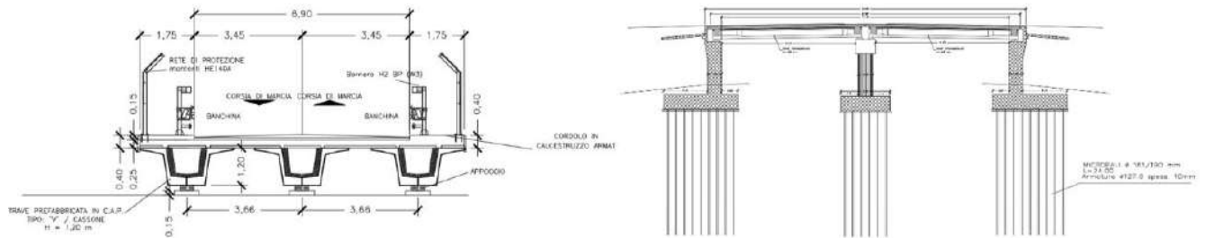
Figura 4-36: Sezioni Tipo Ponte 2
