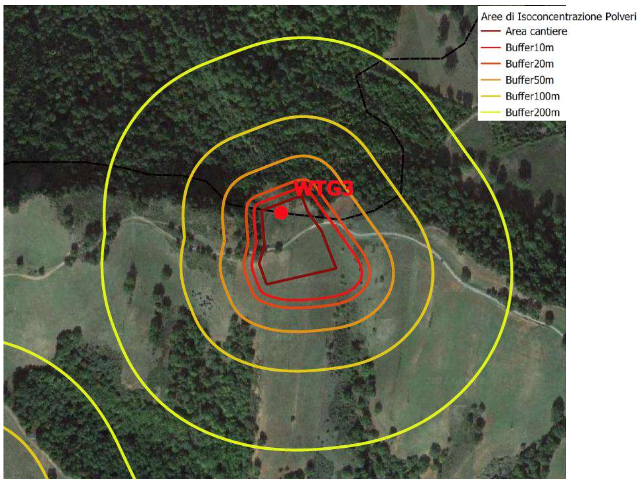
Figura 4-62: Aree Isoconcentriche nell'area di cantiere della turbina WTG03
