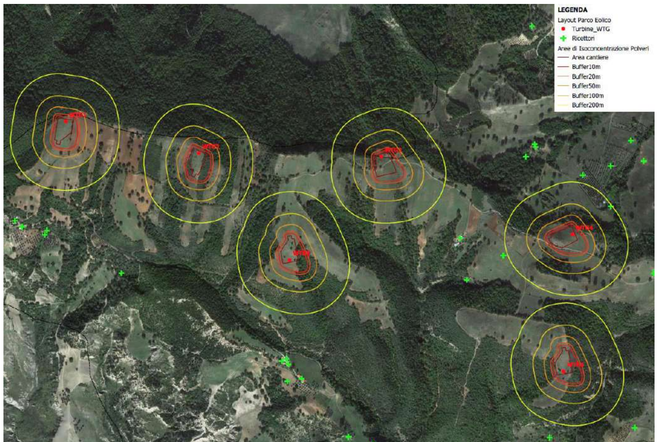
Figura 4-81: Aree di Isoconcentrazione e Ricettori - Layout Impianto
