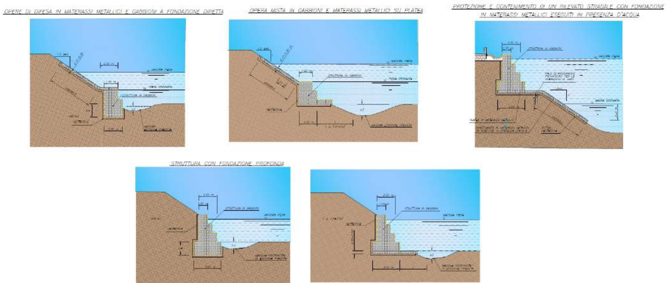
Figura 4-34: Sezioni Tipo interventi di inserimento paesaggistico
