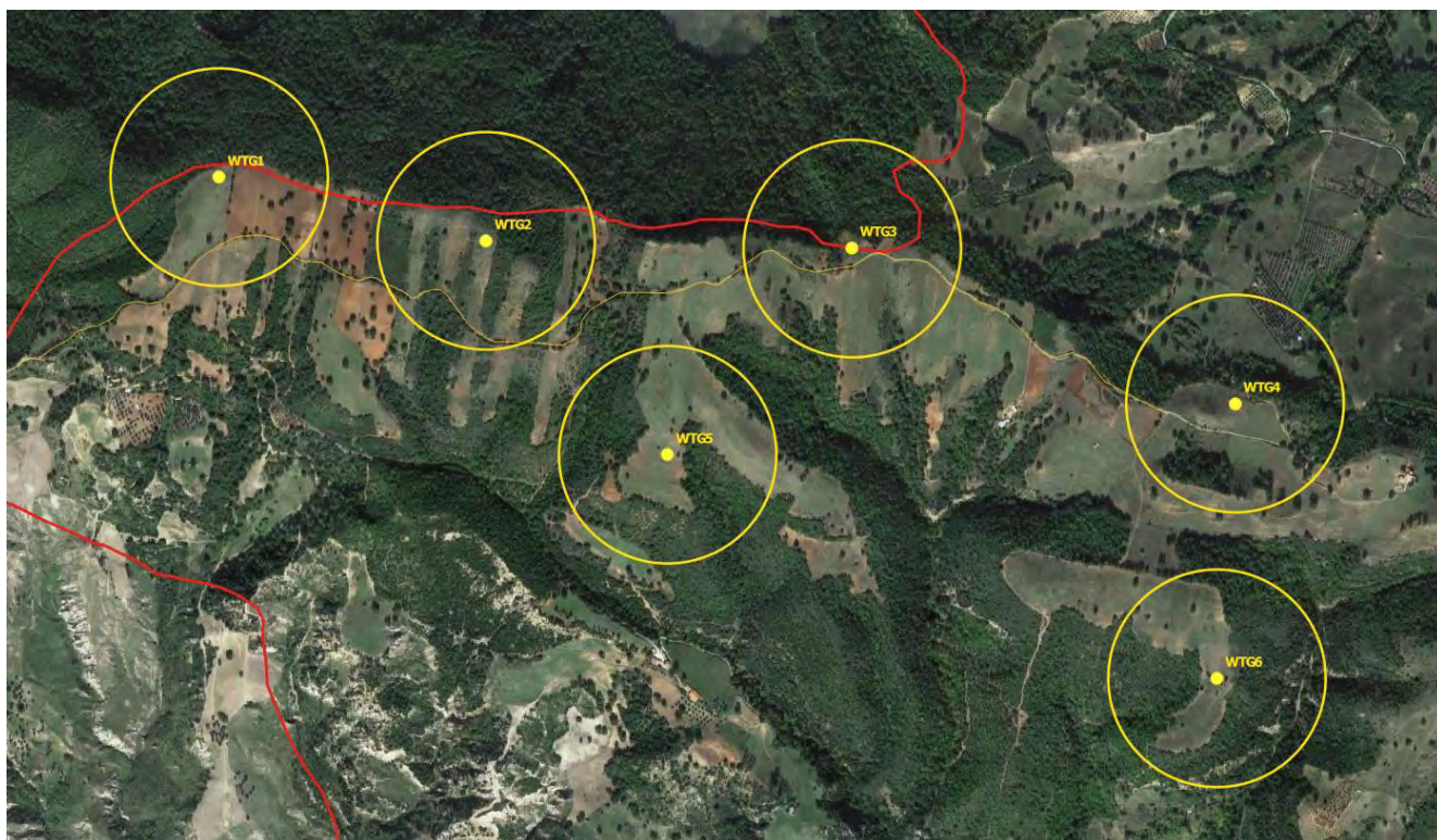
Figura 1 – Indicazione della gittata massima della pala in caso di distacco
