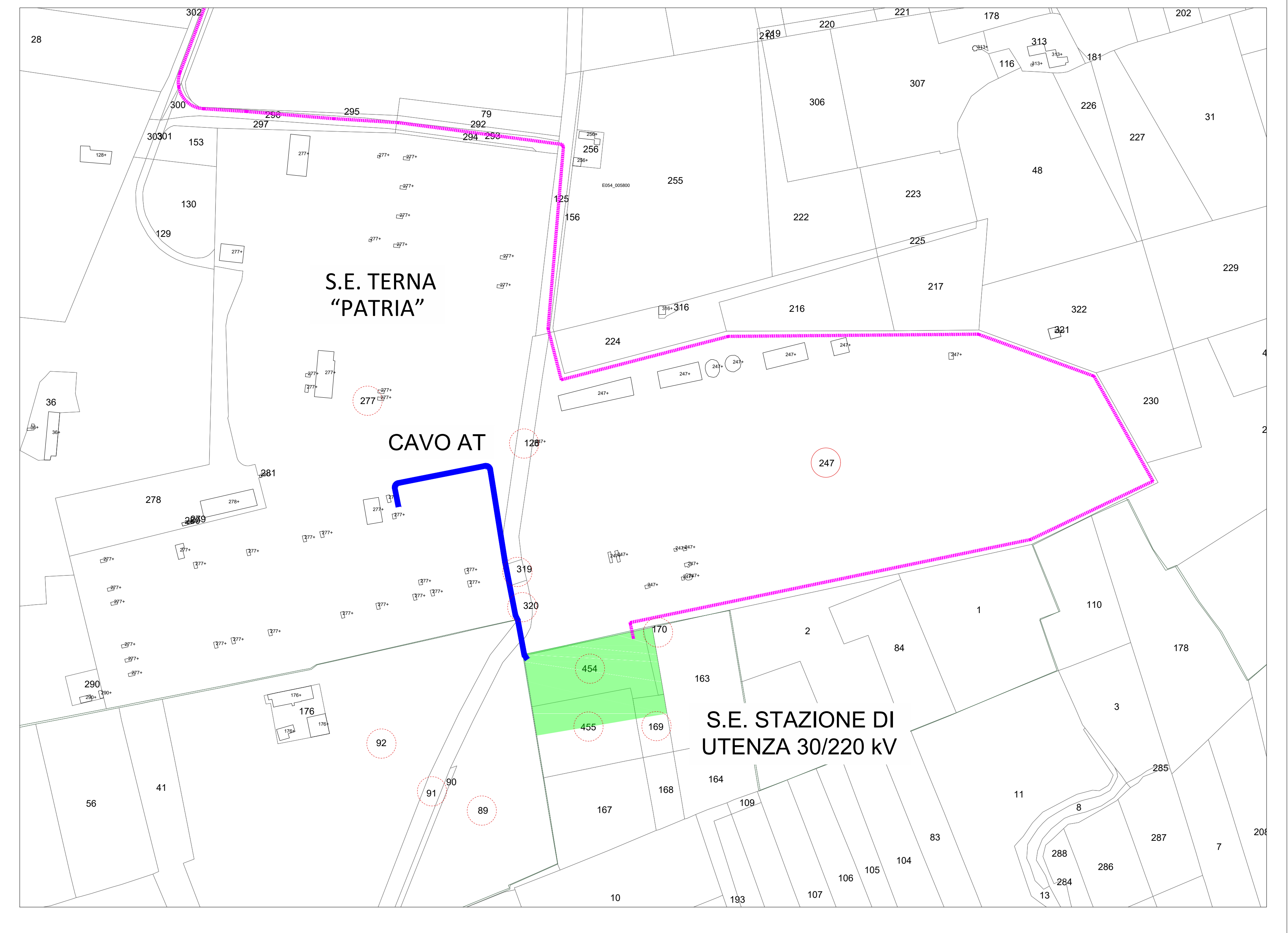
CATASTALE OPERE DI CONNESSIONE ALLA RETE - Scala 1:2000
