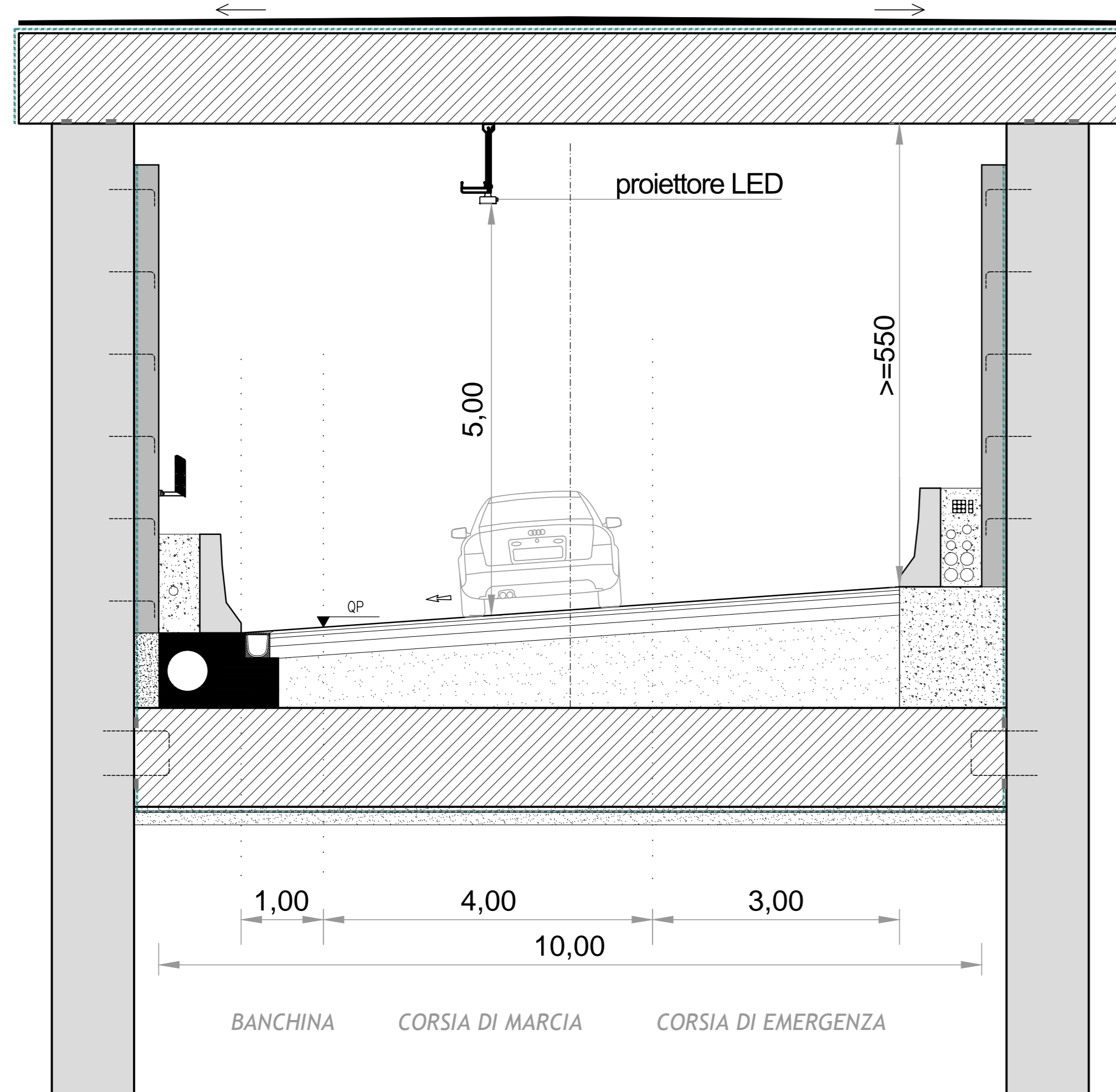
SEZIONE A - GALLERIA IGA_01 - scala 1:50
