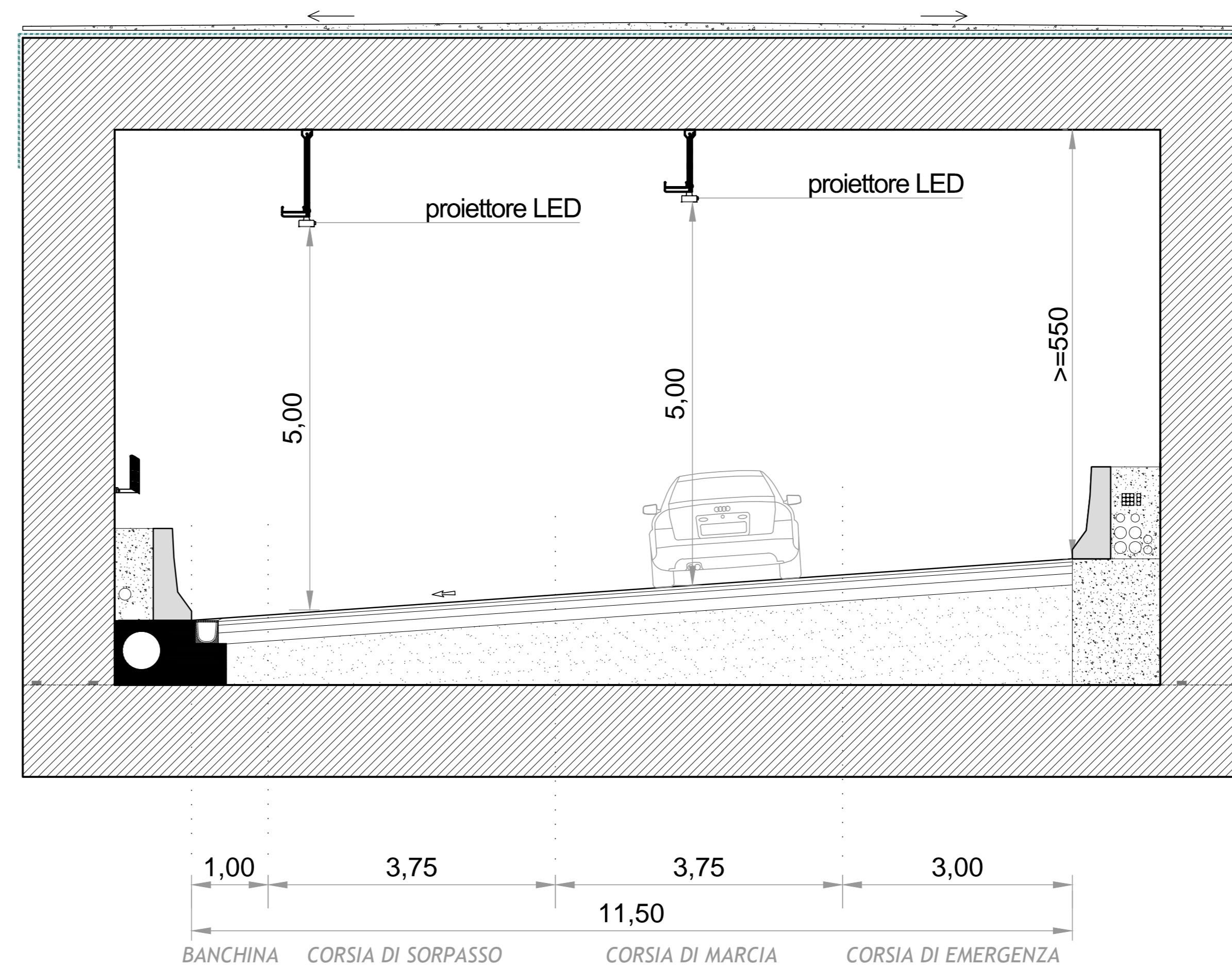
SEZIONE B - GALLERIA IGA_02 - scala 1:50
