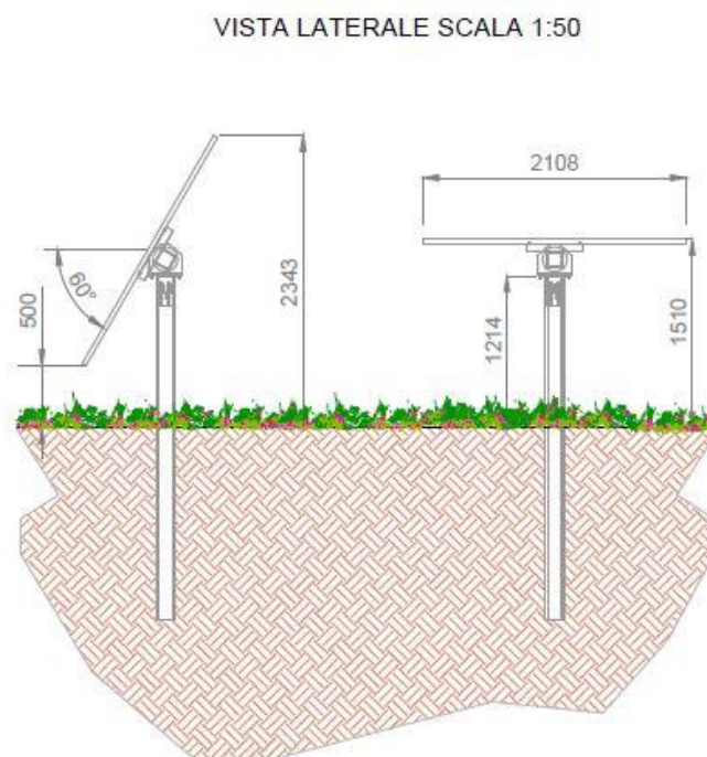
Fig.2. Schema della struttura – sezione
