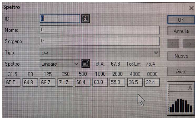
Figura 3: Livelli di potenza sonora trasformatori AT/MT
