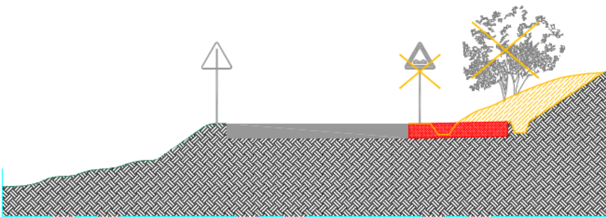
ALLARGAMENTO TIPO SEDE STRADALE LATO MONTE
