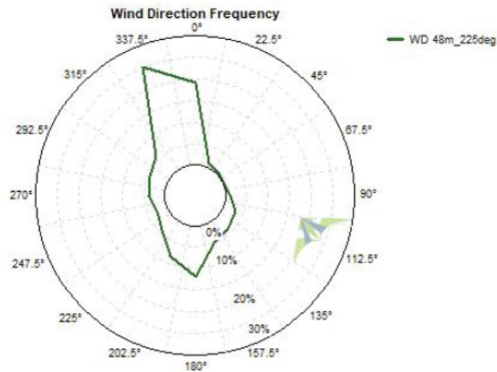
Figura 3-3: Direzione prevalente vento alla stazione anemometrica
