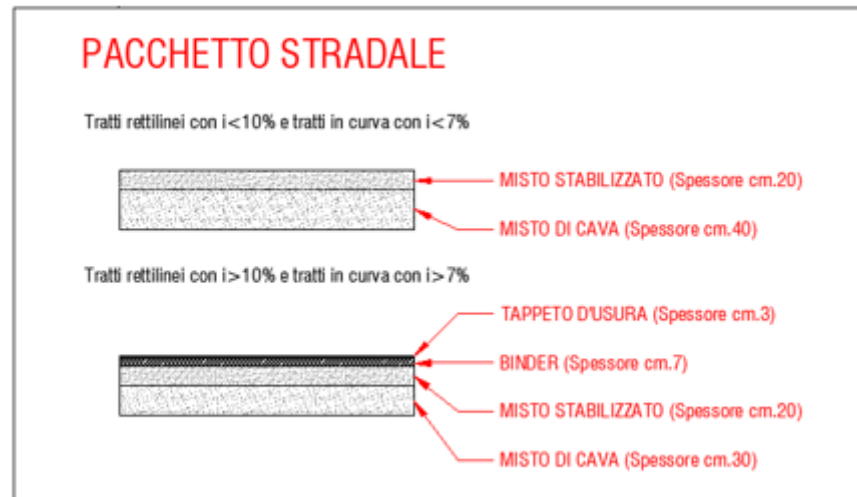
Figura 3-2: Pacchetti stradali
