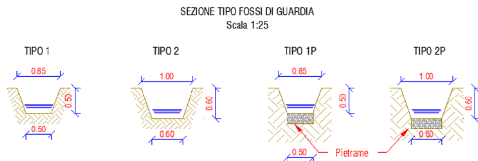
Figura 5-1. Estratto da tavola di progetto – Fossi di guardia
