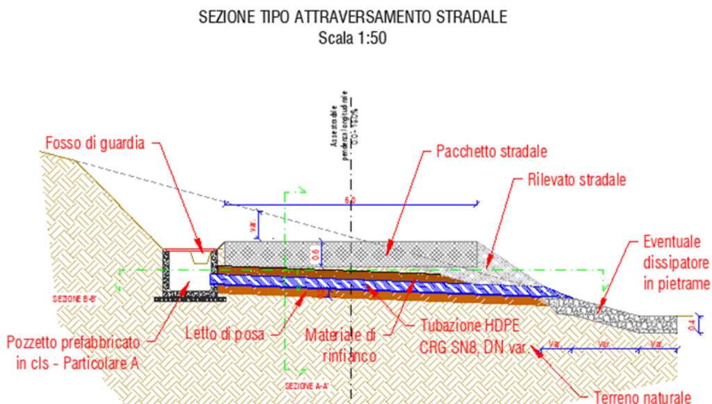
Figura 5-3. Estratto da tavola di progetto - Attraversamento stradale di scarico
