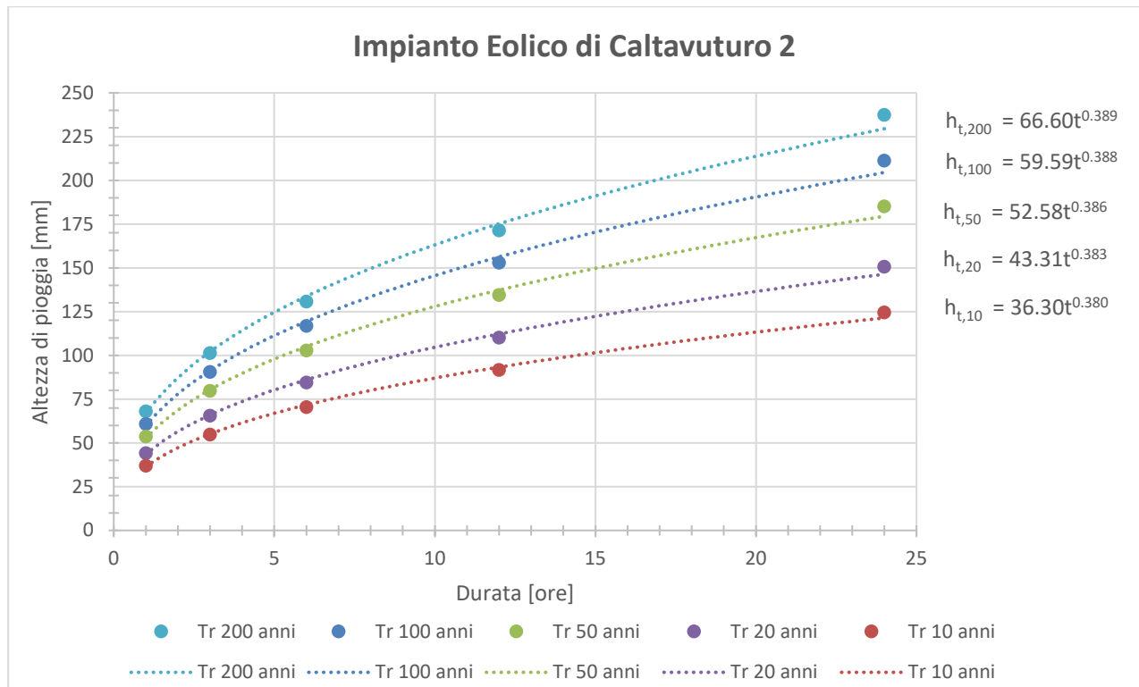
Figura 3-1: curve di possibilità pluviometrica
