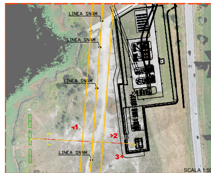
RILIEVO PLANOALTIMETRICO POST-INTERVENTO
