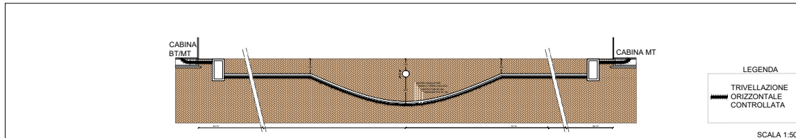
SEZIONE BB' METANODOTTO SNAM
