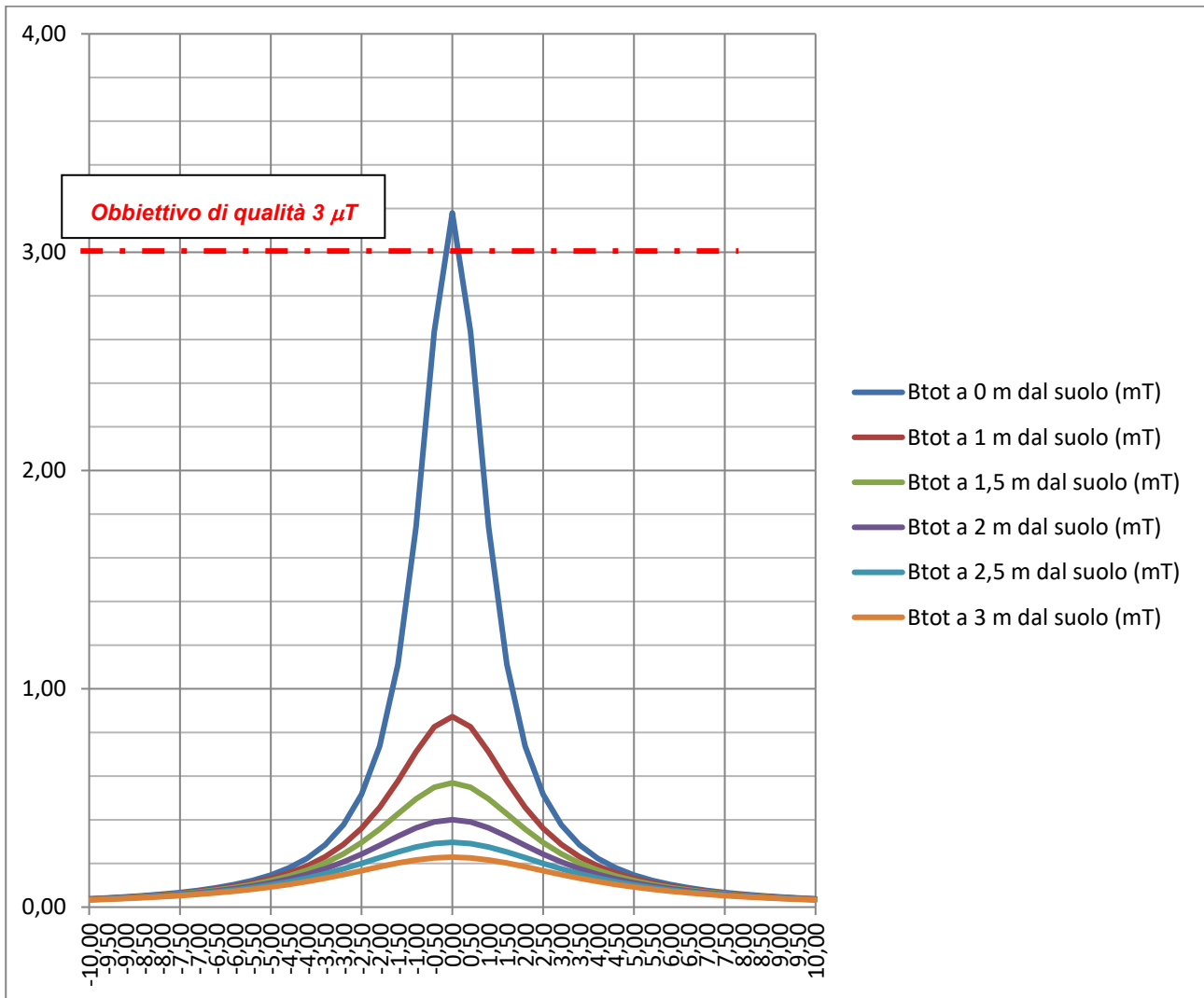
Grafico del campo di induzione magnetica per diverse distanze dall'asse dei cavidotti e altezze dal suolo
