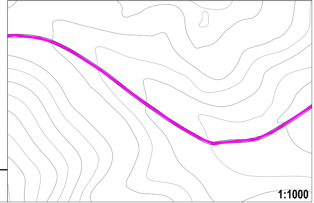
Particolare cavidotto MT - DPA 2,00 m
