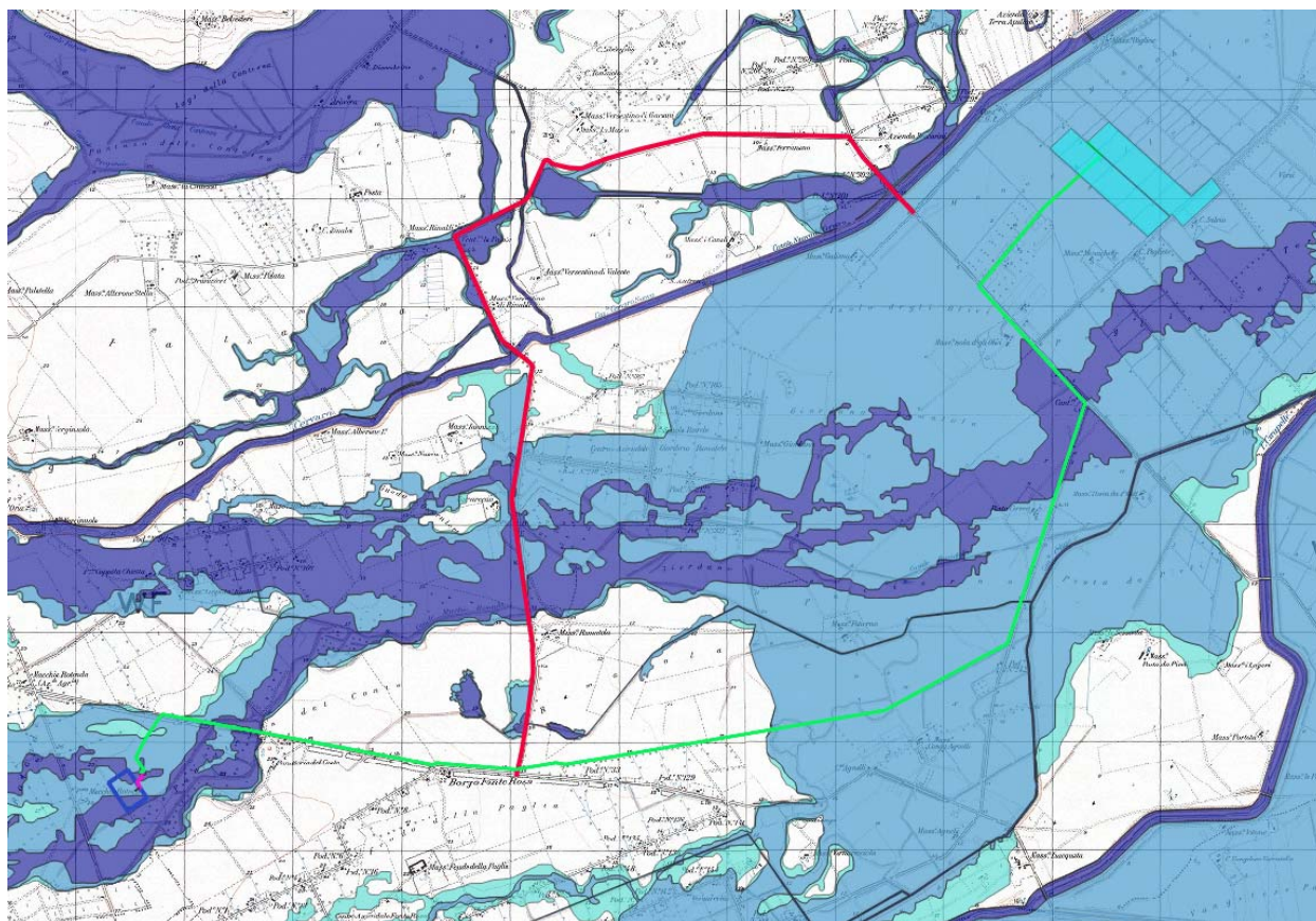
Figura 1 – Soluzione alternativa – Doppio Attraversamento Fiume Cervaro
