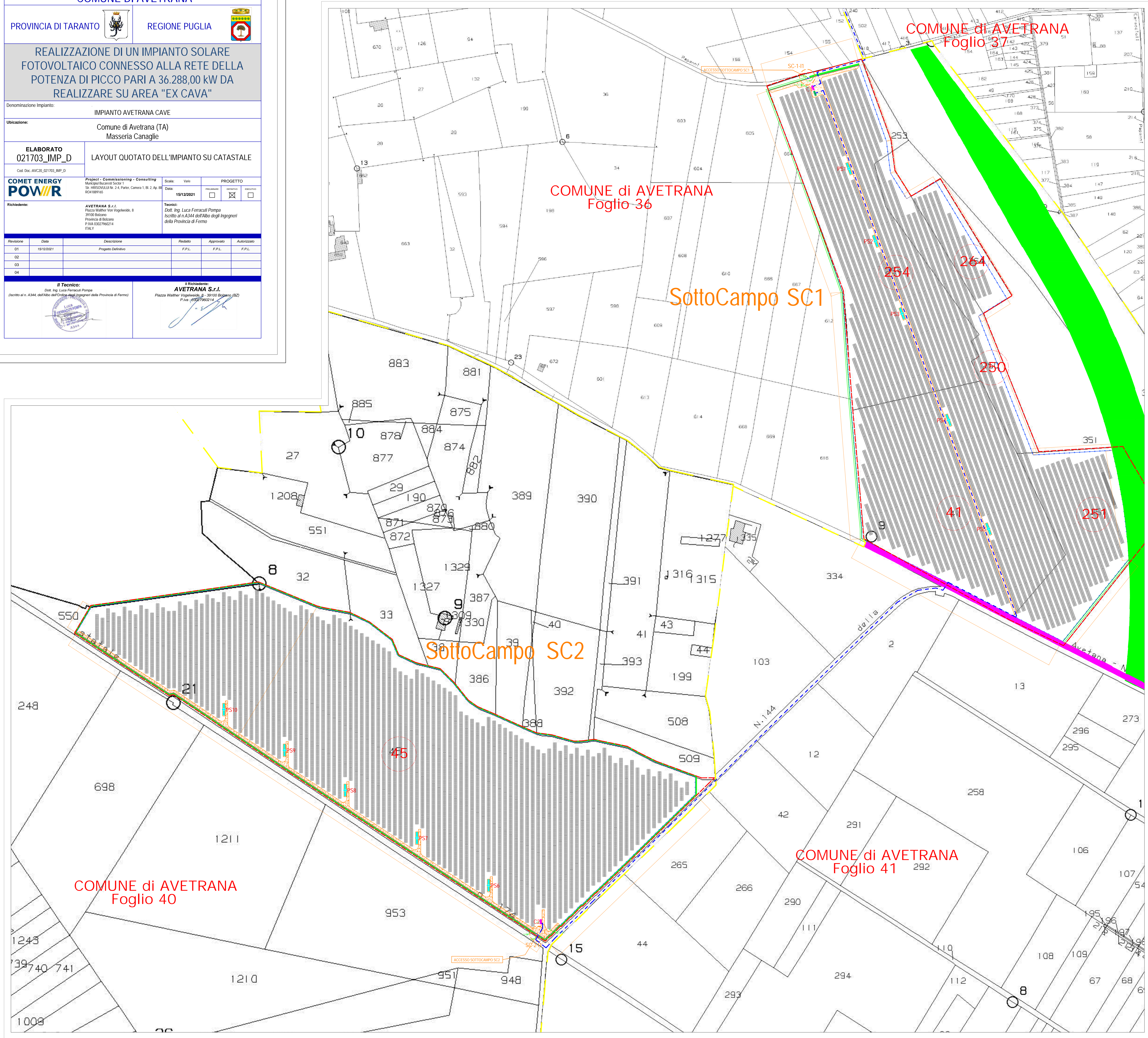
PARTICOLARE IMPIANTI SCALA DI RIPRODUZIONE 1:2.000
