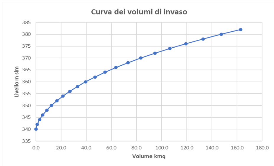
Fig. 3.2a - Diagramma Volumi dell'Invaso - aggiornamento 2006
