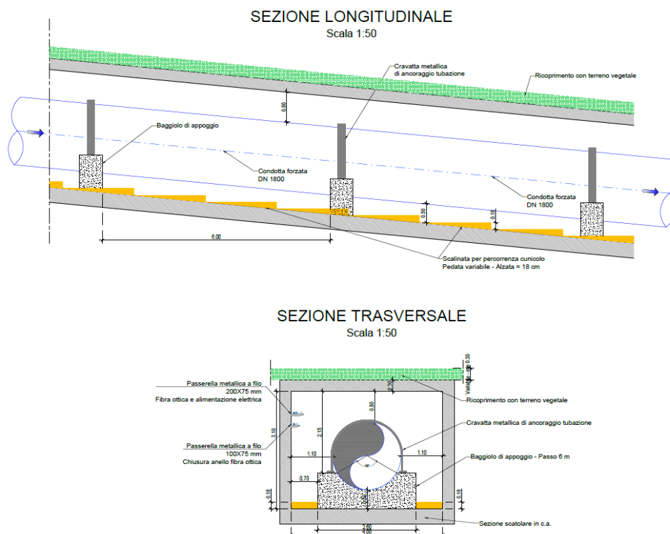
Fig. 5.15 - Cunicolo condotta forzata - Sezioni
