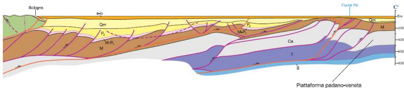
FIGURA 3-2: SEZIONE GEOLOGICA PASSANTE PER IL TRATTO PIÙ ORIENTALE DELLA PORZIONE DI PIANURA IN ESAME (STRALCIO DA AA. VV., 2004, "CARTA SISMOTETTONICA DELLA REGIONE EMILIA-ROMAGNA")
