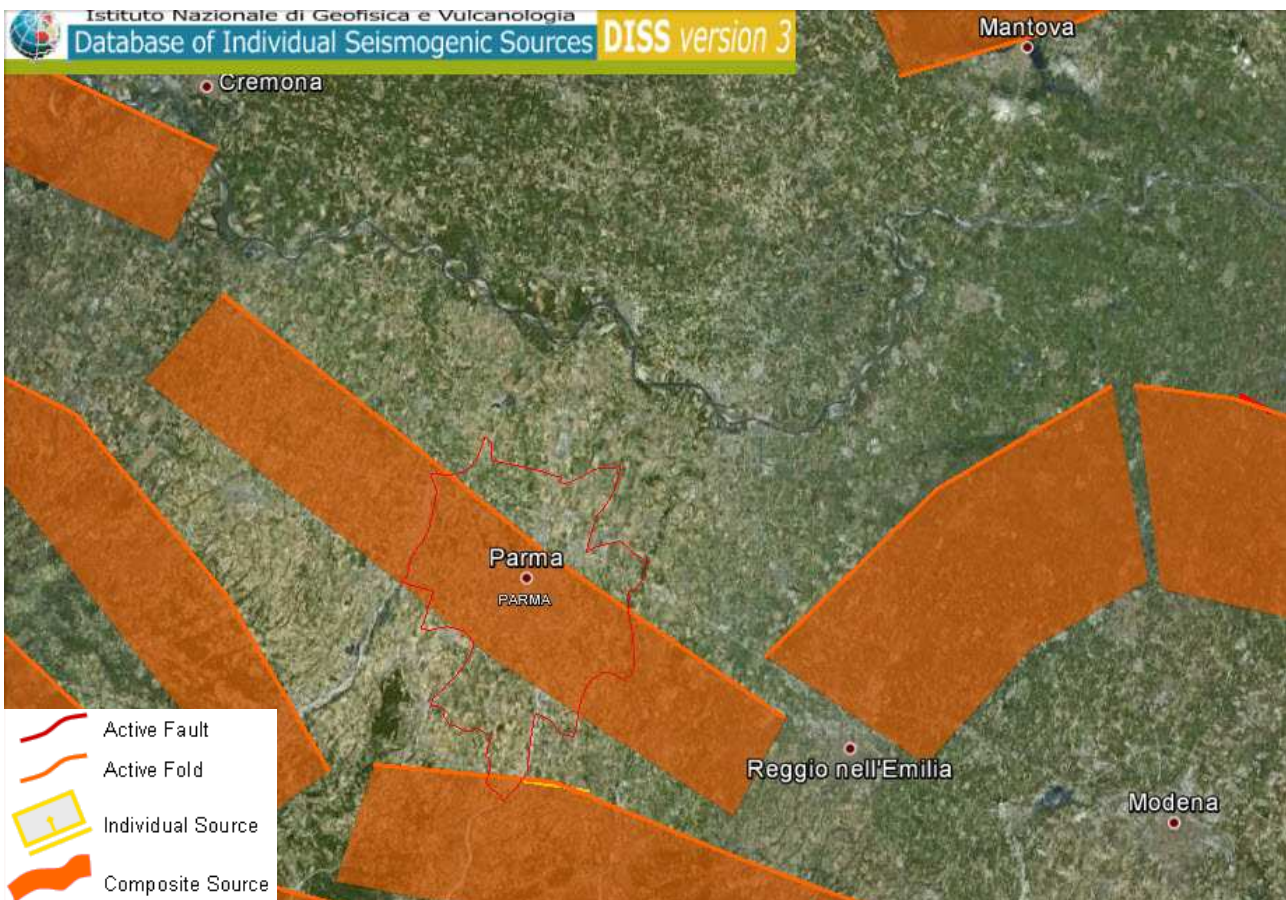
FIGURA 6-1: SORGENTI SISMOGENETICHE CONTENUTE NELLA NUOVA VERSIONE DEL "DATABASE OF POTENTIAL SOURCES FOR EARTHQUAKES LARGER THAN M 5.5 IN ITALY" PER L'AREA IN OGGETTO
