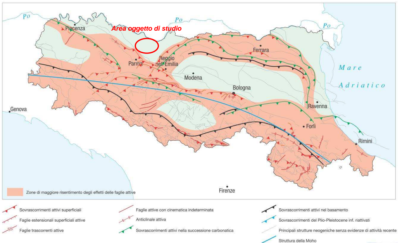
FIGURA 3-3: ZONE DI MAGGIOR RISENTIMENTO DELLE FAGLIE ATTIVE
