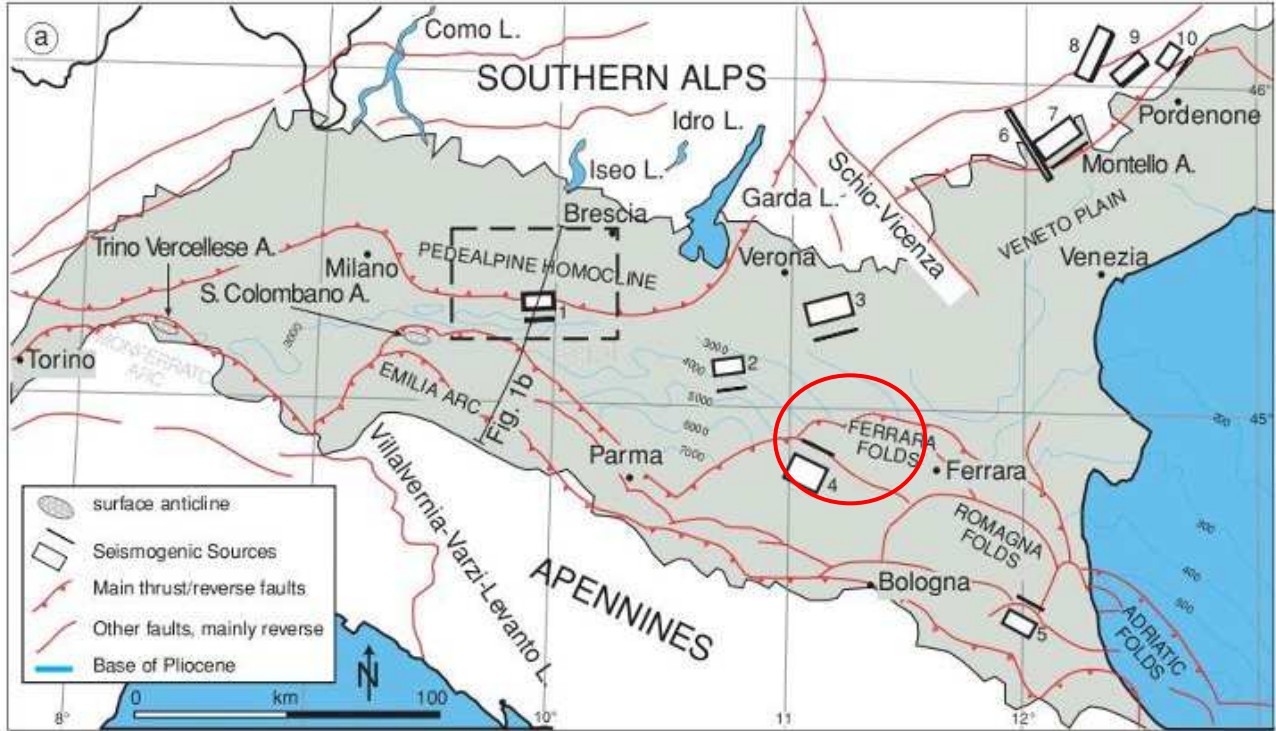
FIGURA 11-2. SCHEMA STRUTTURALE DELLA CATENA SEPOLTA (IN ROSSO L'AREA COLPITA DAL SISMA).
