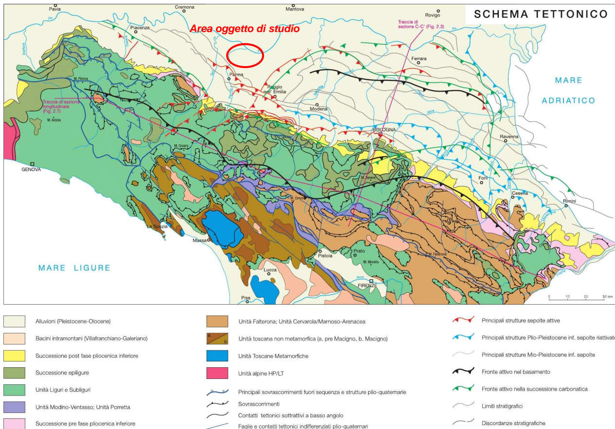
FIGURA 3-1: AREA DI STUDIO CON LE PRINCIPALI STRUTTURE SEPOLTE DELL'APPENNINO SETTENTRIONALE (DA PIERI & GROPPI, 1981, MODIFICATA)
