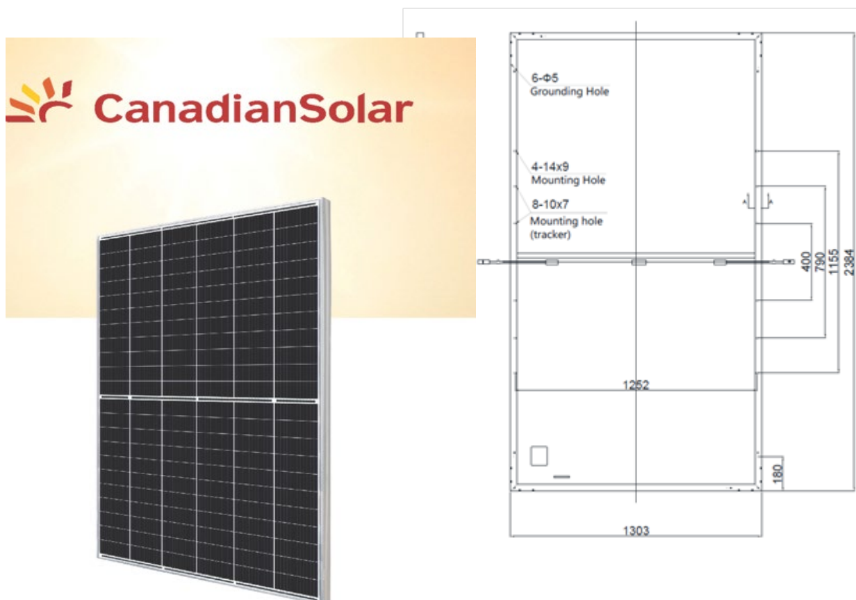
Figura 9 – Modulo fotovoltaico
