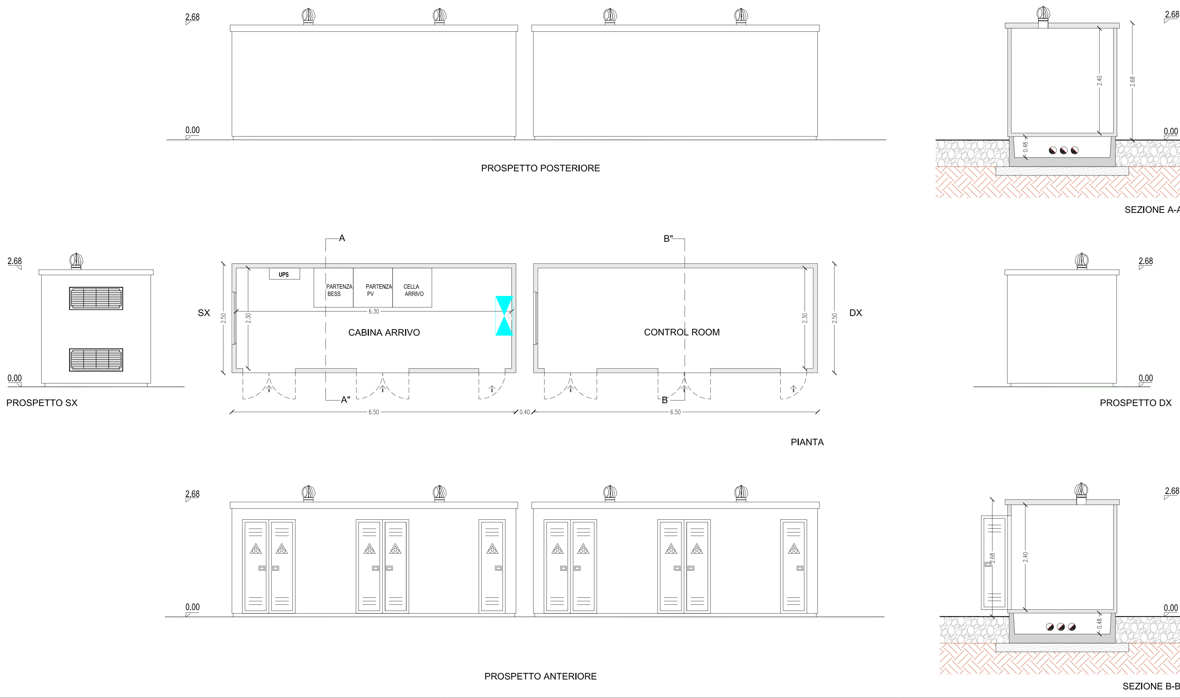
PIANTA PROSPETTI E SEZIONE CABINA ARRIVO - CONTROL ROOM Scala 1:50
