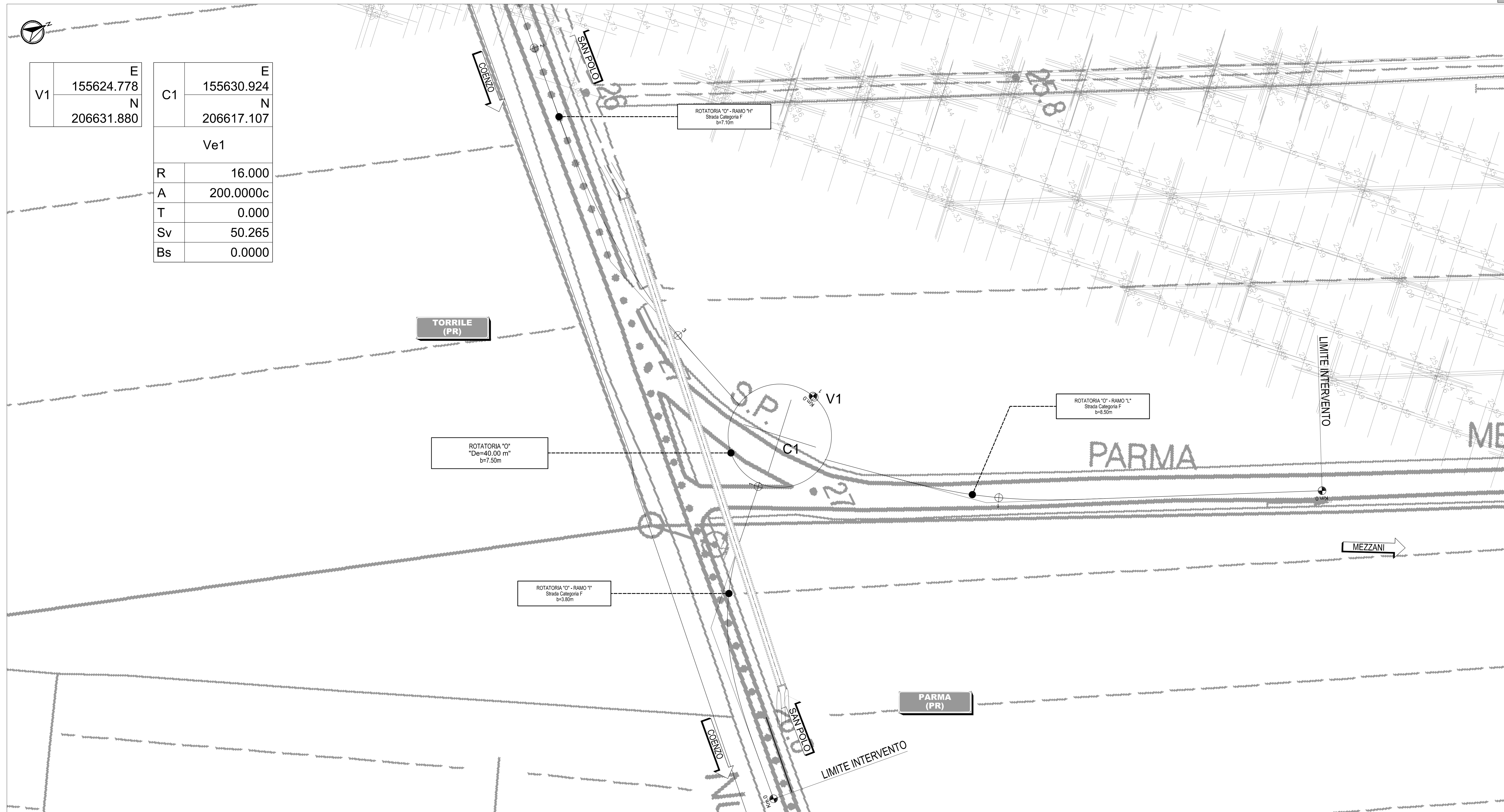
TRAIETTORIE DI DEFLESSIONE - Scala: 1:500 - ROTATORIA O
