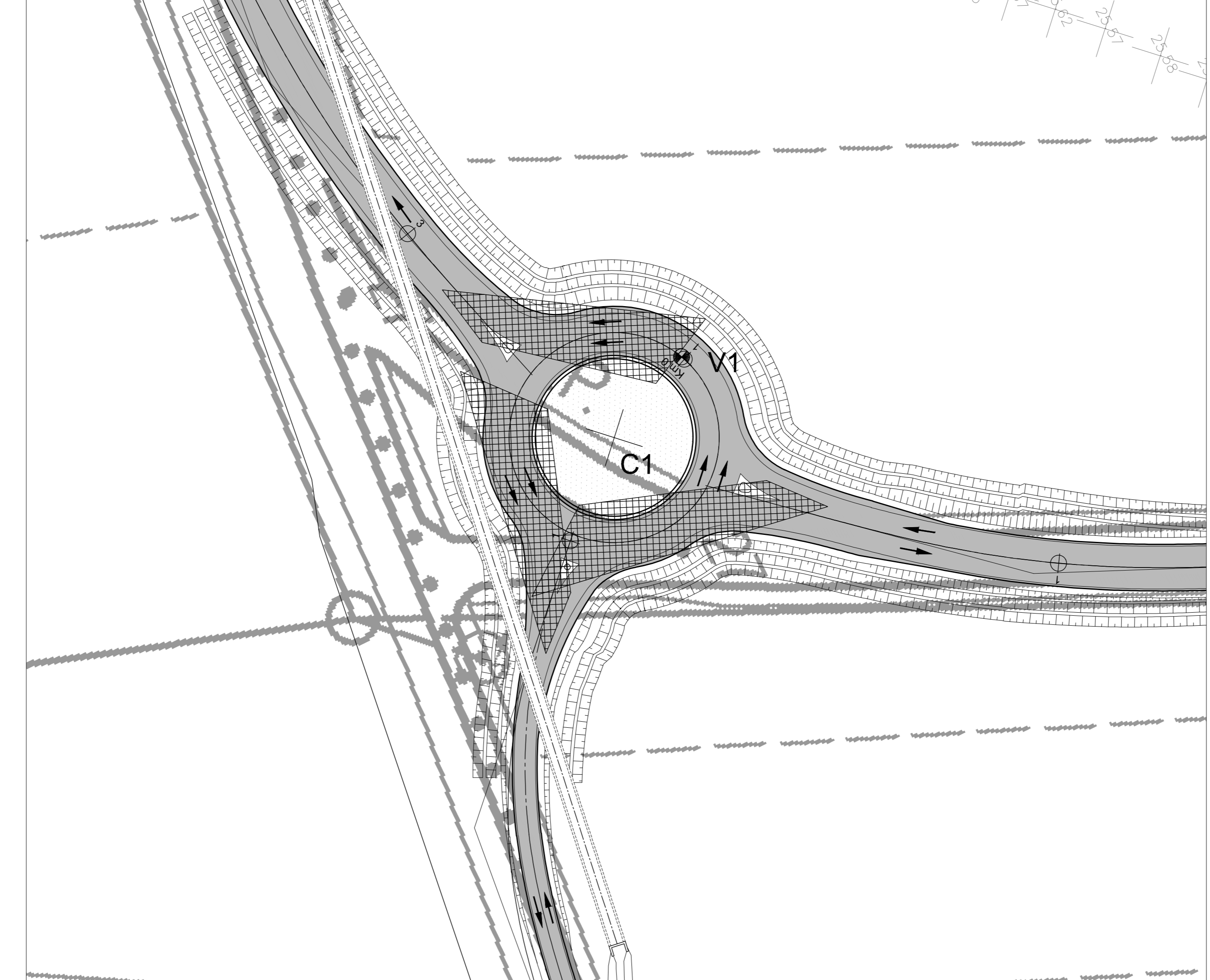
TRIANGOLI DI VISIBILITA' - Scala: 1:500 - ROTATORIA O
