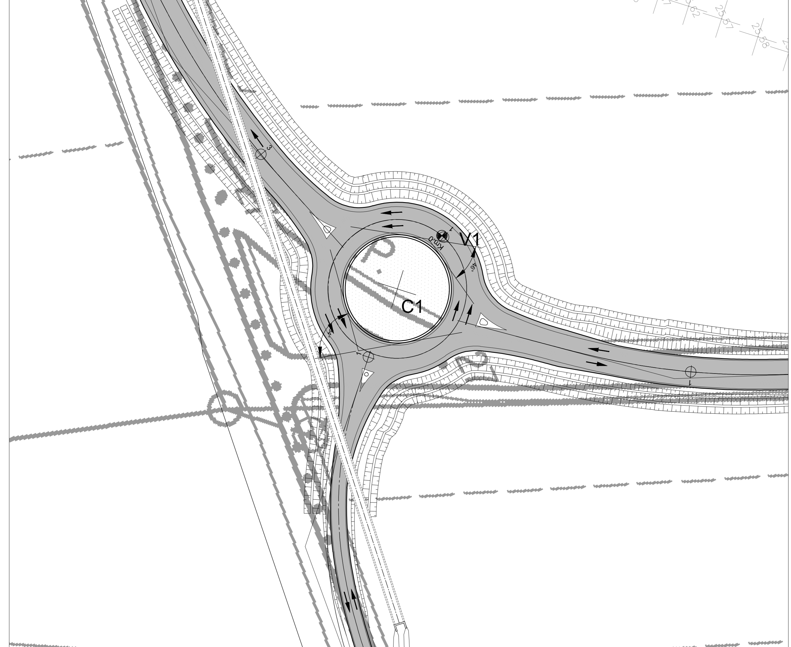
TRAIETTORIE DI DEFLESSIONE - Scala: 1:500 - ROTATORIA O
