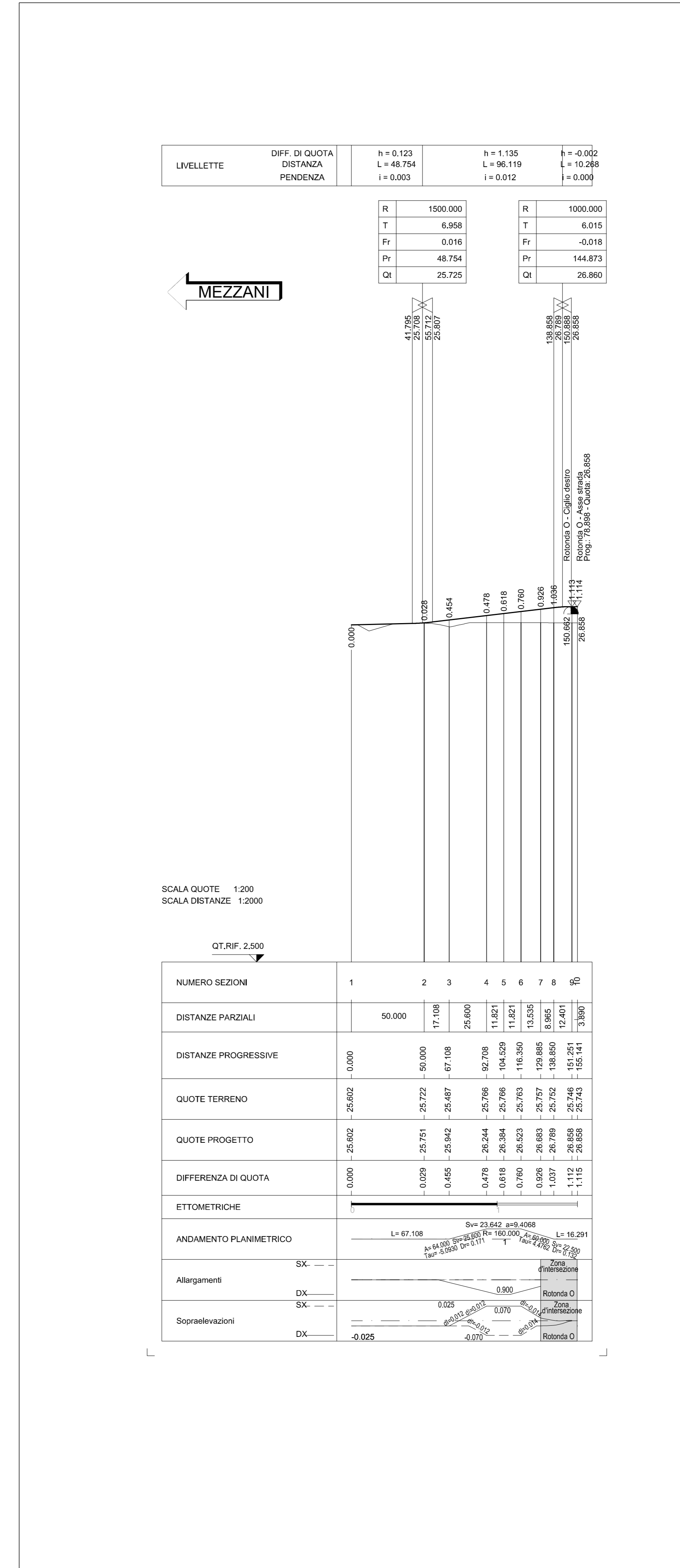
PROFILO LONGITUDINALE - Scala: 1:2.000/200 ASSE L
