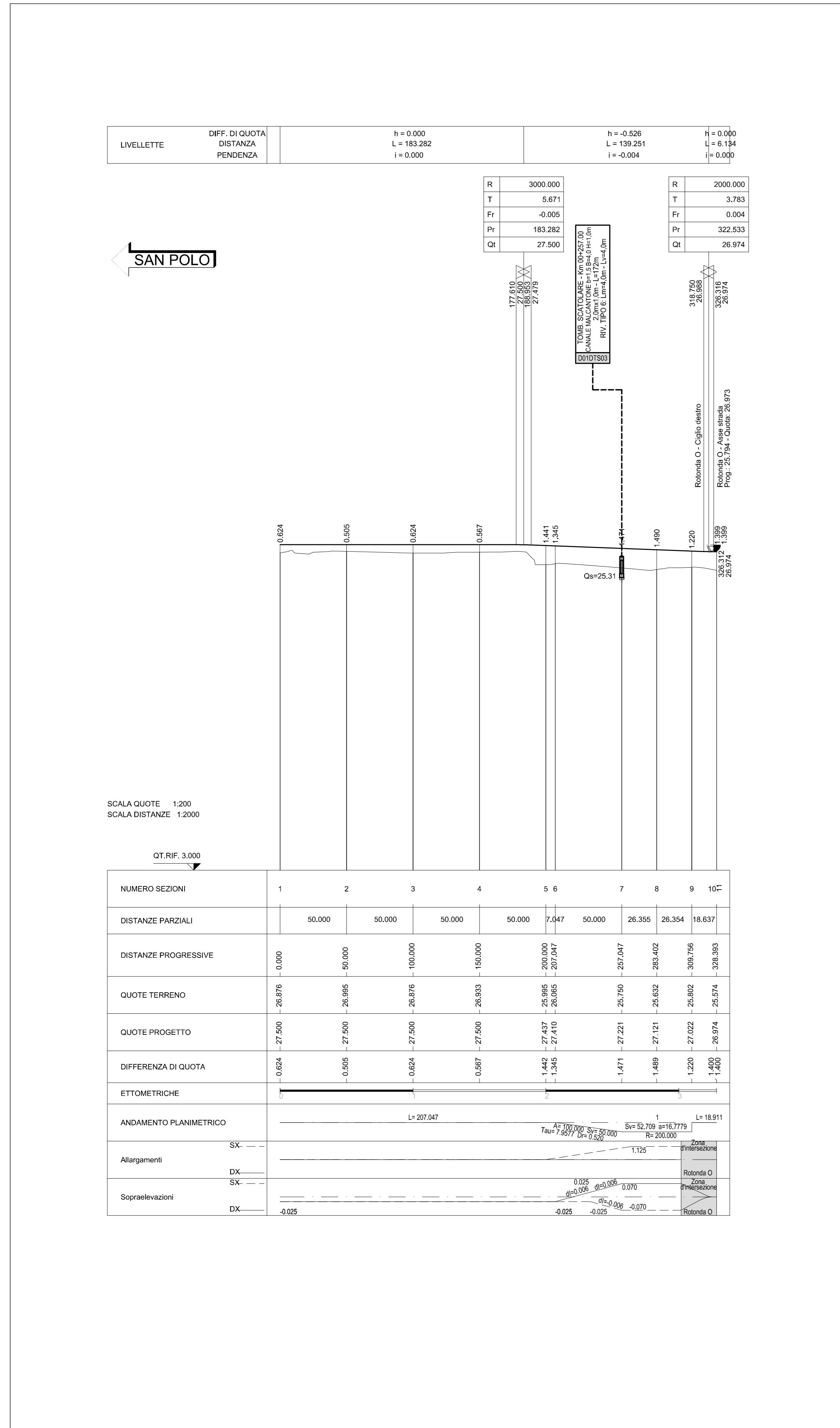
PROFILO LONGITUDINALE - Scala: 1:2.000/200 ASSE H
