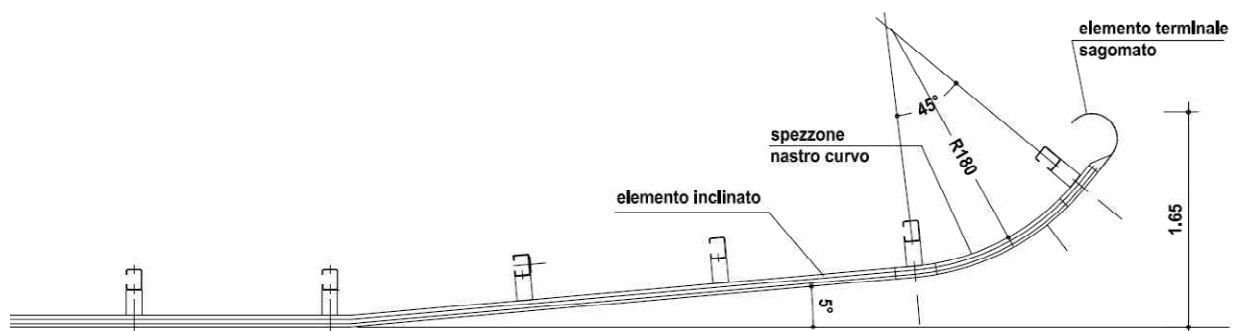
figura 7.1: schema di blocco terminale di avvio
