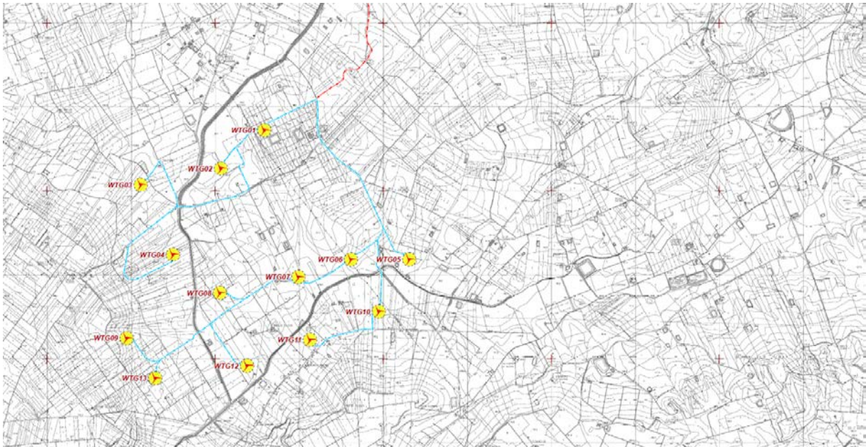
Figura 1: Inquadramento dell'area di realizzazione dell'impianto di 13 aerogeneratori per una potenza complessiva di 72.80 MW in agro del Comune di Mazara del Vallo (TP) - stralcio dell'elaborato grafico "Corografia generale"
