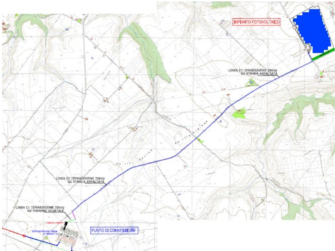
Figura 5 – Planimetria generale dell’impianto
