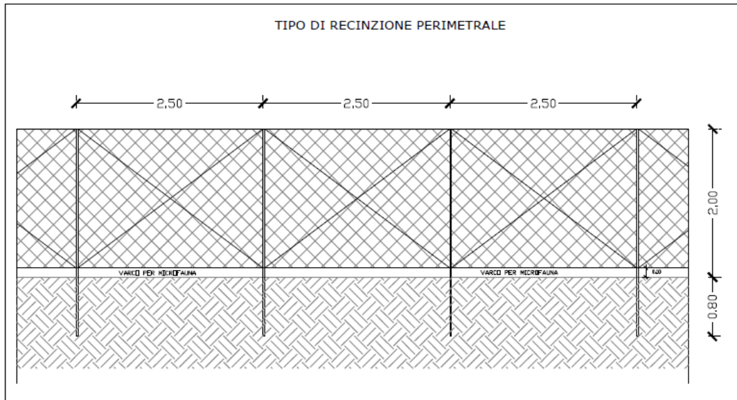
Figura 21 - Recinzione tipo dell'area del campo fotovoltaico
