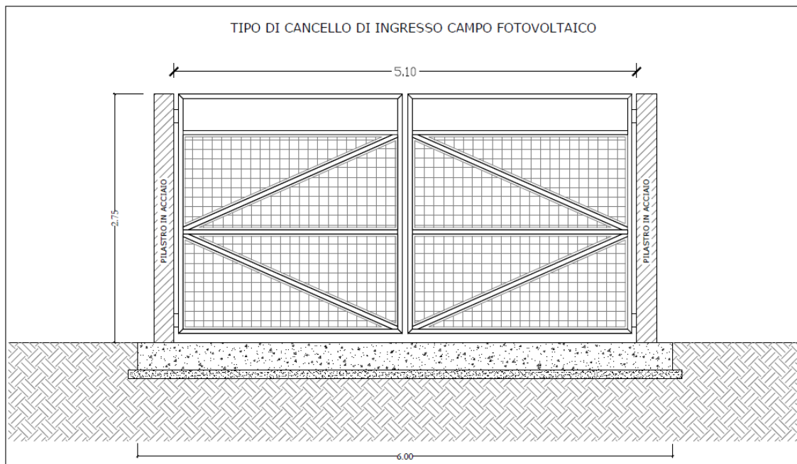
Figura 22 - Cannello di ingresso al campo fotovoltaico
