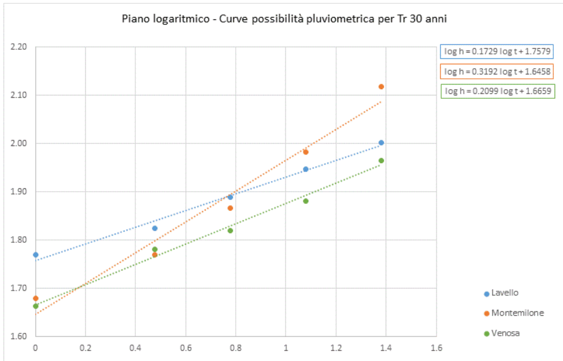
Figura 10 – Curve di possibilità pluviometrica trentennali per le stazioni di Lavello, Montemilone e Venosa su piano logaritmico
