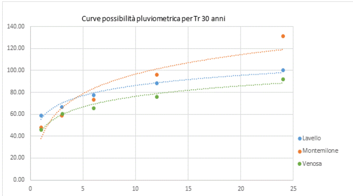
Figura 9 – Curve di possibilità pluviometrica trentennali per le stazioni di Lavello, Montemilone e Venosa
